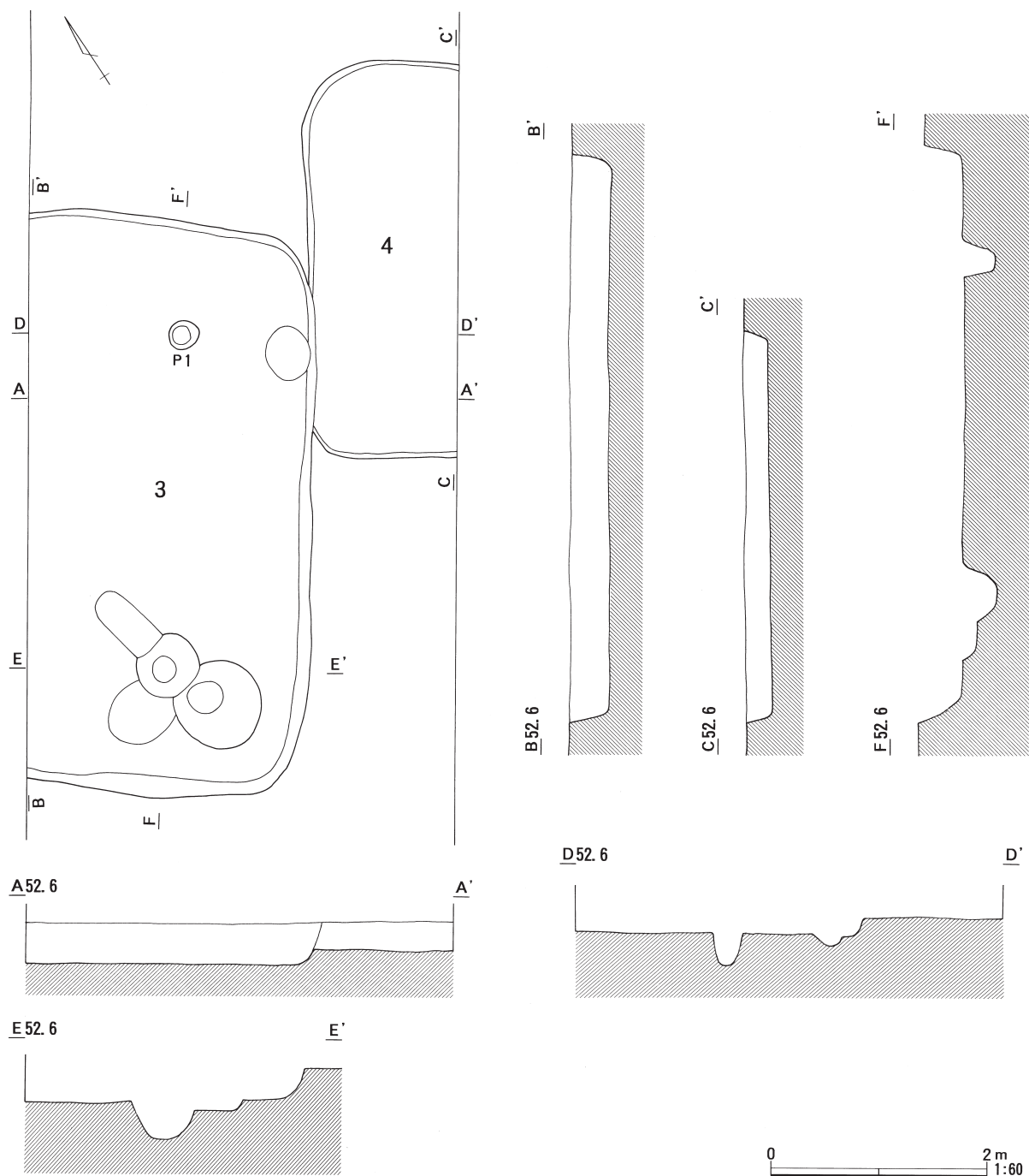
図9 石神境遺跡SI-3・4平面図および断面図
