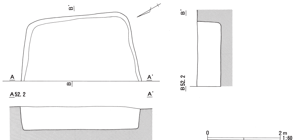
図42 石神境遺跡SI-20平面図および断面図
