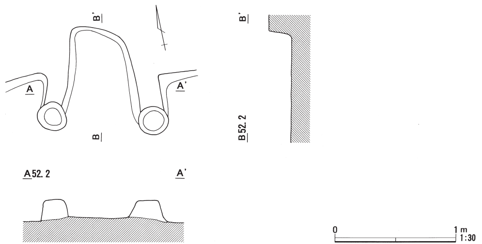
図31 石神境遺跡SI-14カマド平面図および断面図
