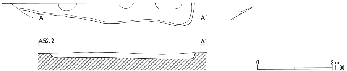
図35 石神境遺跡SI-16平面図および断面図
