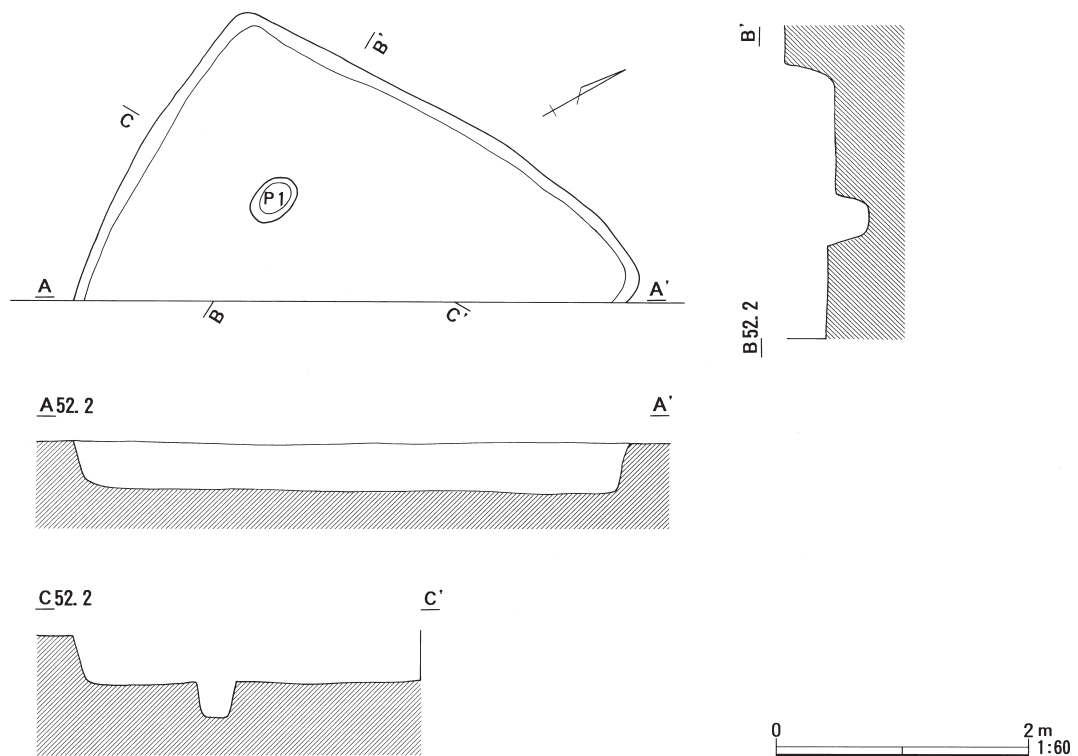
図24 石神境遺跡SI-10平面図および断面図
