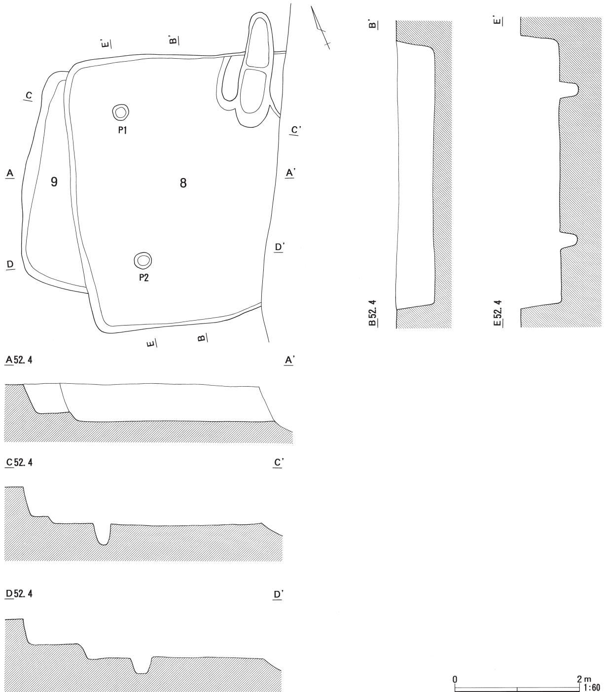
図20 石神境遺跡SI-8・9平面図および断面図
