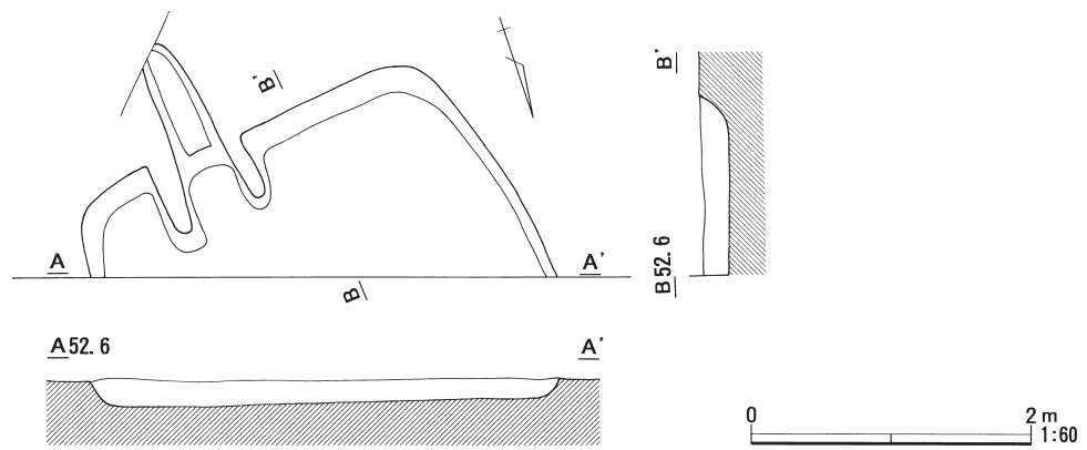
図12 石神境遺跡SI-5平面図および断面図
