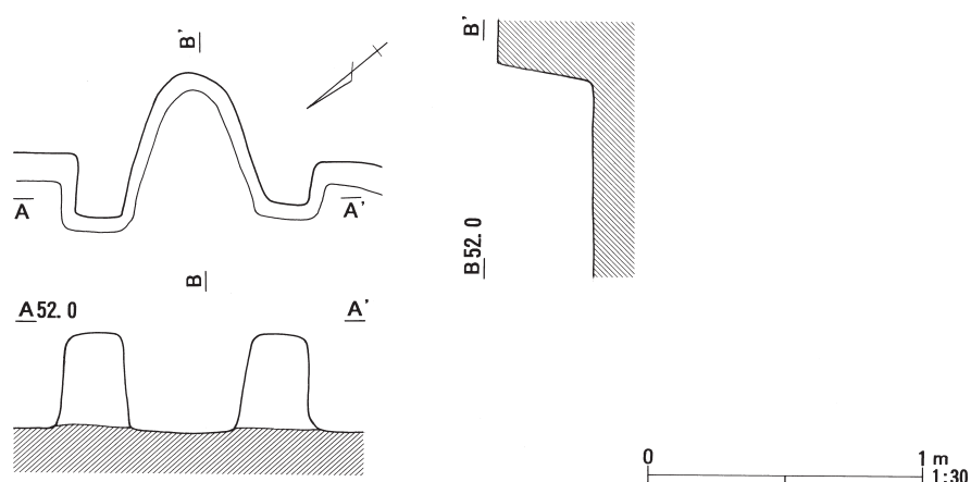
図41 石神境遺跡SI-19カマド平面図および断面図
