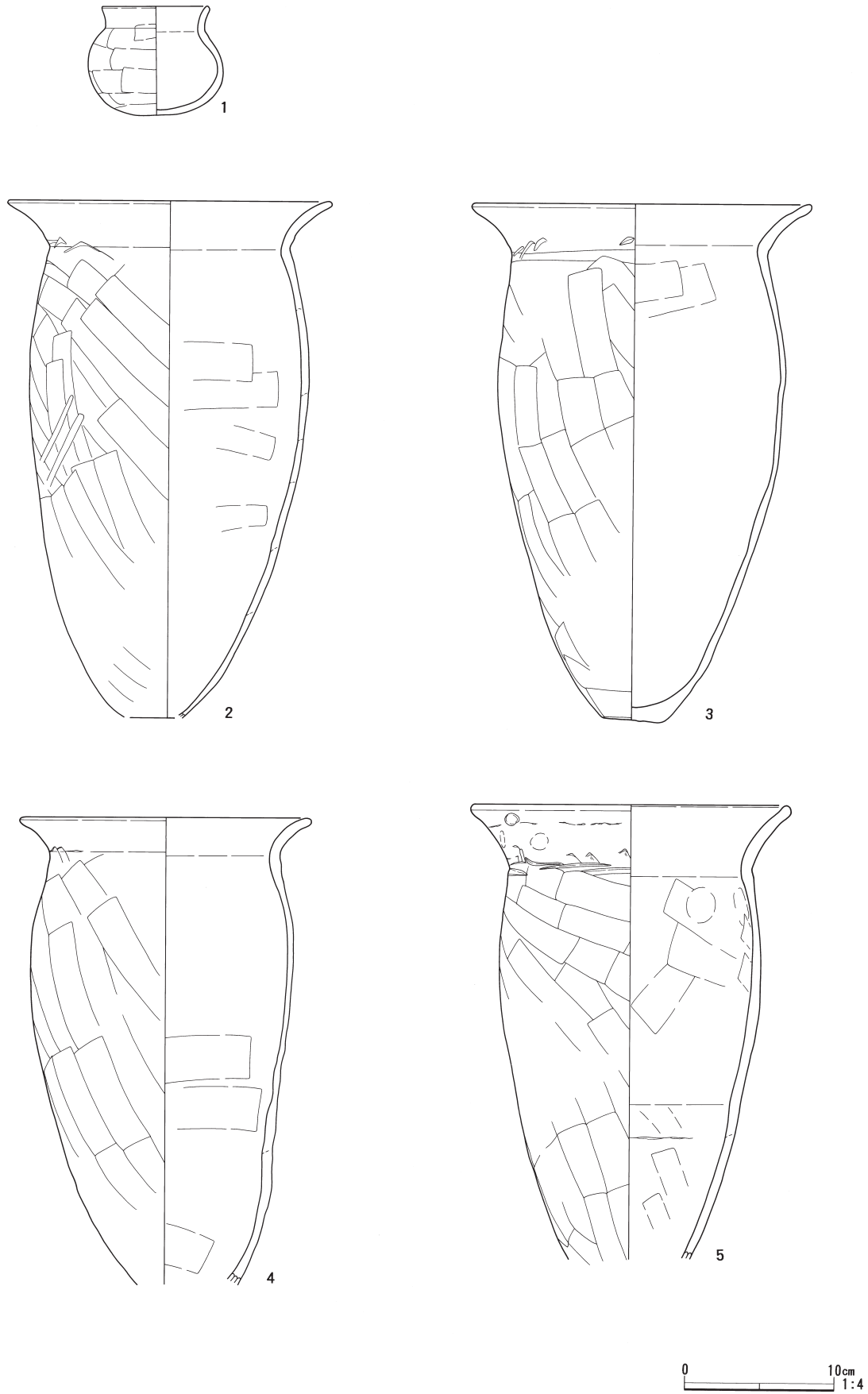
图7 石神境遺跡SI-2出土遺物（1）
