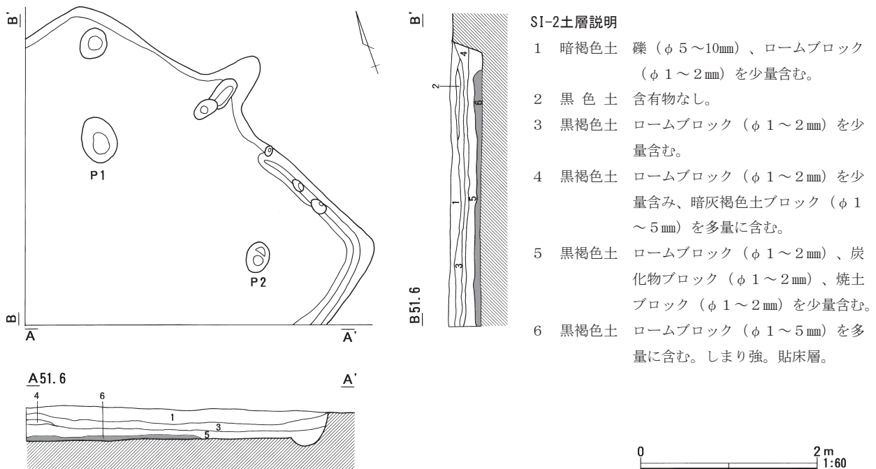
図76 天神林Ⅱ遺跡SI-2平面図および断面図
