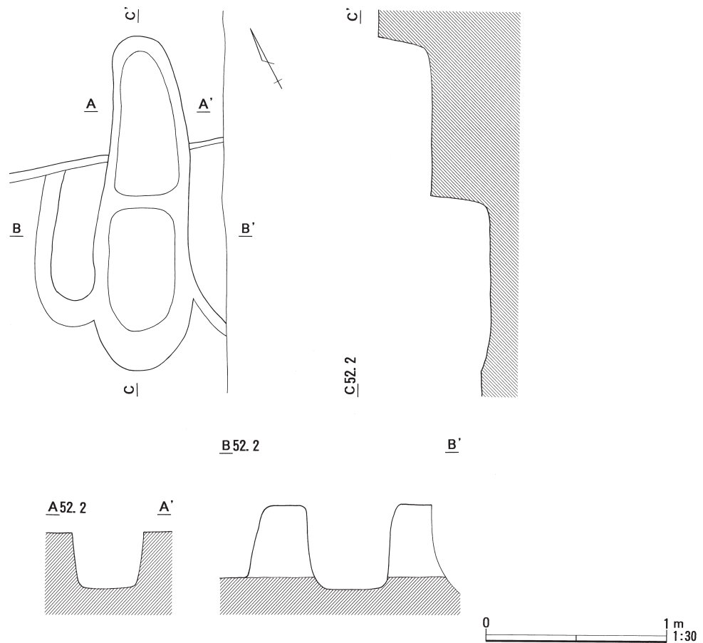
図21 石神境遺跡SI-8カマド平面図および断面図
