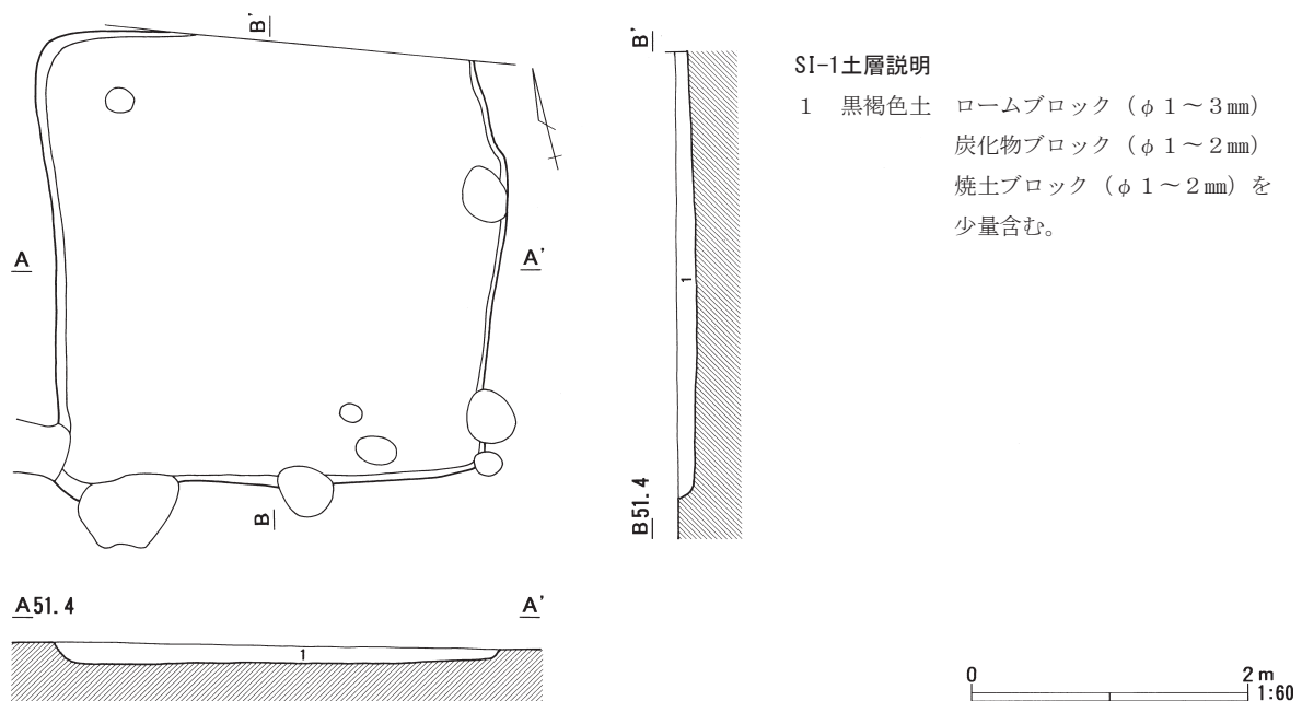
図75 天神林Ⅱ遺跡SI-1平面図および断面図
