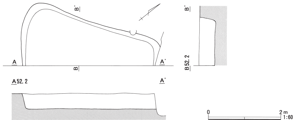
図44 石神境遺跡SI-21平面図および断面図
