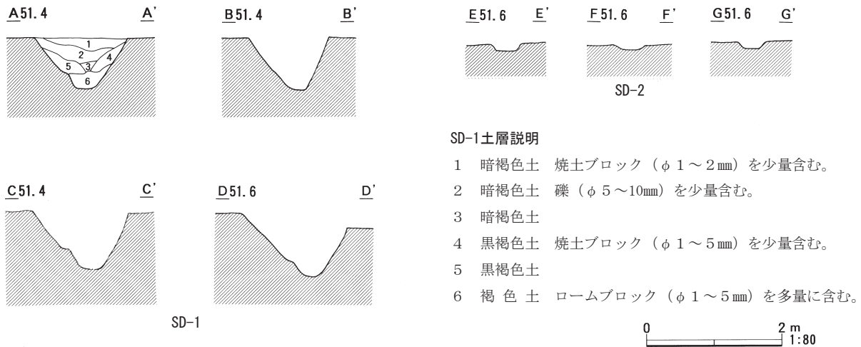
図78 天神林Ⅱ遺跡SD-1・2断面図
