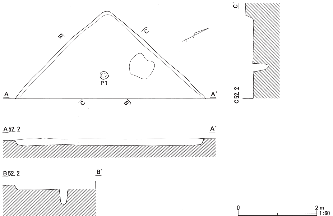
図27 石神境遺跡SI-12平面図および断面図
