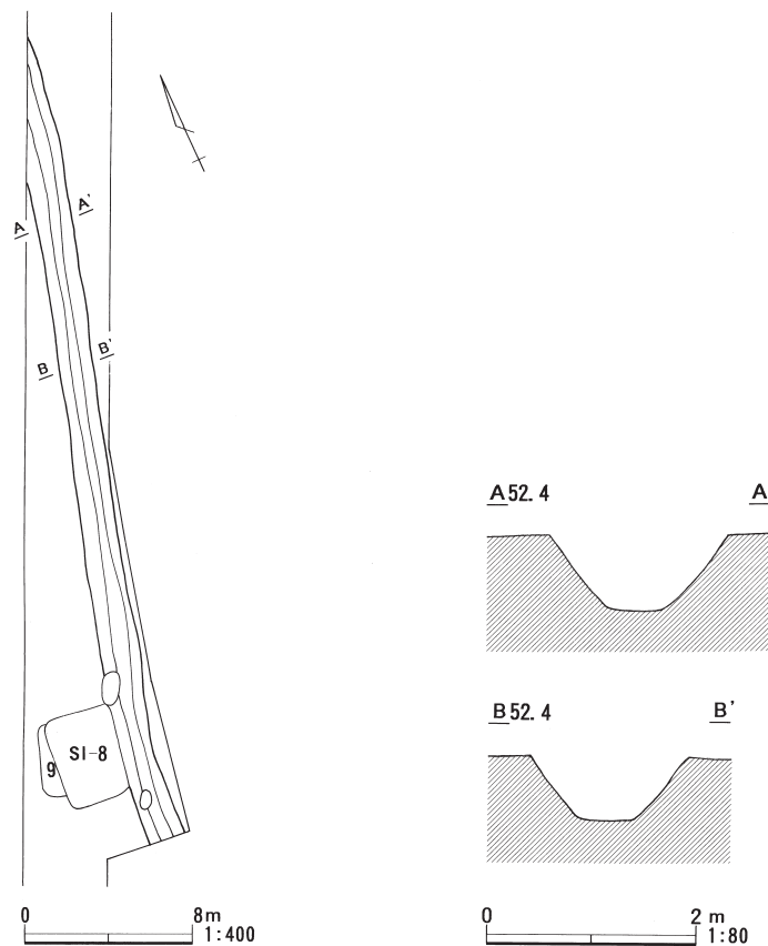
図50 石神境遺跡SD-1平面図および断面図
