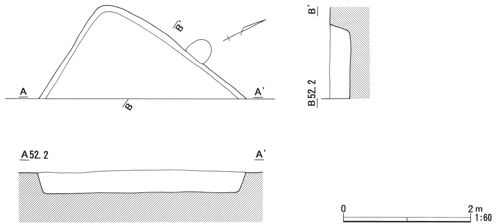
図26 石神境遺跡SI-11平面図および断面図
