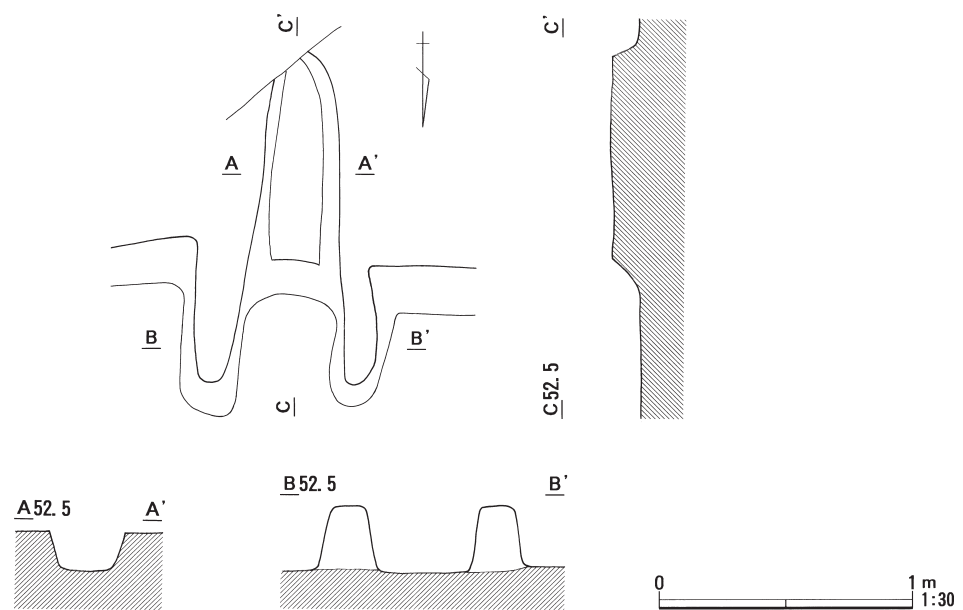
図13 石神境遺跡SI-5カマド平面図および断面図
