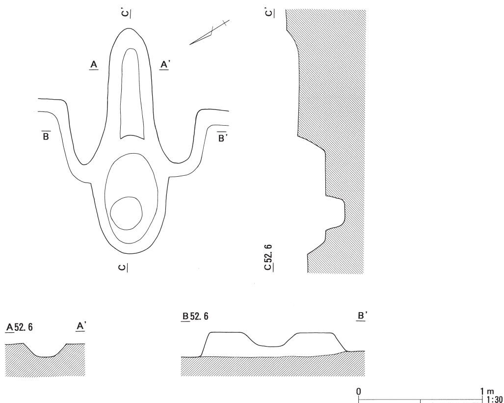
図18 石神境遺跡SI-7カマド平面図および断面図
