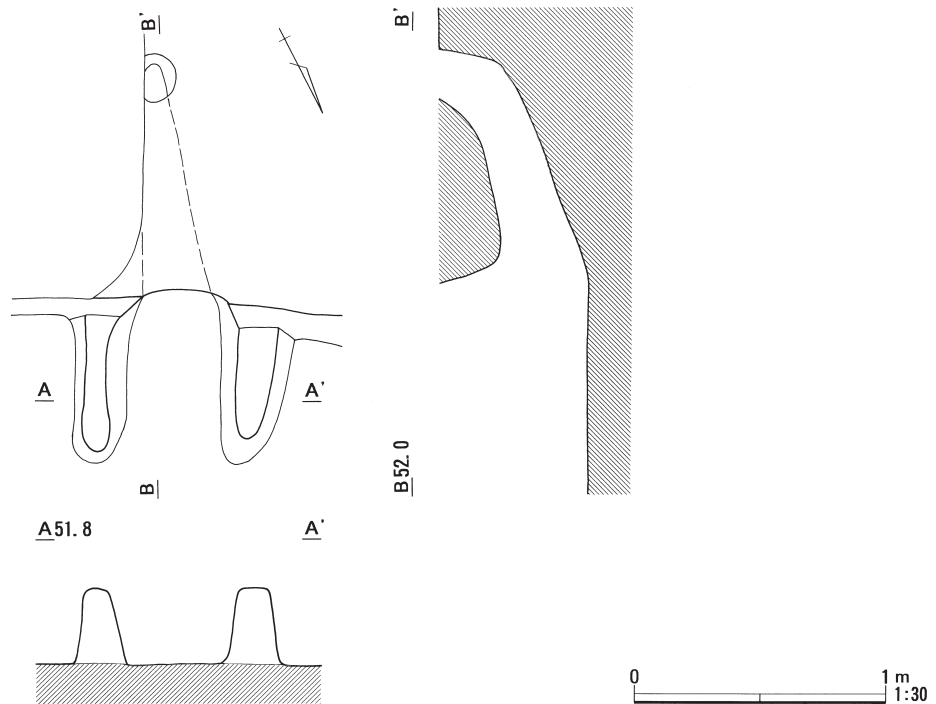
図46 石神境遺跡SI-22カマド平面図および断面図
