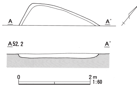
図38 石神境遺跡SI-18平面図および断面図
