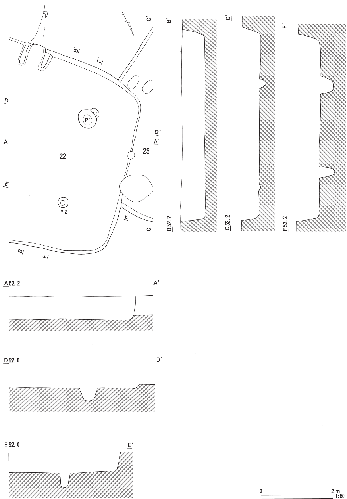
図45 石神境遺跡SI-22・23平面図および断面図
