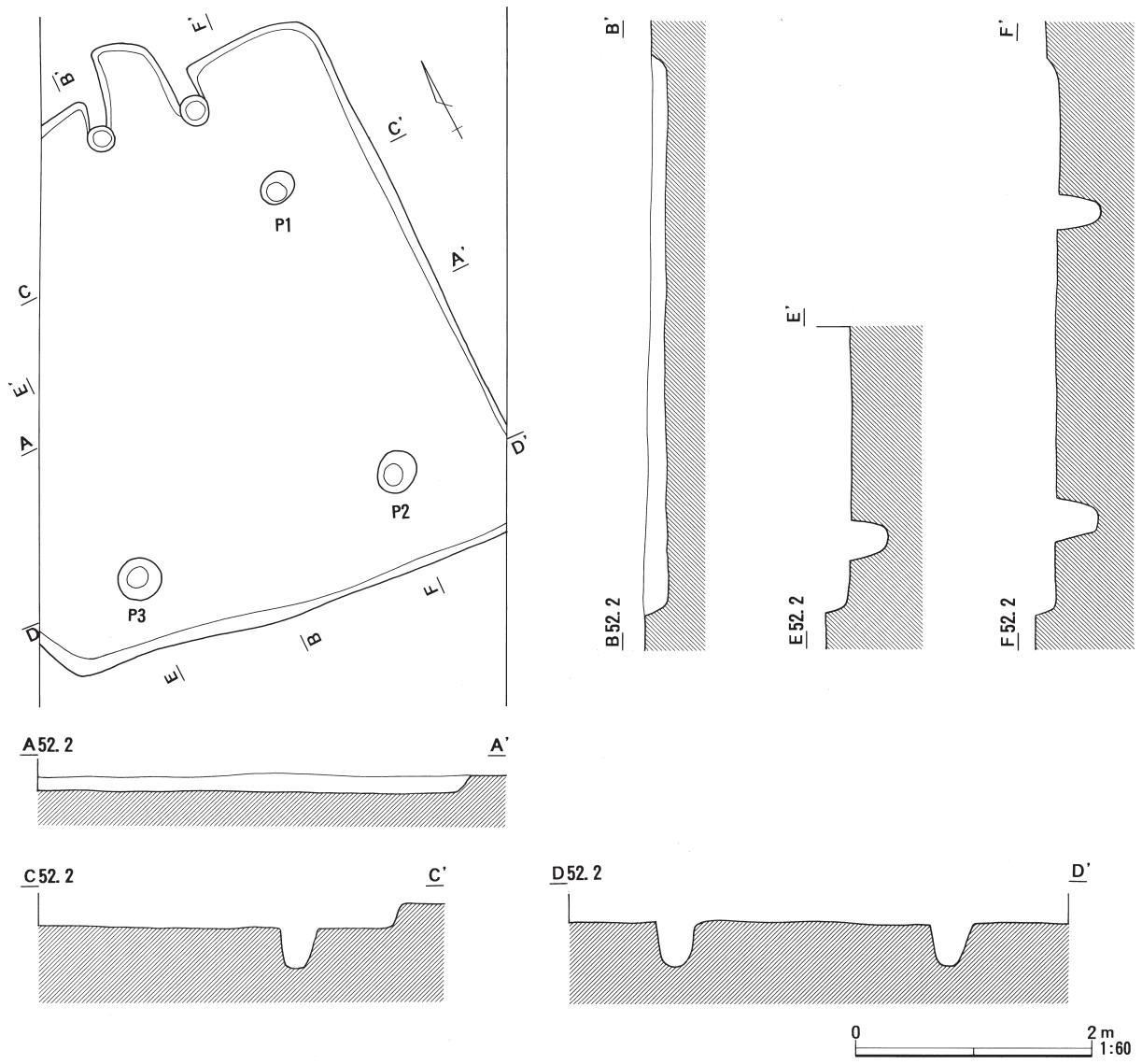
図30 石神境遺跡SI-14平面図および断面図
