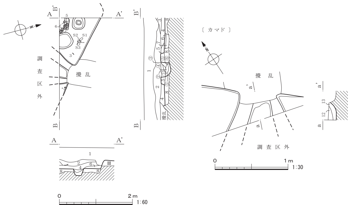
第8図 第10号住居跡平面図・断面図
