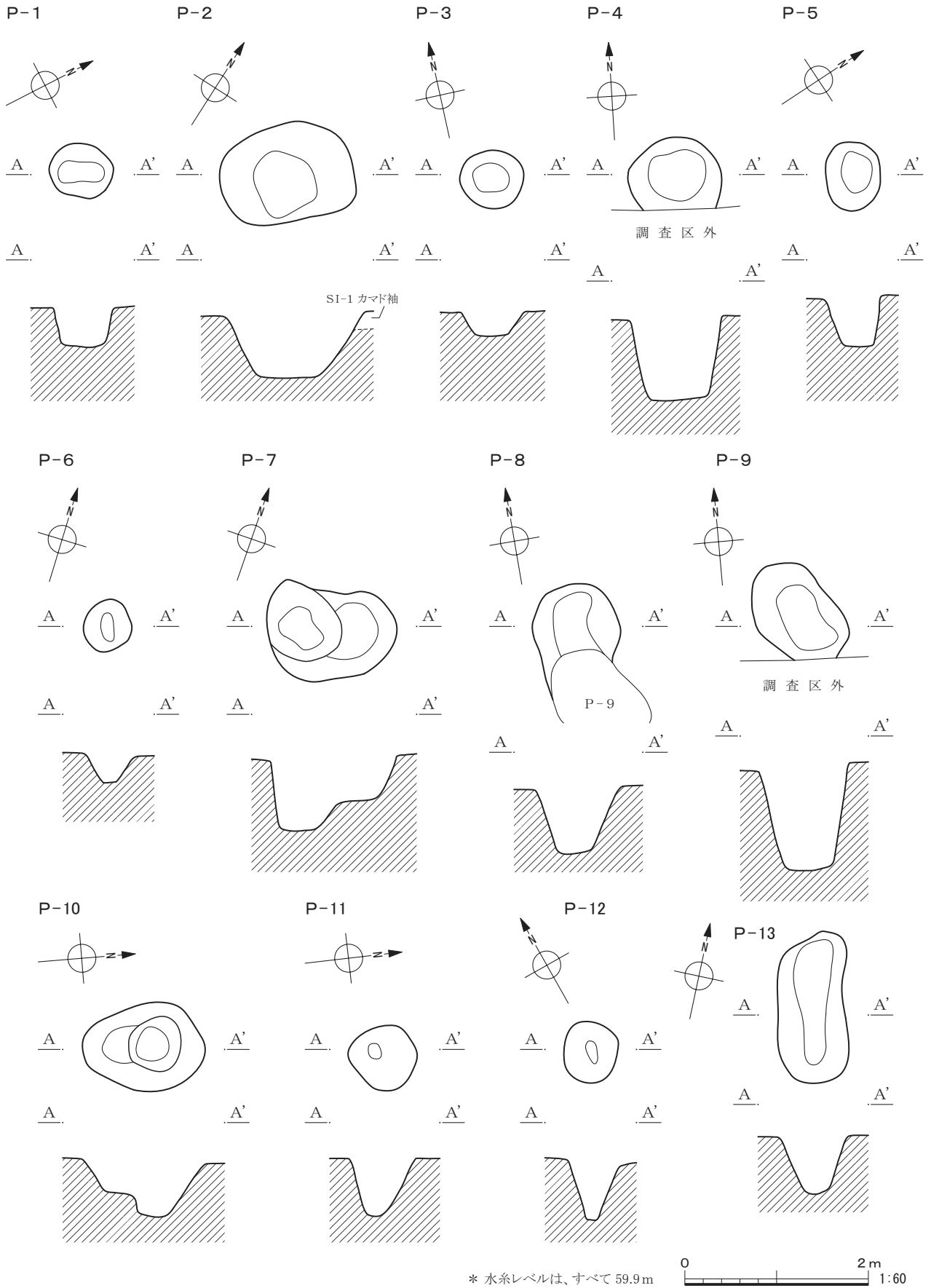
第33図 第1～13号ピット平面図・断面図
