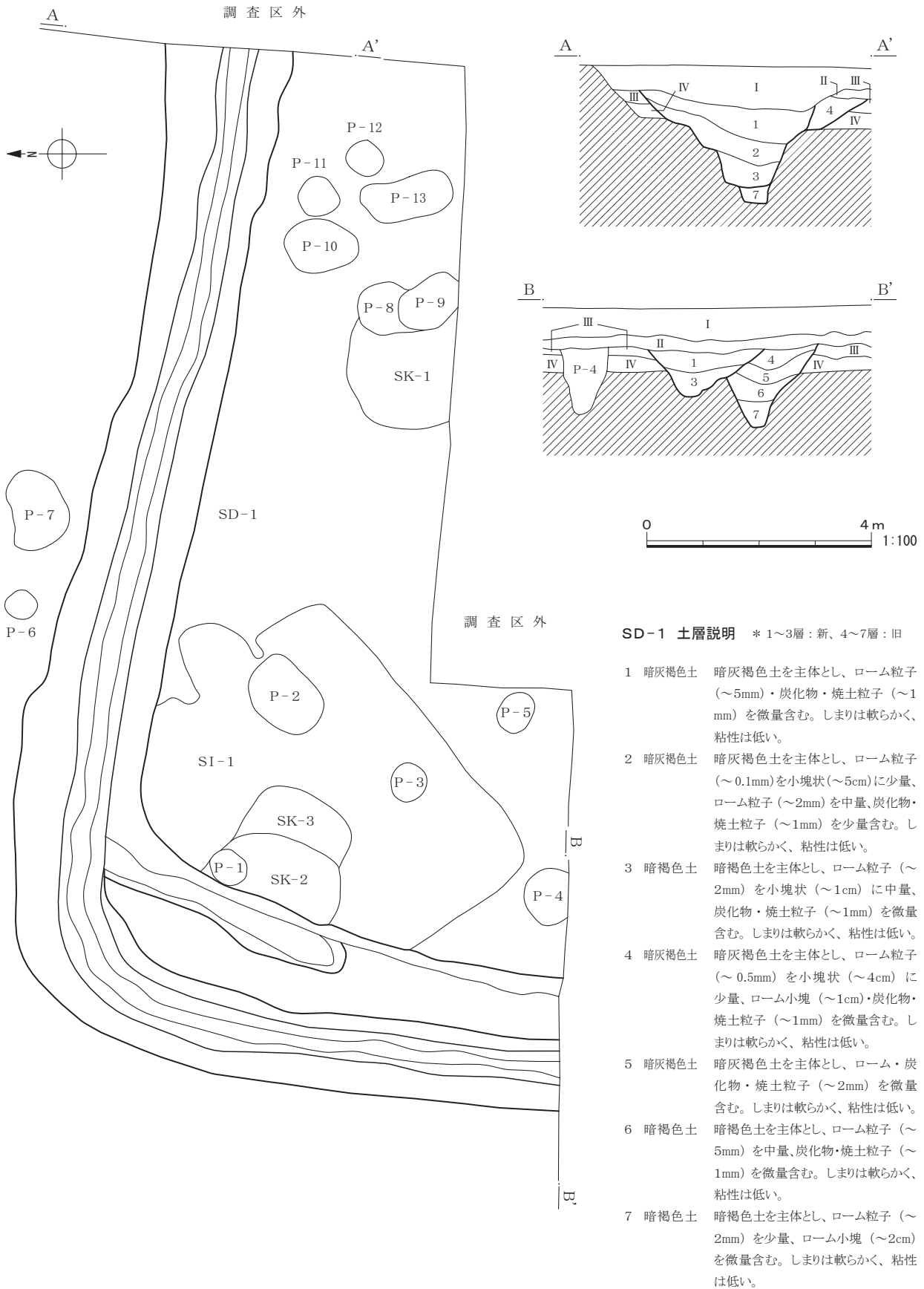
第 28 図 第 1 号溝址平面図・断面図
