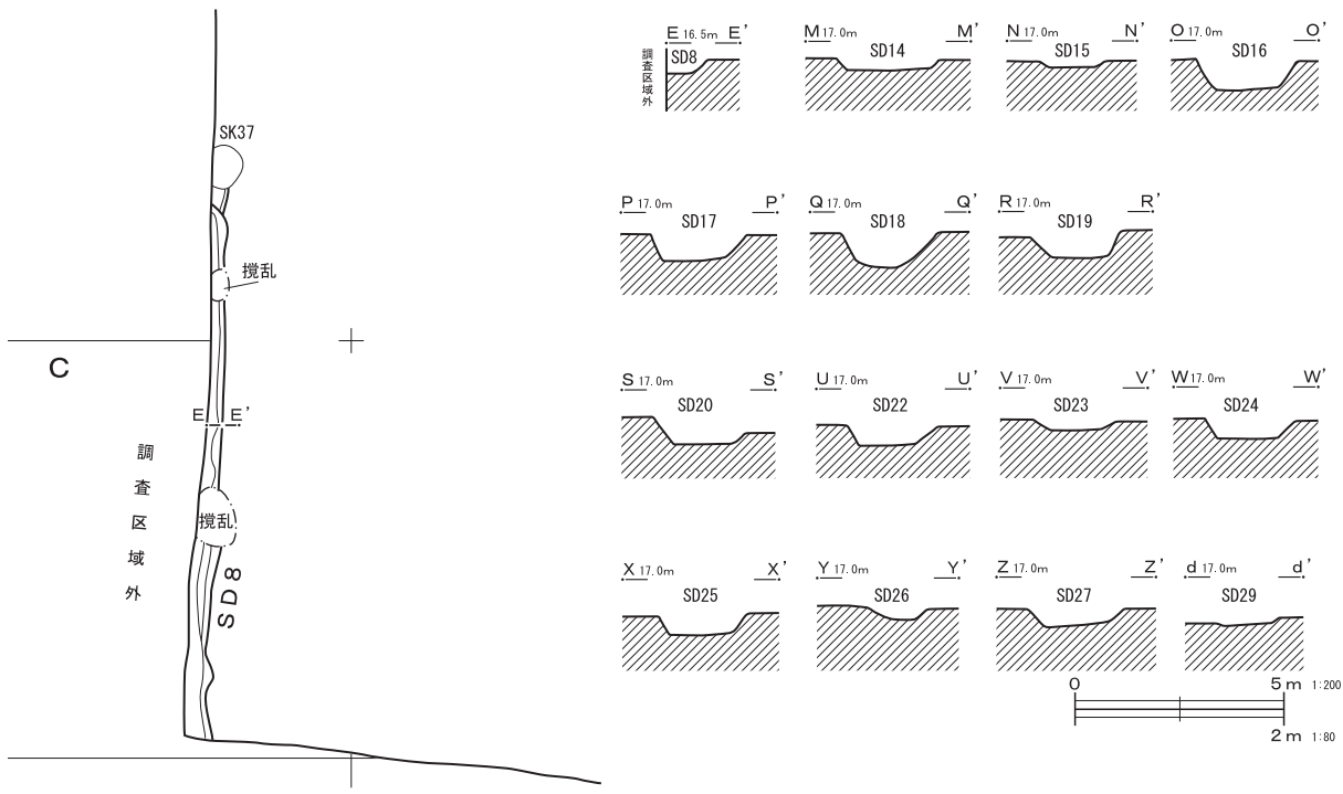
第200図 溝跡 (4)
