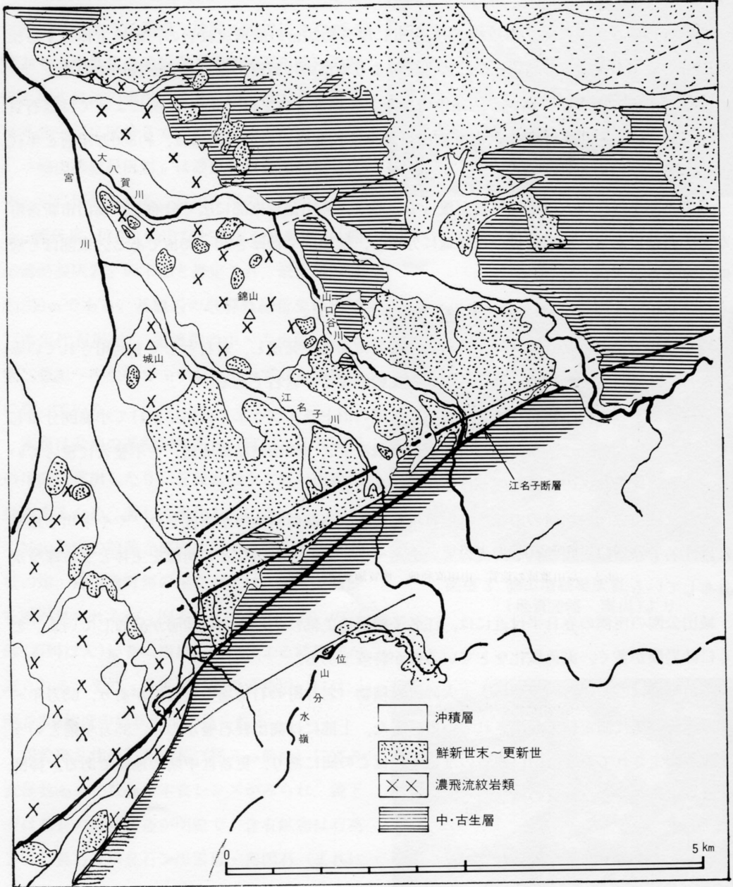
挿図7 地質概念図 (高山図幅による)
