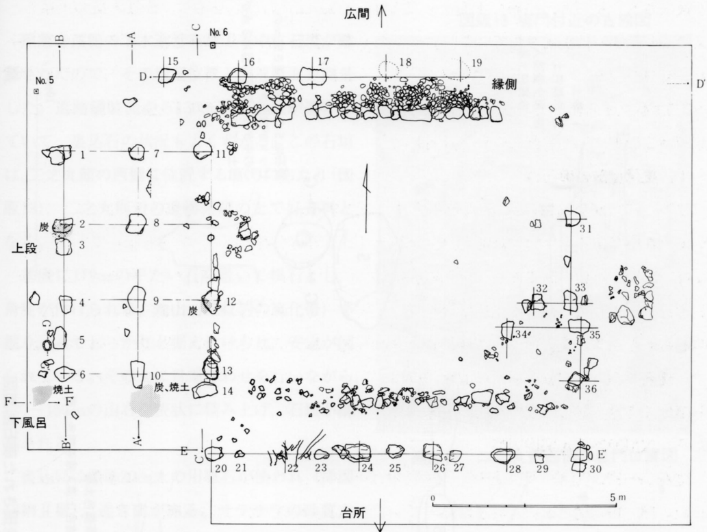
挿図15 発掘された礎石実測図
