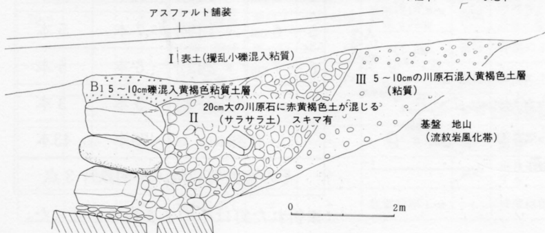
挿図18 二之丸館西側唐門付近の断面図
