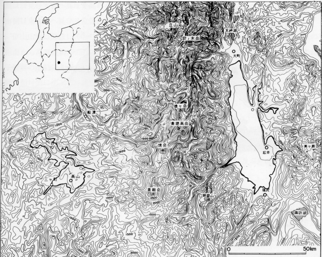
挿図1 松本盆地、高山盆地の接峰図面(第四紀No.19 1973より引用)
