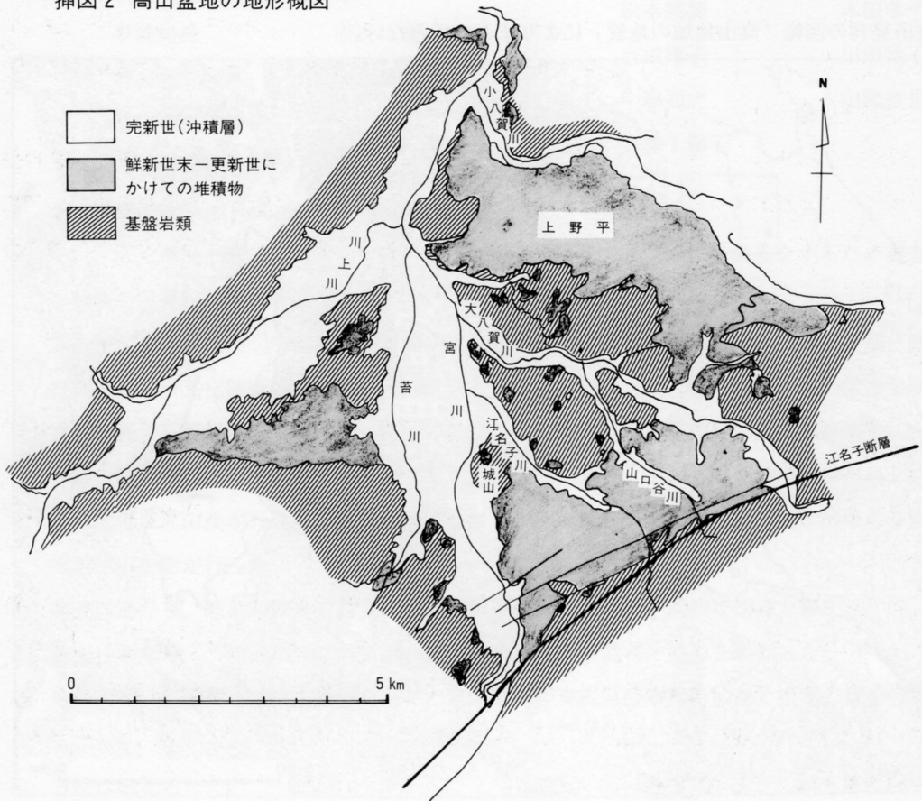
挿図2 高山盆地の地形概図
