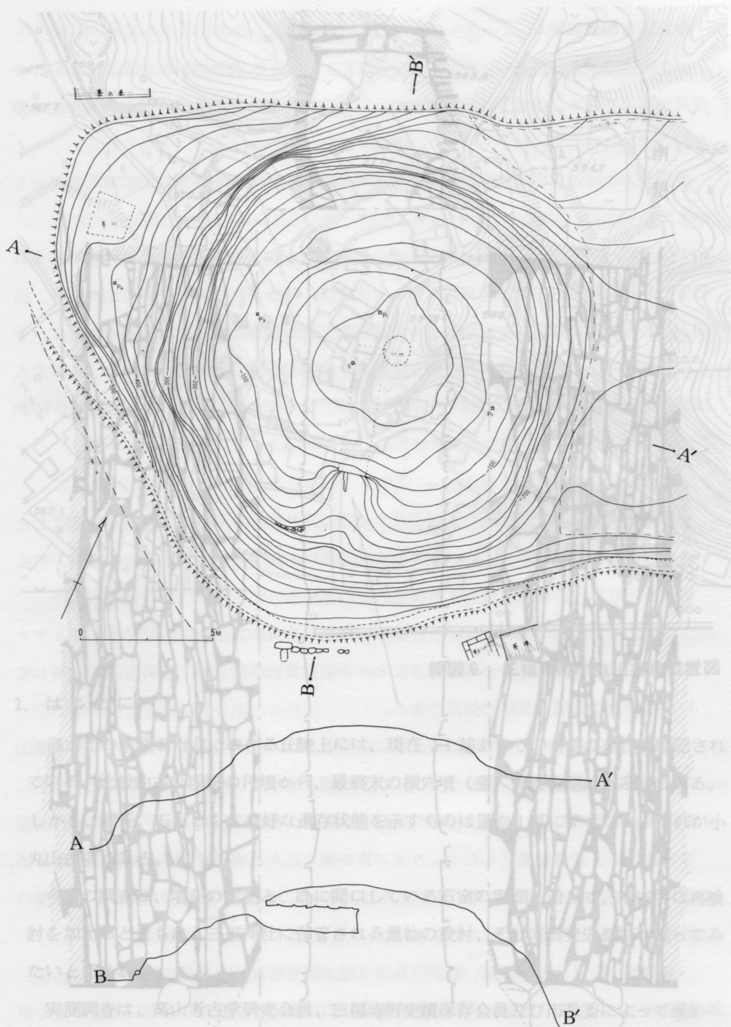
挿図4. 三福寺町小丸山古墳墳丘平面図及び断面図
