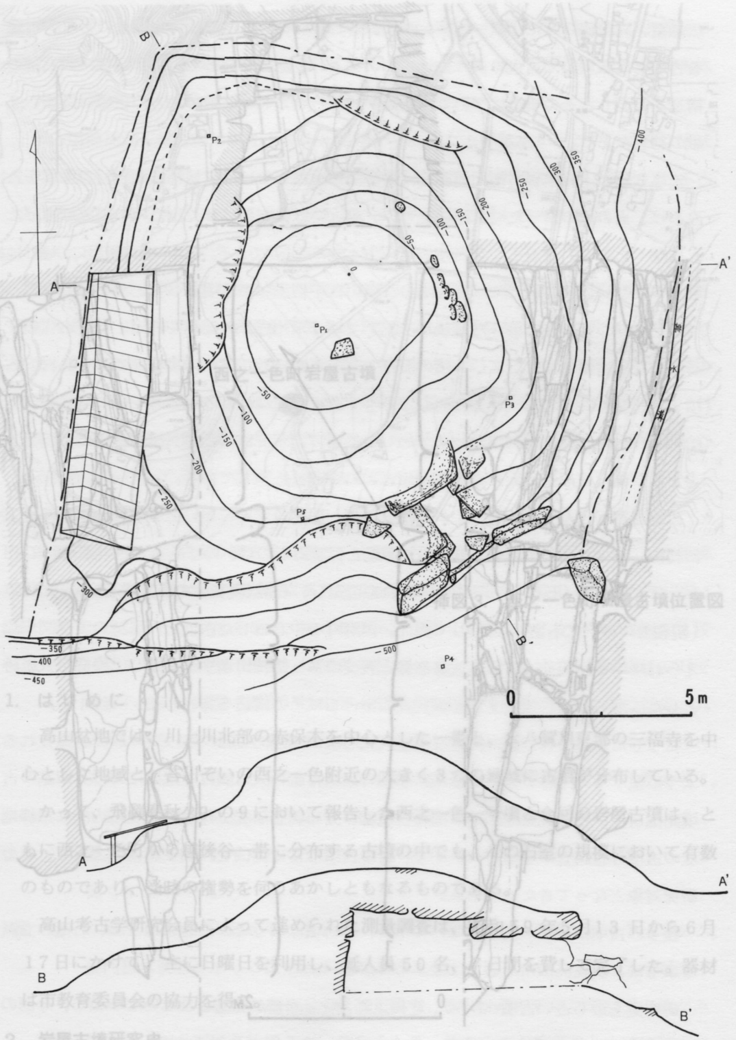
図 西之一色町岩屋古墳墳丘平面図及び断面図
