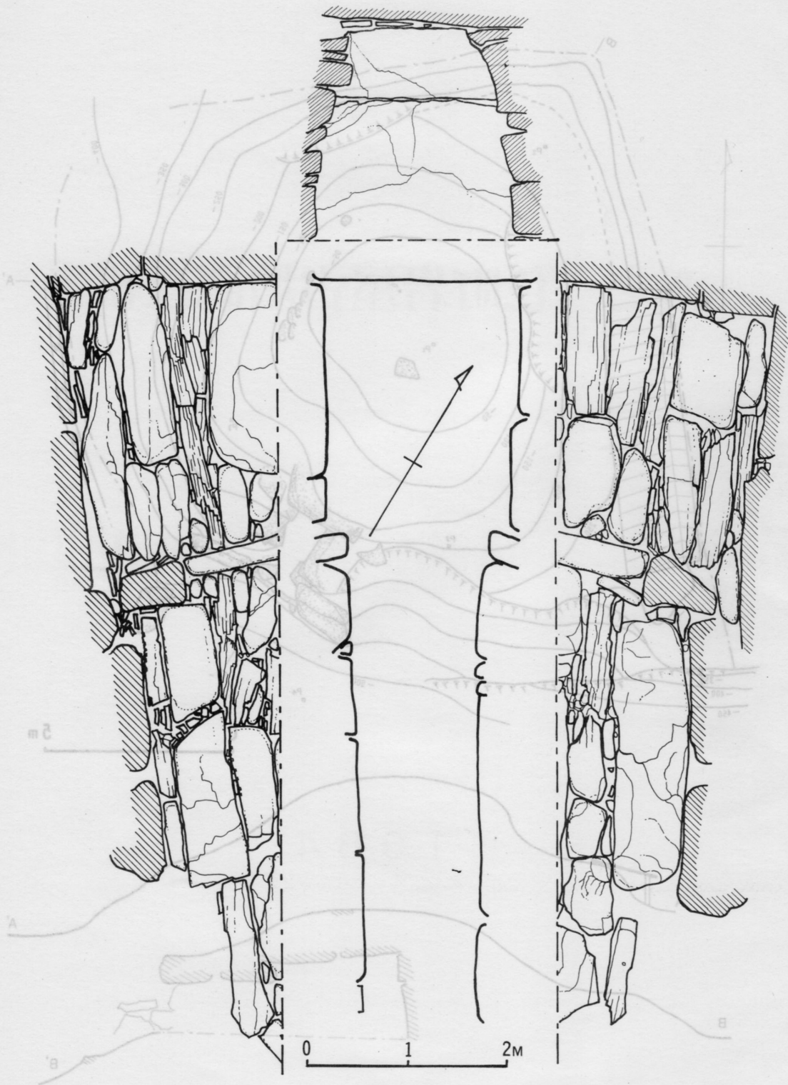
西之一色町岩屋古墳石室実測図 挿図 2. 西之一色町岩屋古墳石室実測図
