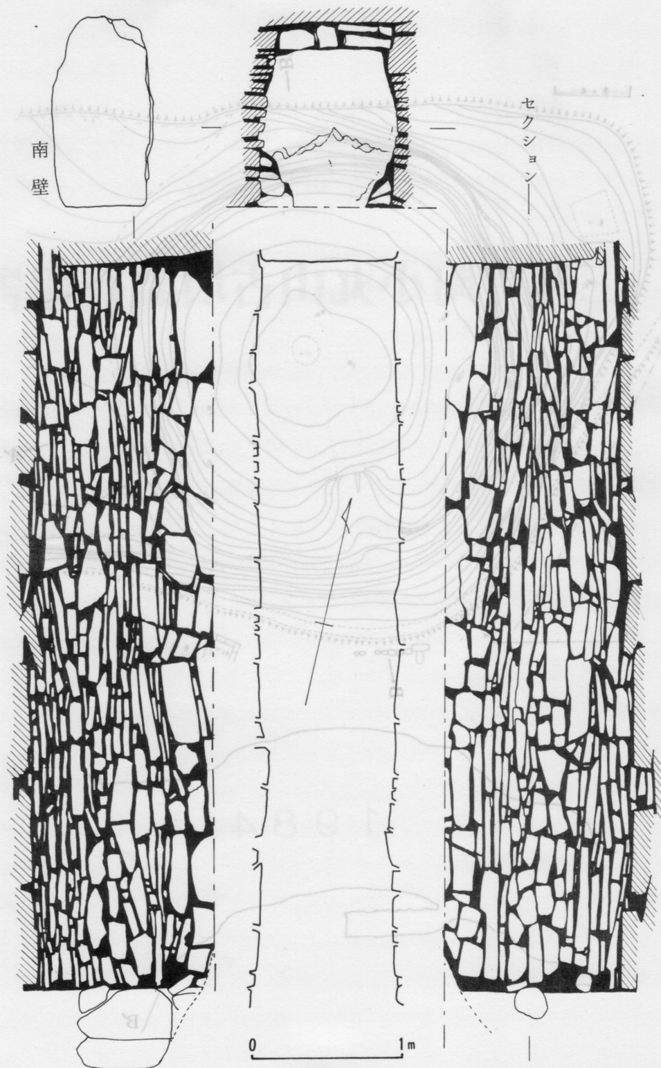
三福寺町小丸山古墳石室実測図 挿図5. 三福寺町小丸山古墳石室実測図
