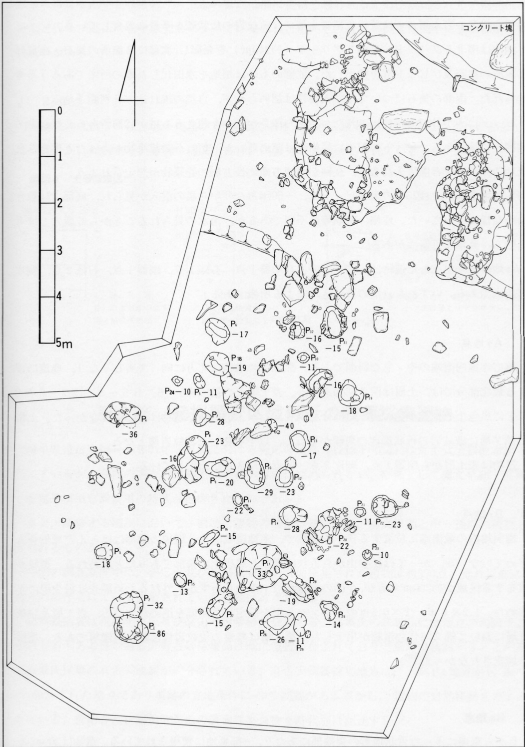
挿図8 掘立柱遺構(SB01)実測図
