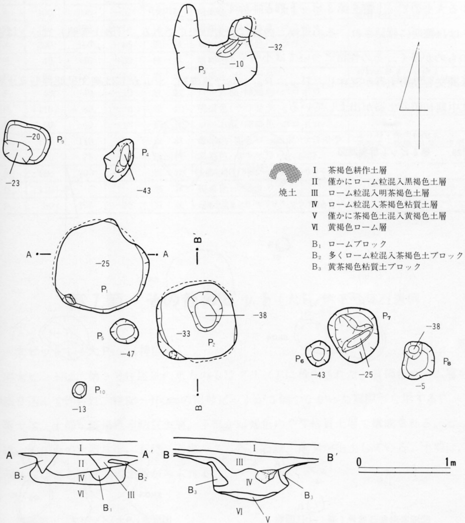
挿図28 第1ピット群実測図
