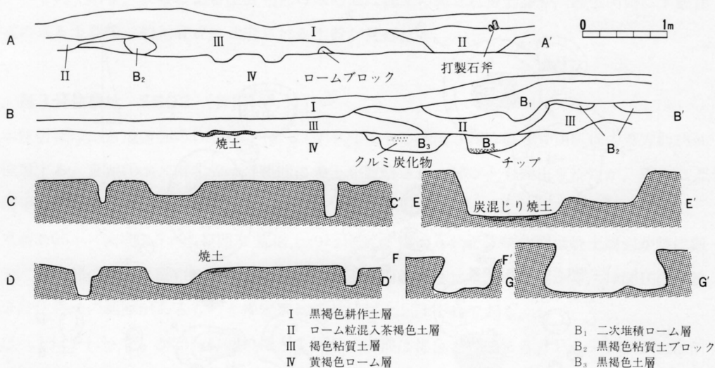
挿図17 第3号住居址(SB03)土層断面図
