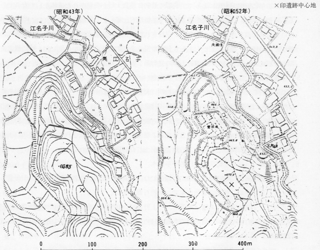
挿図2 昭和43年と昭和52年の地形図
