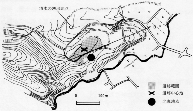
挿図3 向畑地区の地形図
