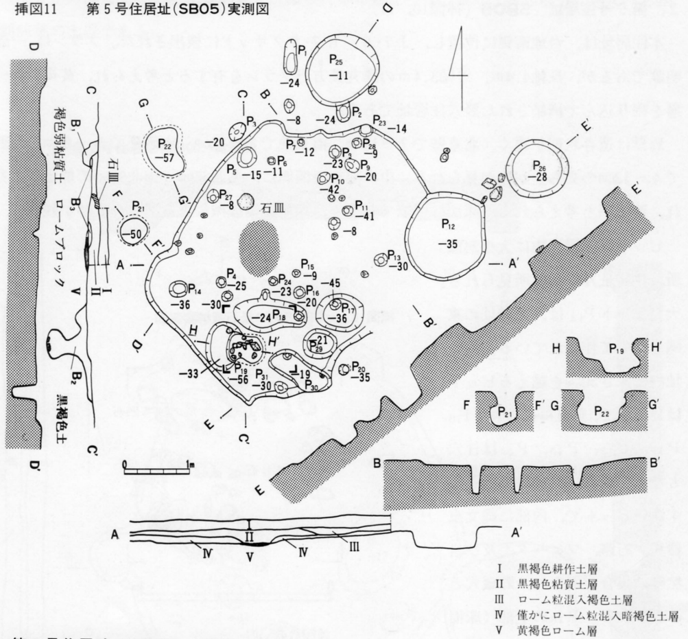
挿図11 第5号住居址(SB05)実測図
