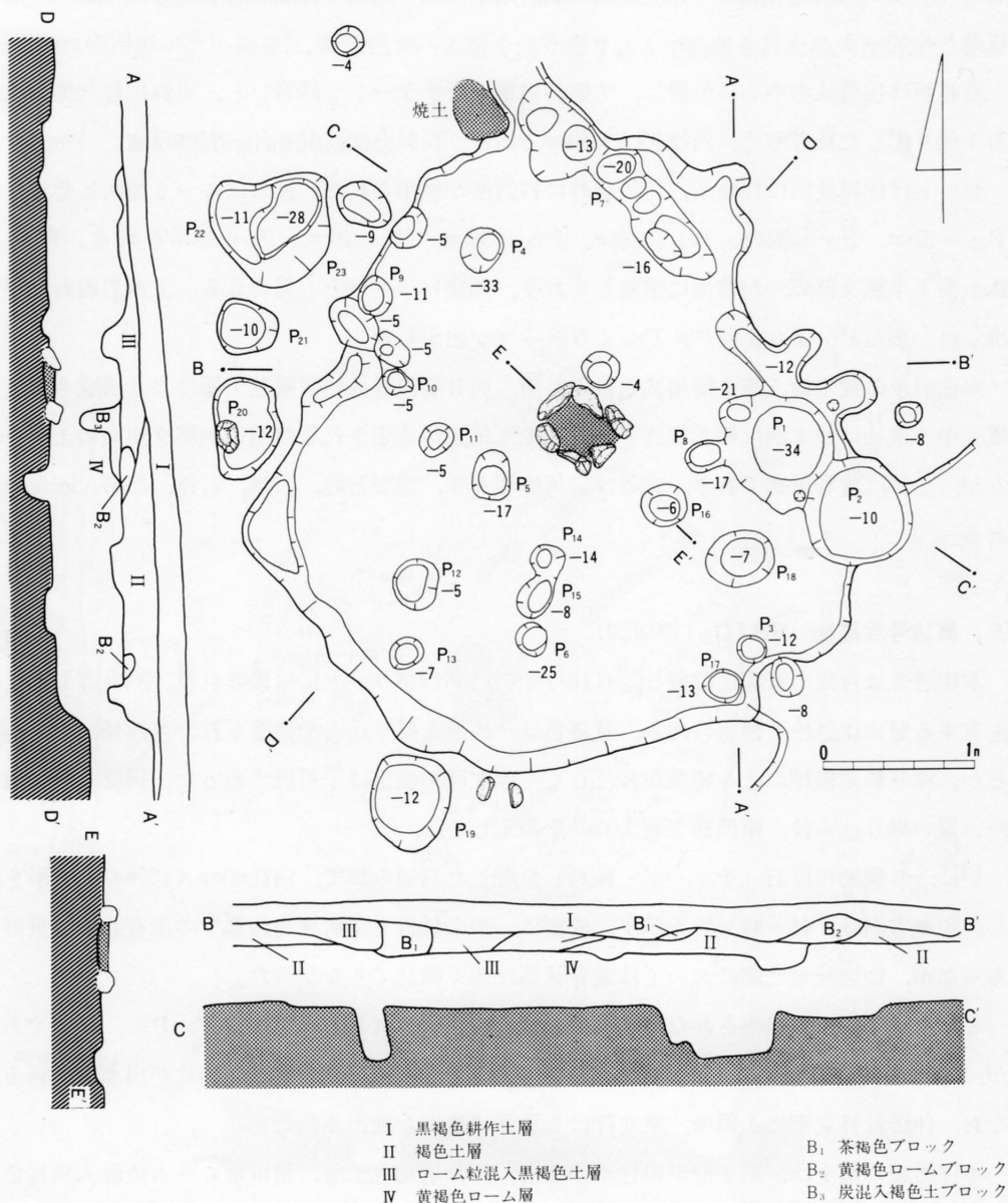
挿図20 第10号住居址(SB10)実測図
