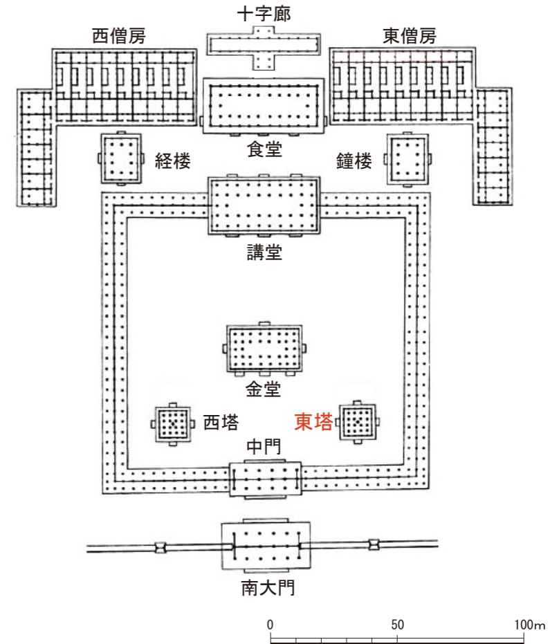
図6 薬師寺伽藍配置図
