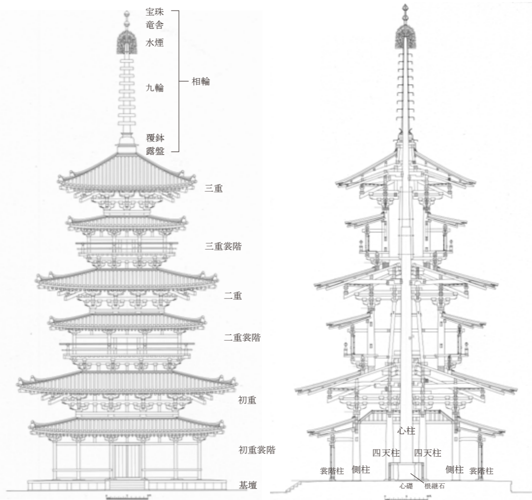
図3 東塔の各部名称
