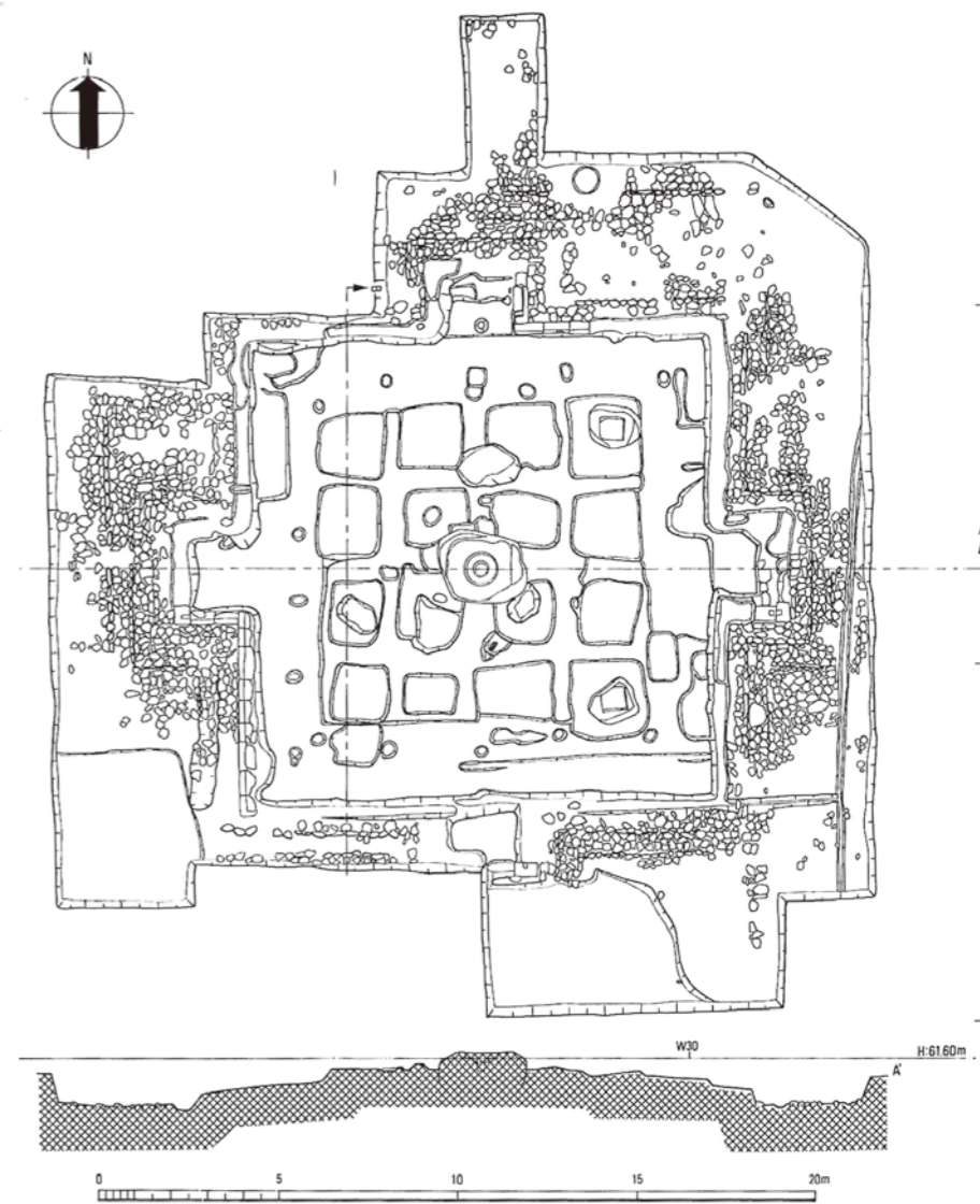
【参考】薬師寺西塔平面・断面図
