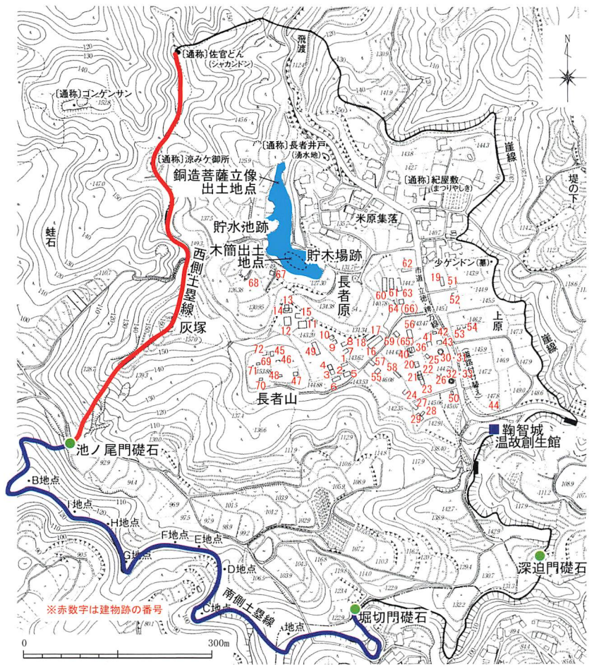
鞠智城跡全体図
