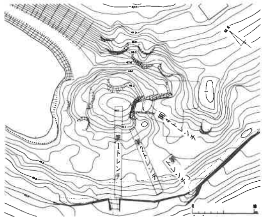
第8図 調査トレンチ配置図
