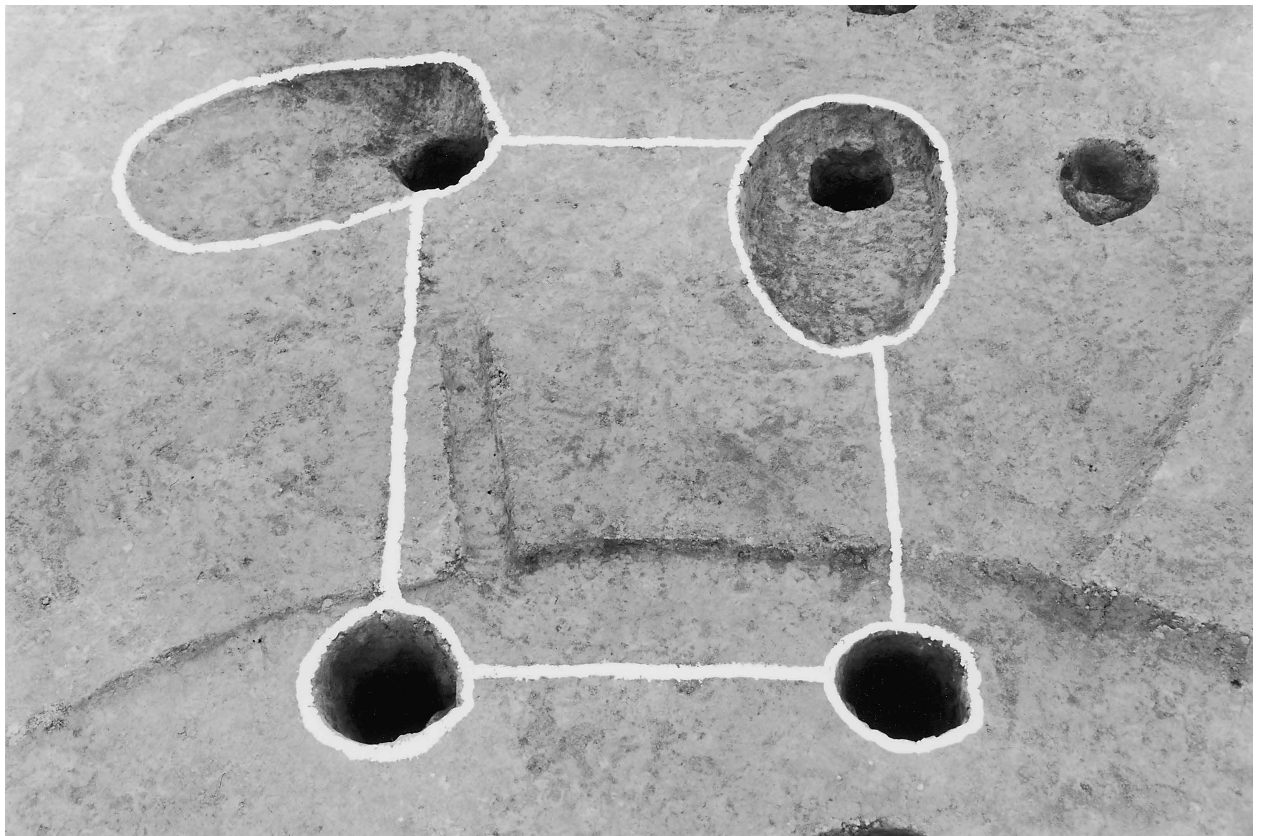
2 第5号掘立柱建物跡
