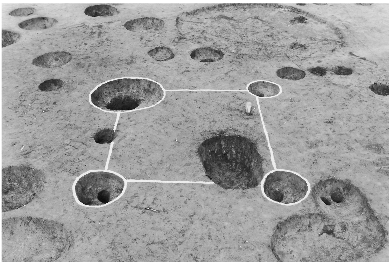
2 第7号掘立柱建物跡
