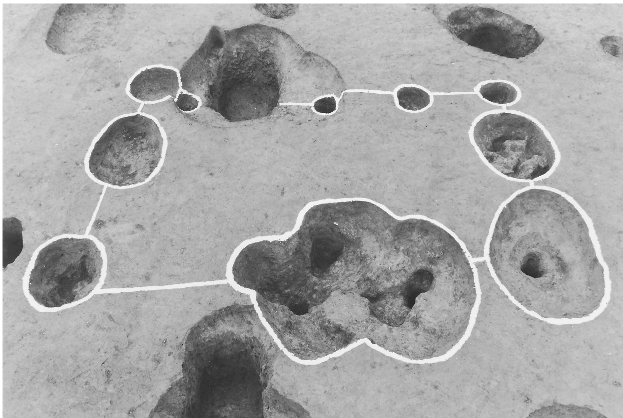
1 第10号掘立柱建物跡
