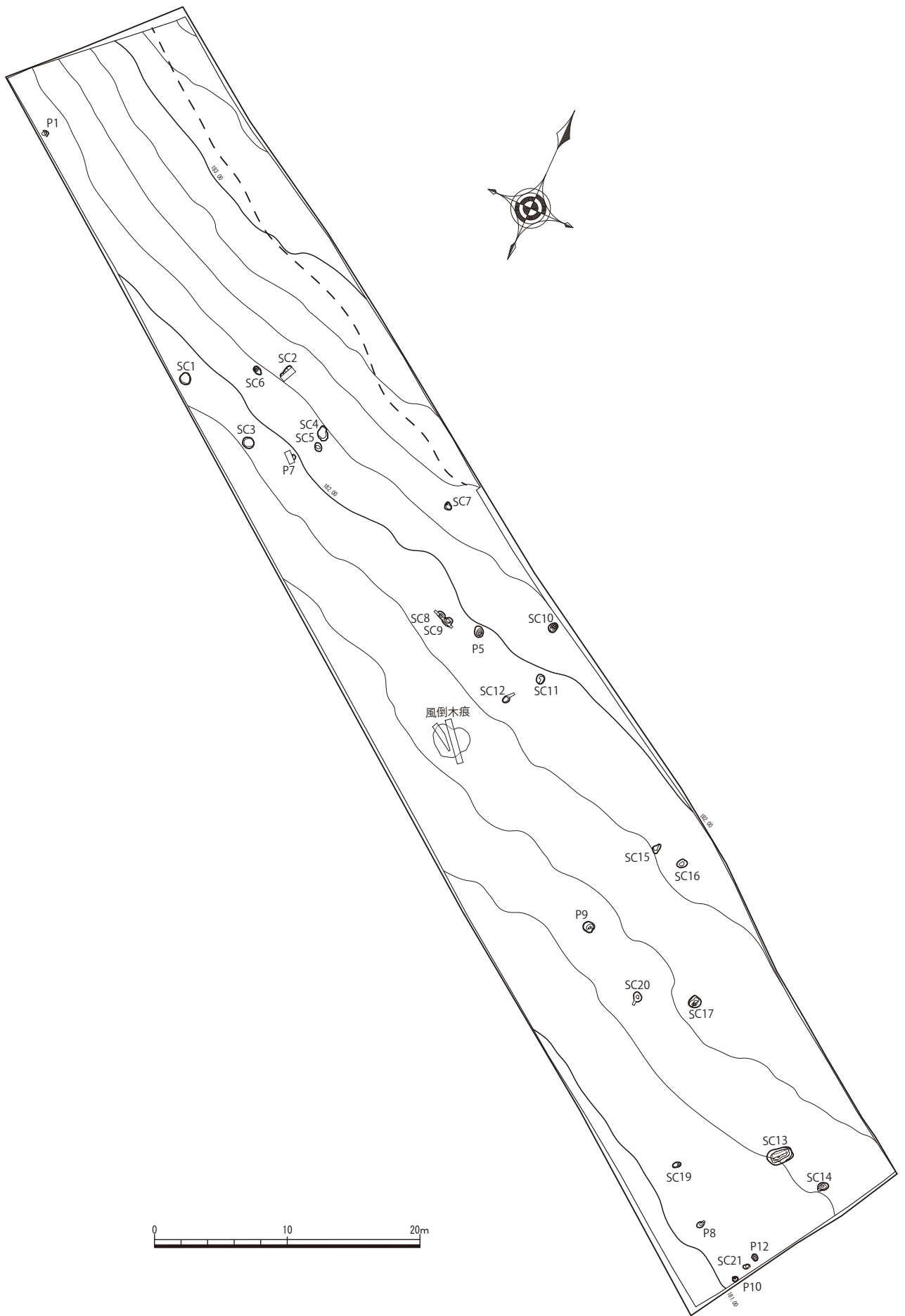
第6図 遺構配置図 (S=1/400)
