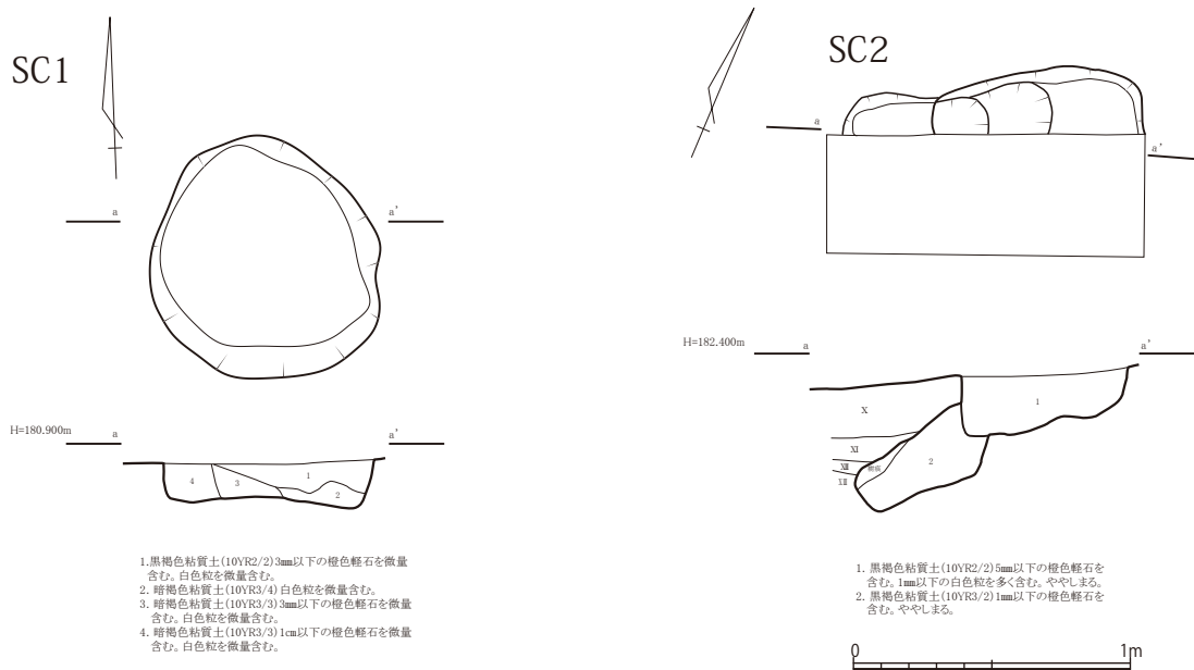
第7図 SC実測図① (S=1/30)
