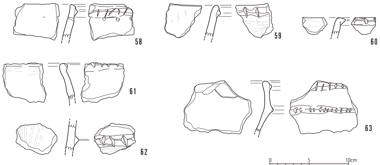
第18図 包含層出土土器実測図⑥(S=1/3)
