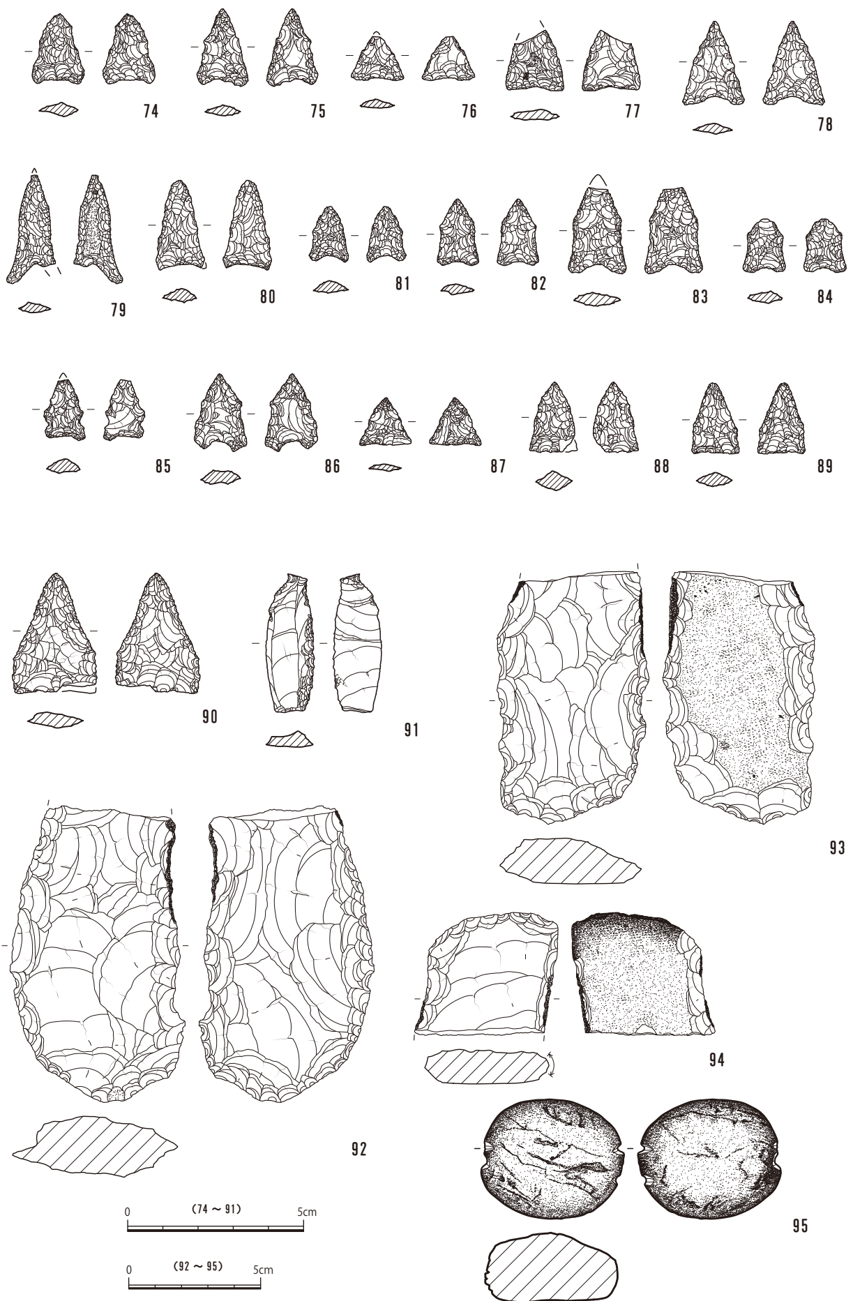
第 21 图 包含層出土石器实测图 (S= 2/3 · 1/2)
