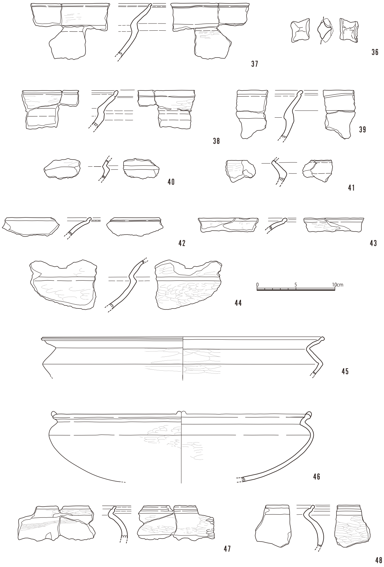
第 16 图 包含層出土土器实测图④ (S=1/3)
