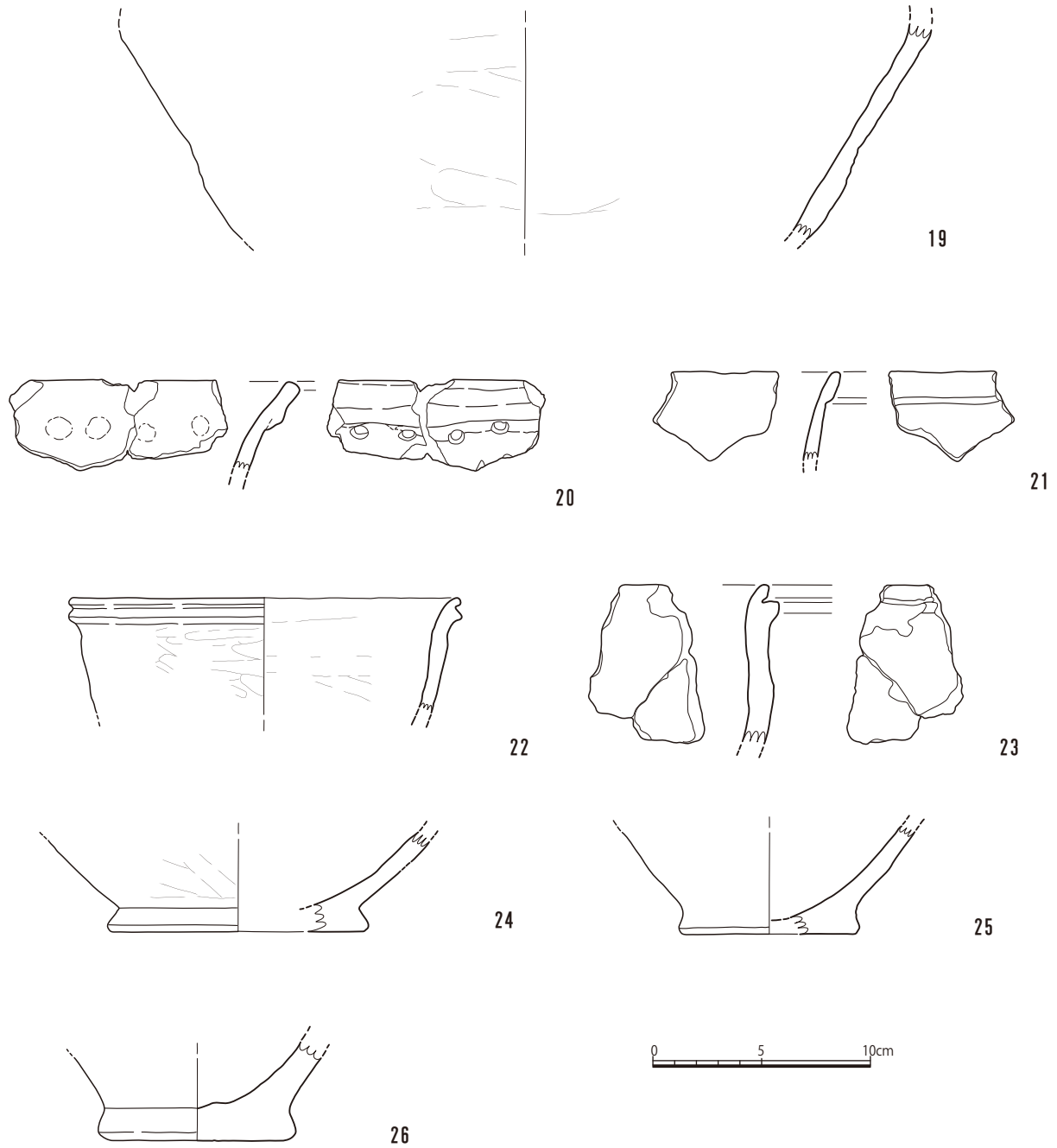
第14図 包含層出土土器実測図②(S=1/3)
