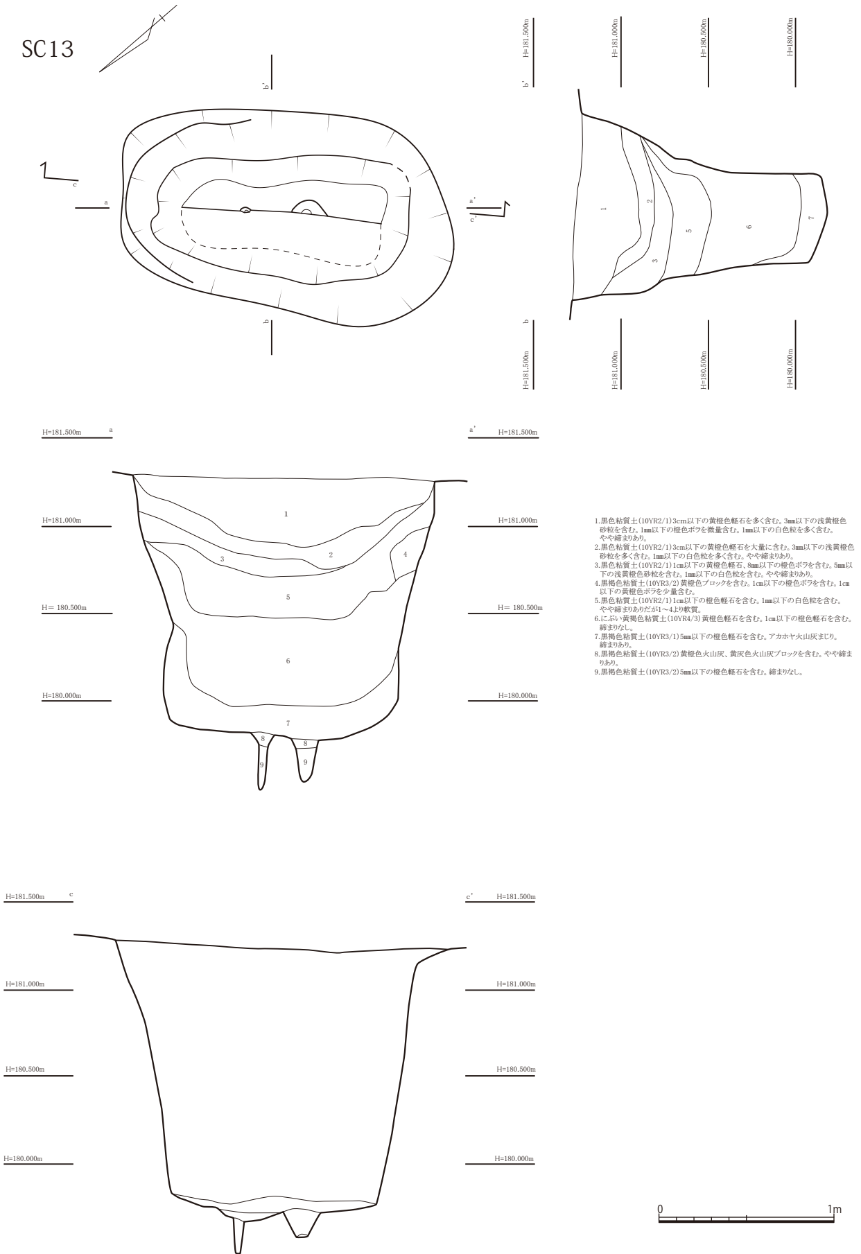
第 10 図 SC 実測図④ (S=1/30)
