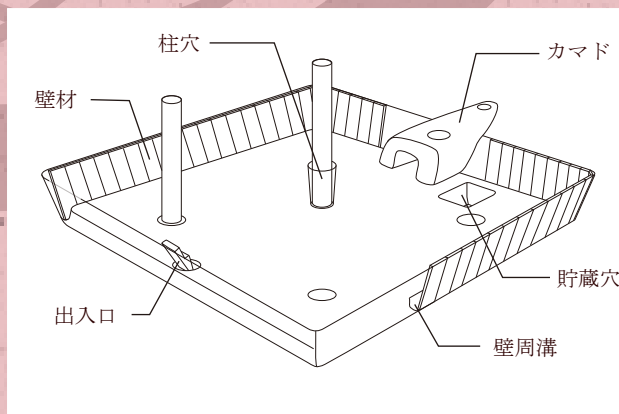
竪穴住居の構造
