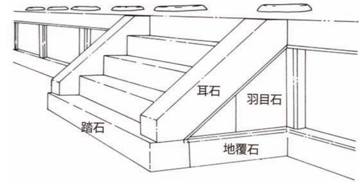
図5 階段の模式図
