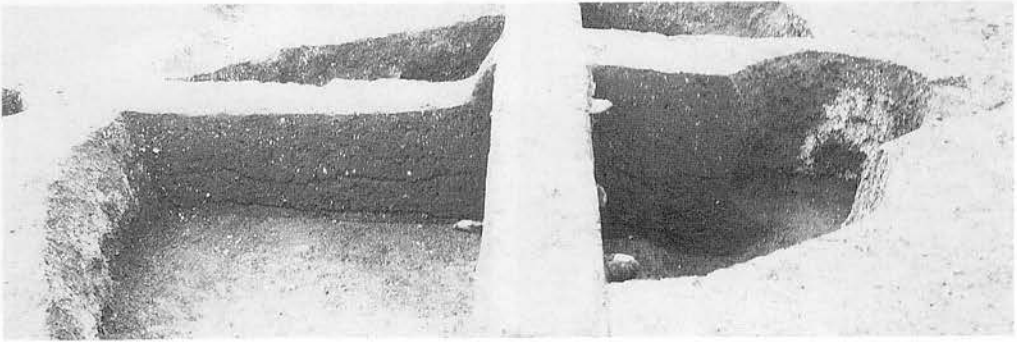
SA68断面
