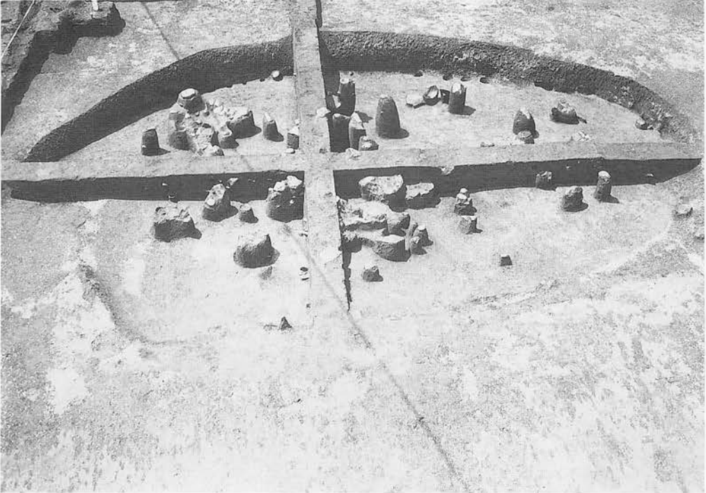
SA07断面
