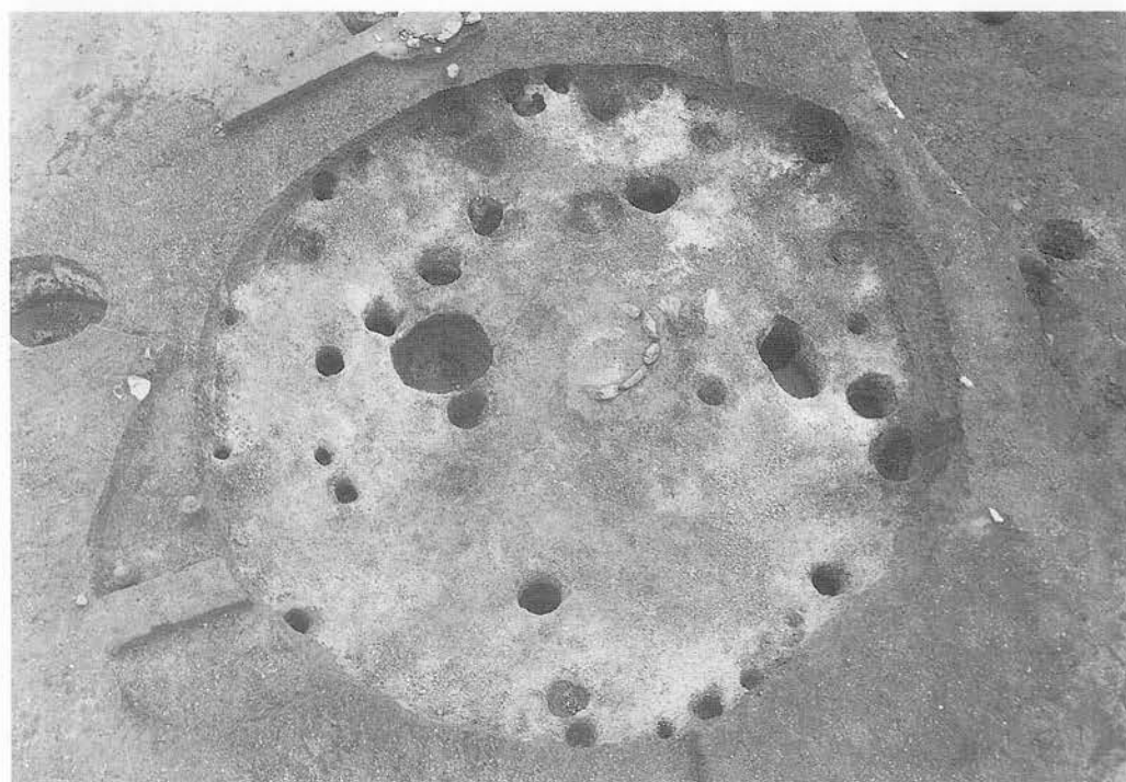
SA41平面
