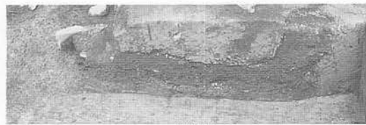
煙道部
