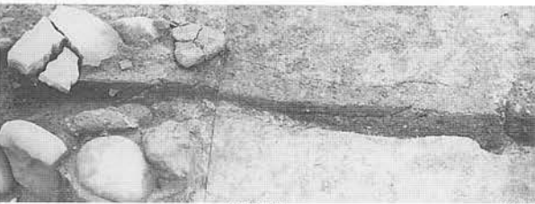
煙道部
