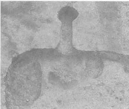
カマド
