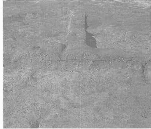
焼土 断面
