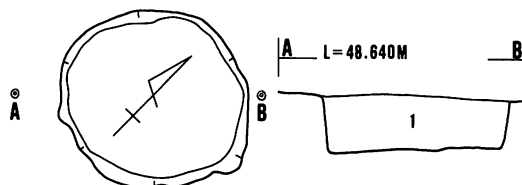
第 10 図 F 20 土坑
