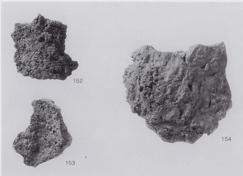
第2号炉出土炉壁・羽口（2） 第34図
