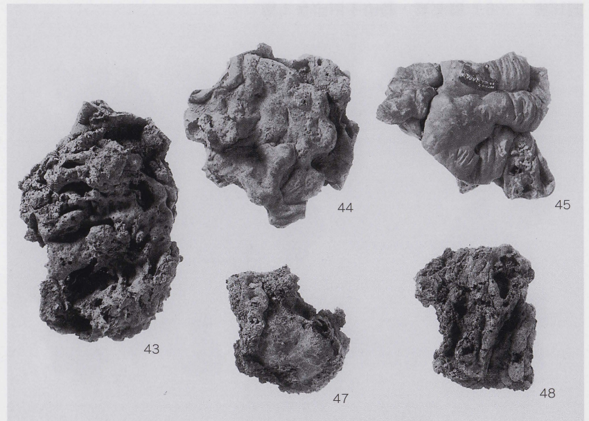
第1号炉出土炉壁・鉄滓類（6） 第18・19图
