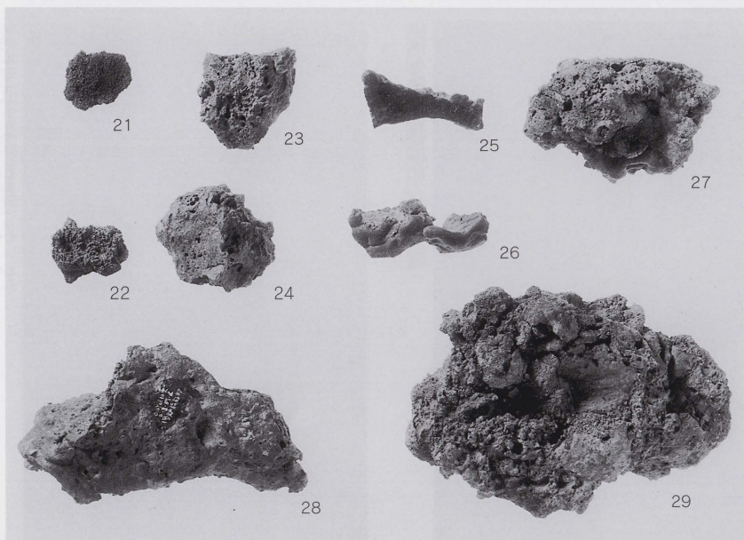
第1号炉出土炉壁・鉄滓類（4） 第16图
