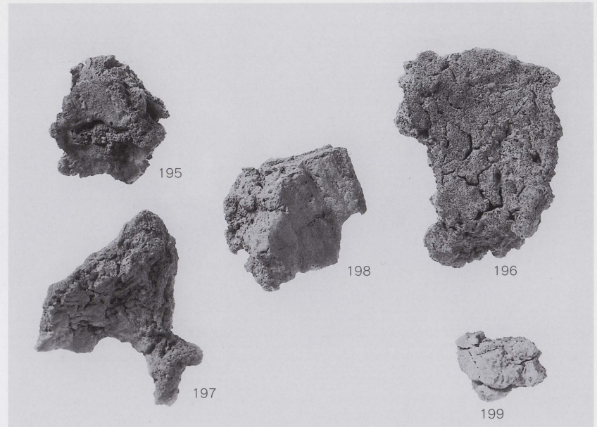
第3号炉出土炉壁・羽口・鉄滓(1) 第34图
