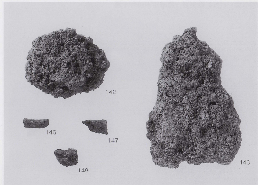
第1号炉出土炉壁・鉄滓類（10） 第21図
