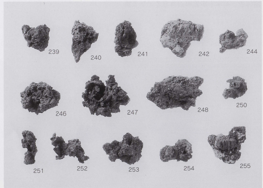
第3号炉出土炉壁・羽口・鉄滓(2)
