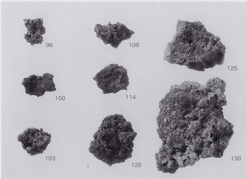
第1号炉出土炉壁・鉄滓類（8） 第20・21图
