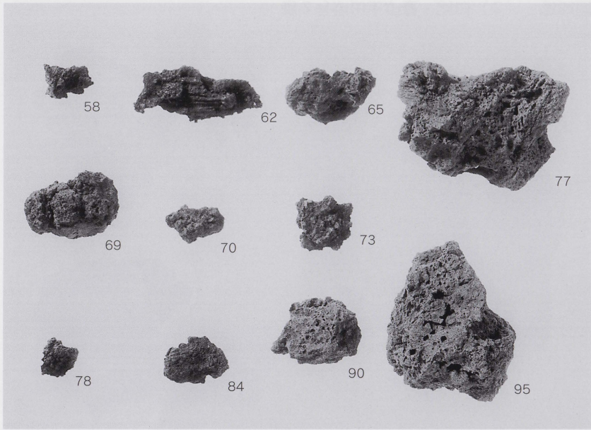
第1号炉出土炉壁・鉄滓類（7） 第19・20图
