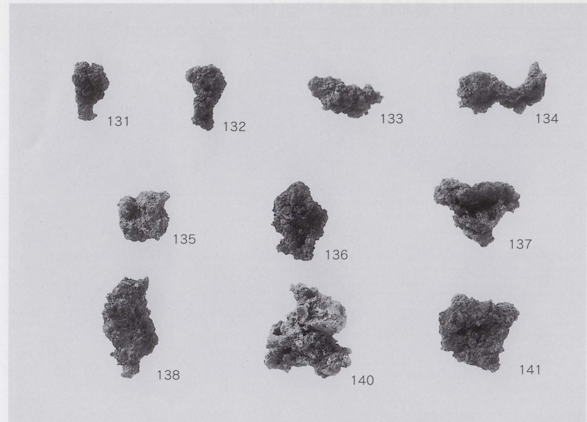
第1号炉出土炉壁・鉄滓類（9） 第21図
