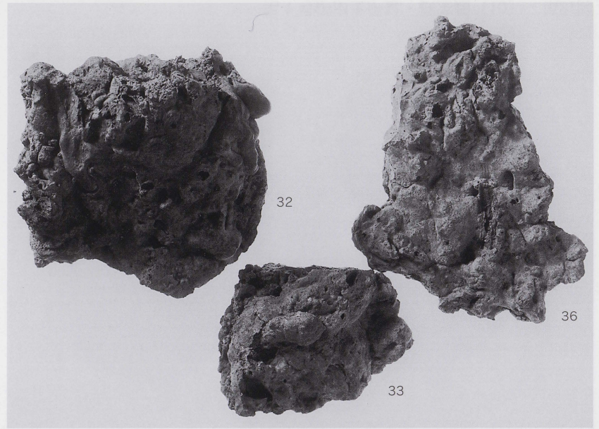
第1号炉出土炉壁・鉄滓類（5） 第17图
