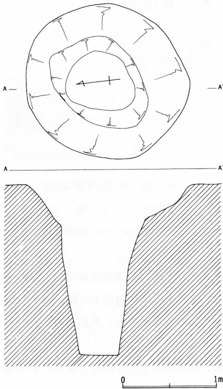
第4図 第1号井戸跡実測図
