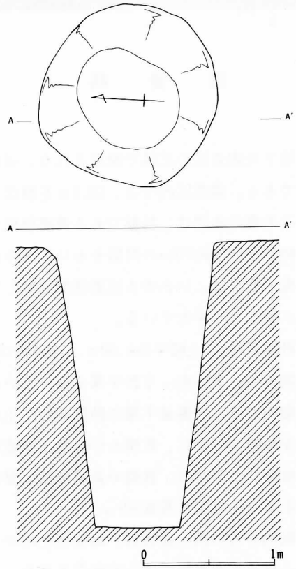
第5図 第2号井戸跡実測図
