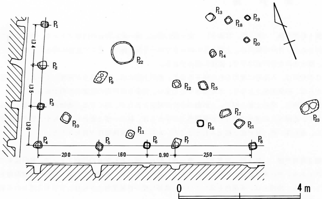
第3図 第1ピット群実測図
