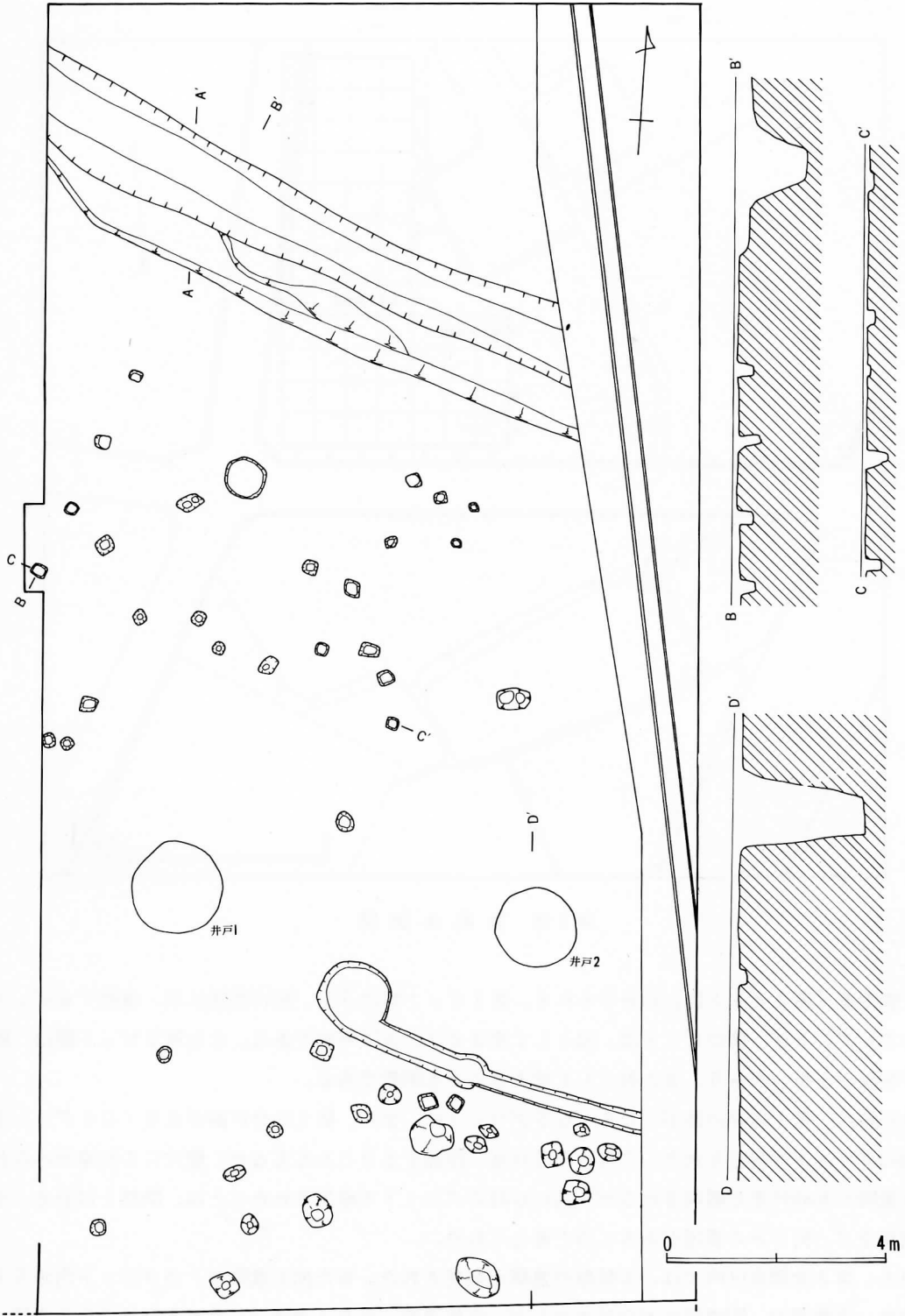
第2図 遺構全測図
