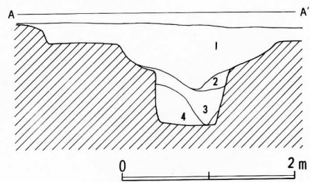
第6図 堀遺構断面図
