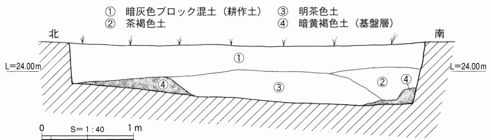
挿図10. 第8トレンチ土層断面図（東壁面）
