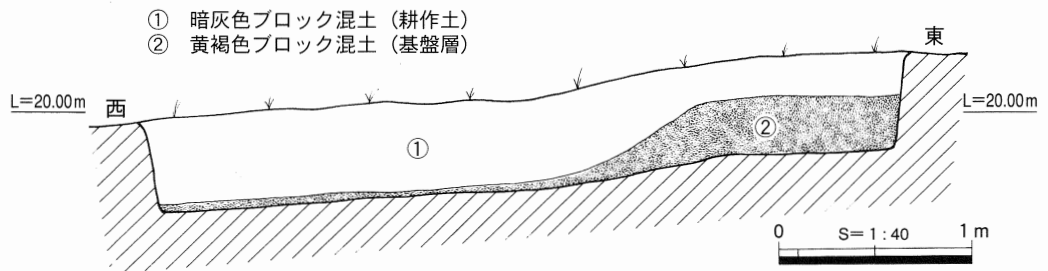
挿図15. 第11トレンチ土層断面図 (東壁面)
