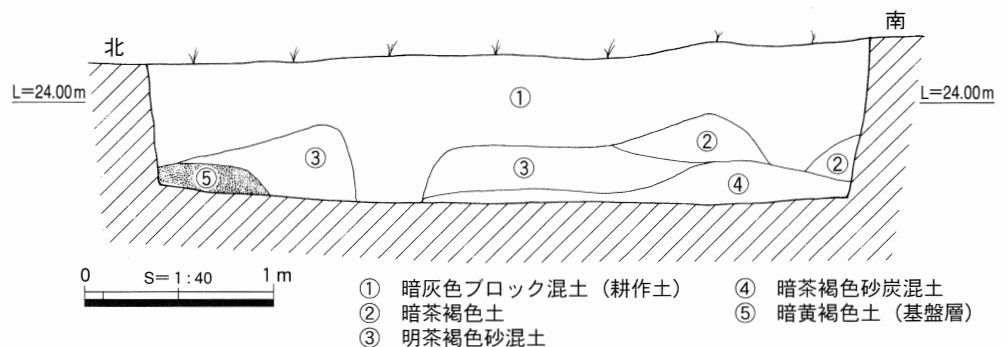
挿図16. 第12トレンチ土層断面図 (東壁面)
