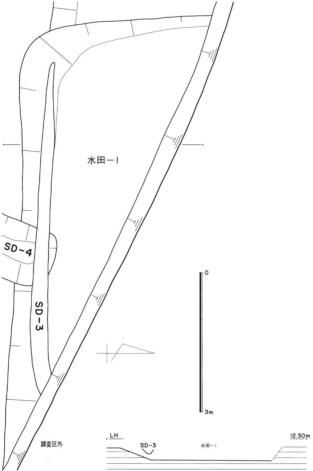
第7図 水田-1 実測図 (縮尺 1 : 50)
