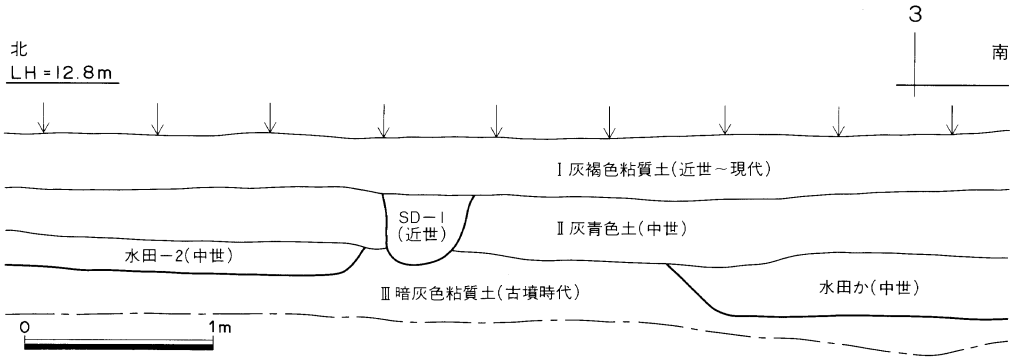
第4図 土層図(西調査区東壁 縮尺1:40)
