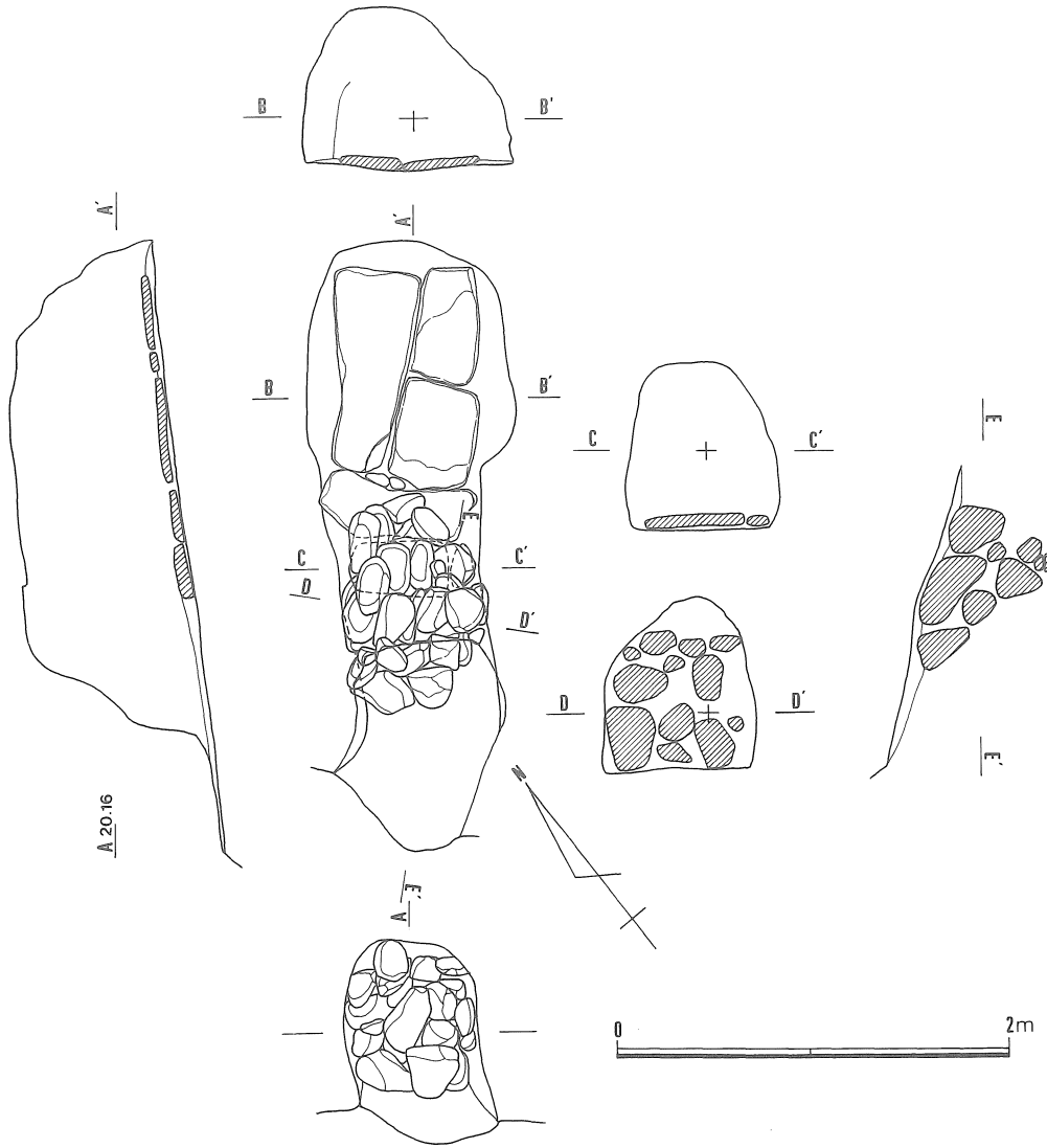
第9図 3号横穴実測図
