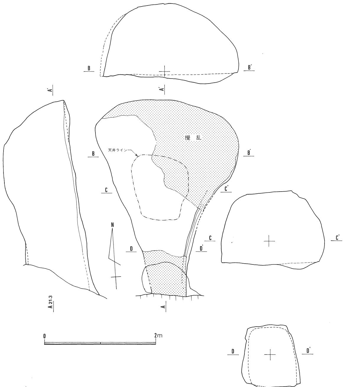
第7図 2号横穴実測図
