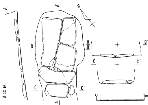
第10図 3号横穴棺床実測図
