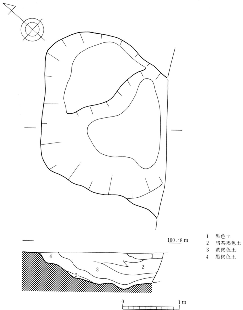
第10図 第3号土坑実測図 (1/40)
