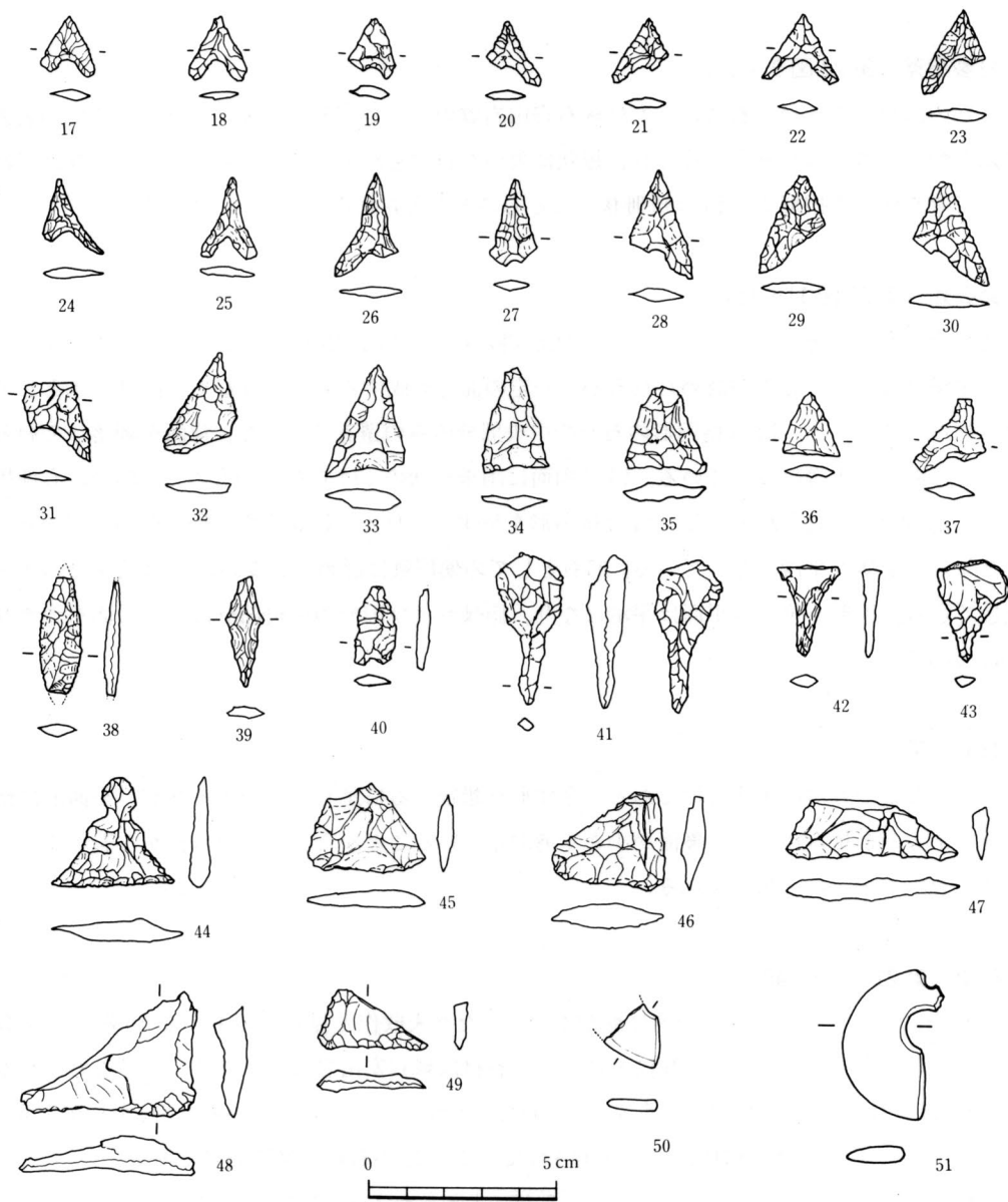
第21図 石器実測図(2) (S = 1/2)
