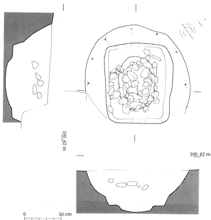
第11図 第1号土坑実測図 (1/30)
