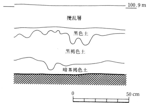
第5図 土層断面図 (3G) (1/20)
