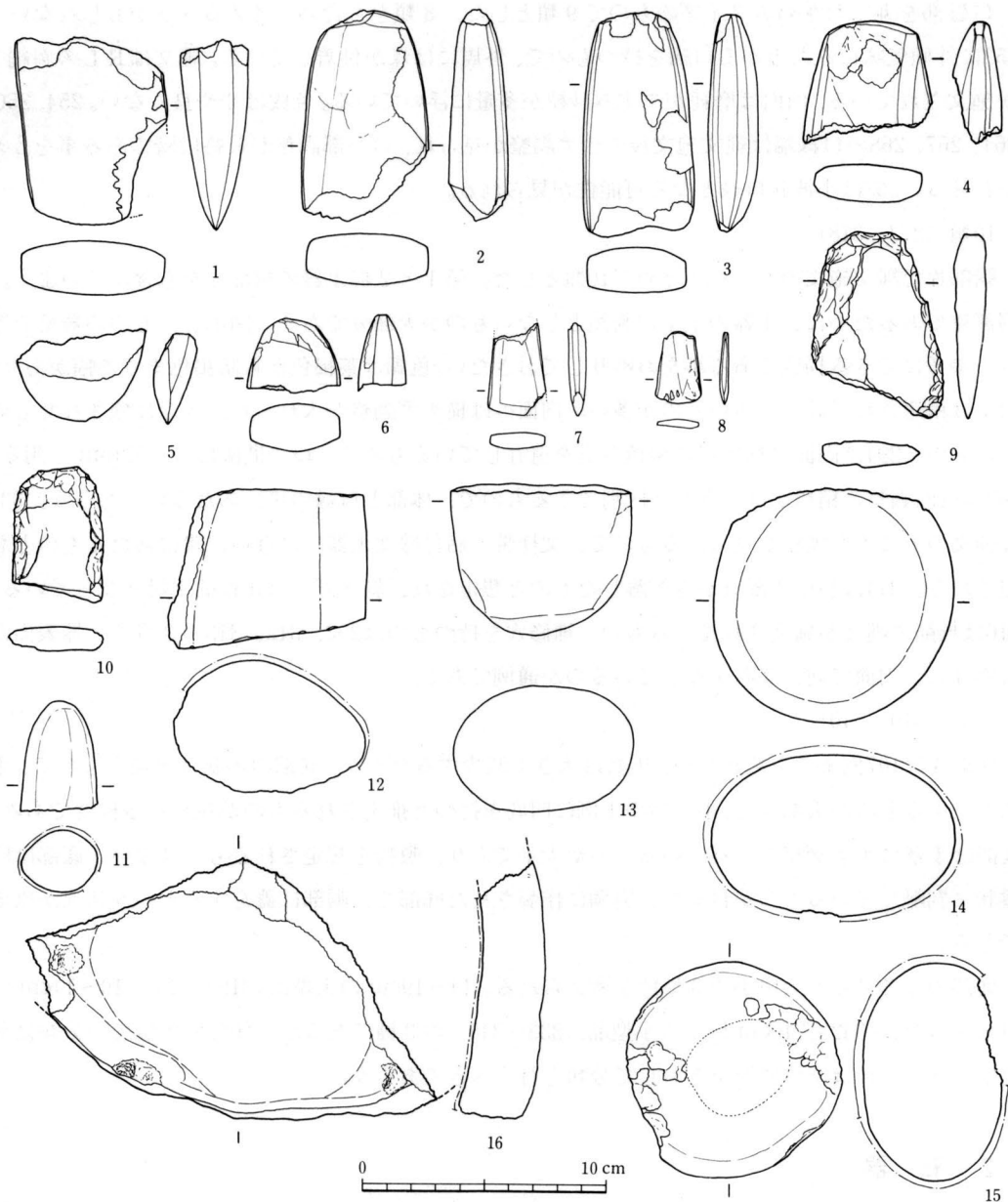
第20図 石器実測図(1) (S = 1/3)
