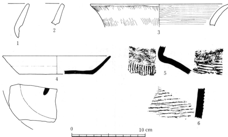
第22図 須恵器、土師器実測図 (S = 1/3)
