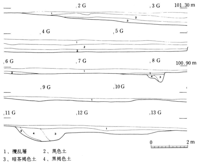
第4図 土層断面図 (1/80)
