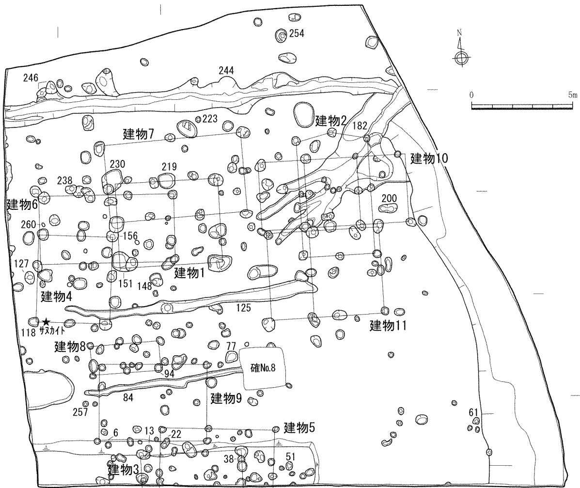
平面図
