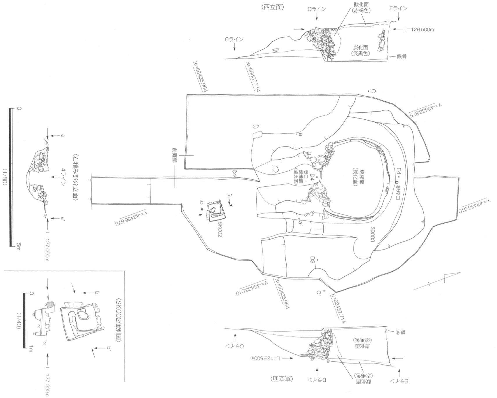
図5 SX001 木炭窯最終操業時遺構図 [図6に対応]
