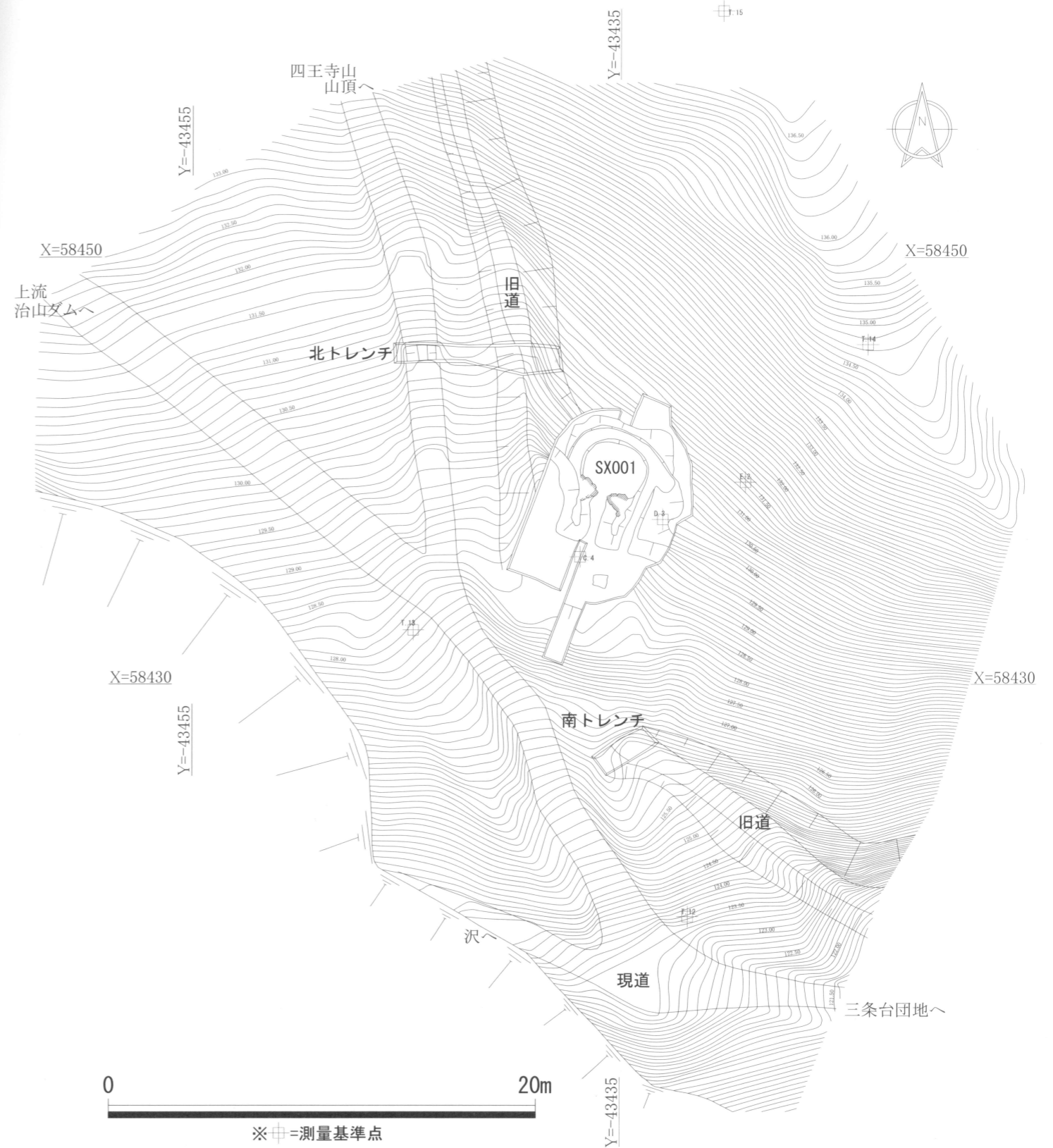
図4 調査地位置及び周辺地形測量図 (1/250)
