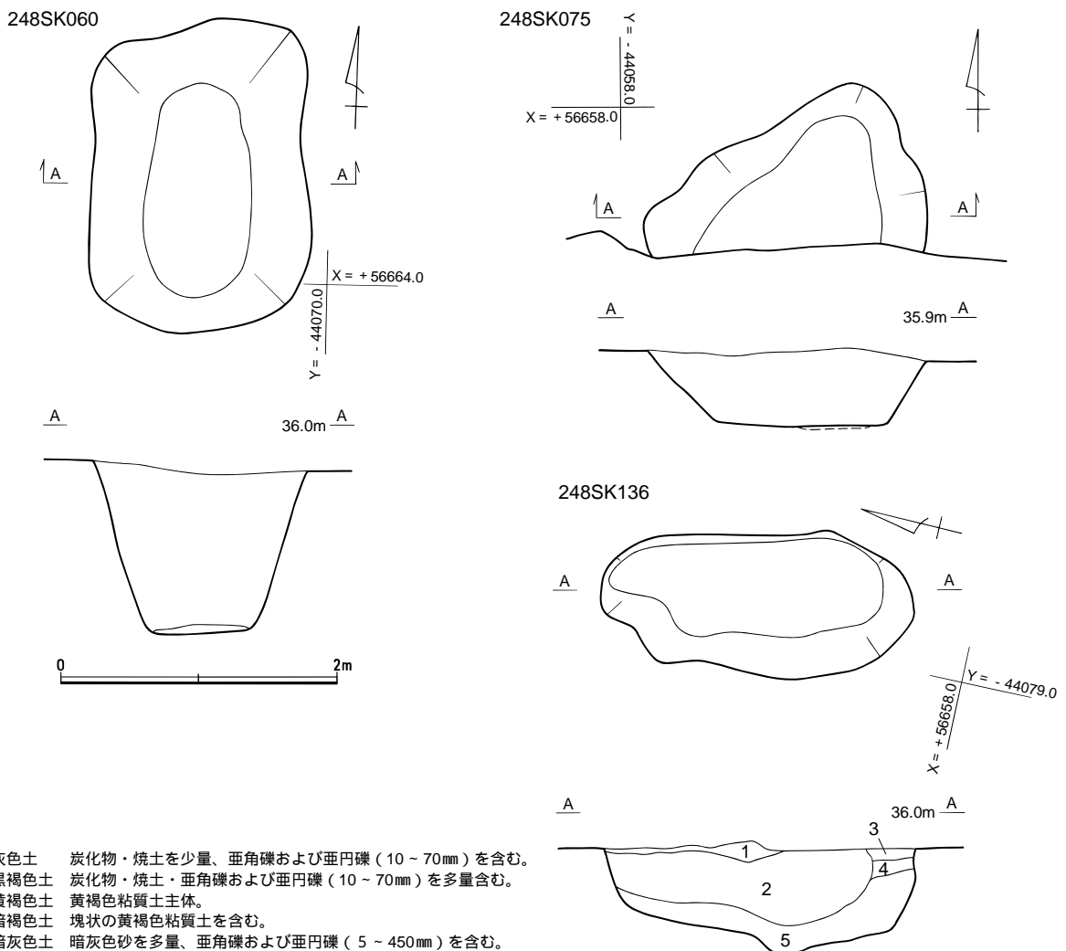
第14図 248SK060・075・136実測図(1/50)
