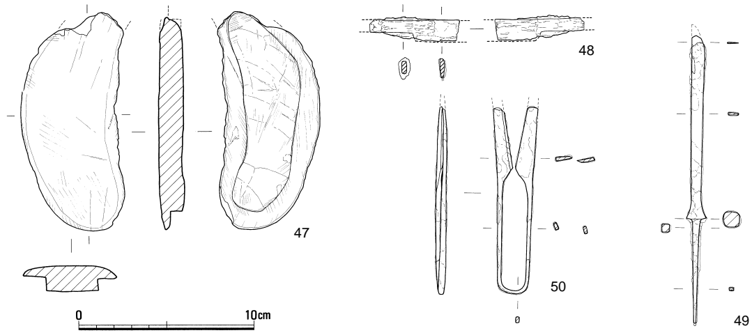
第64図 暗灰色土遺物実測図その3(1/3)
