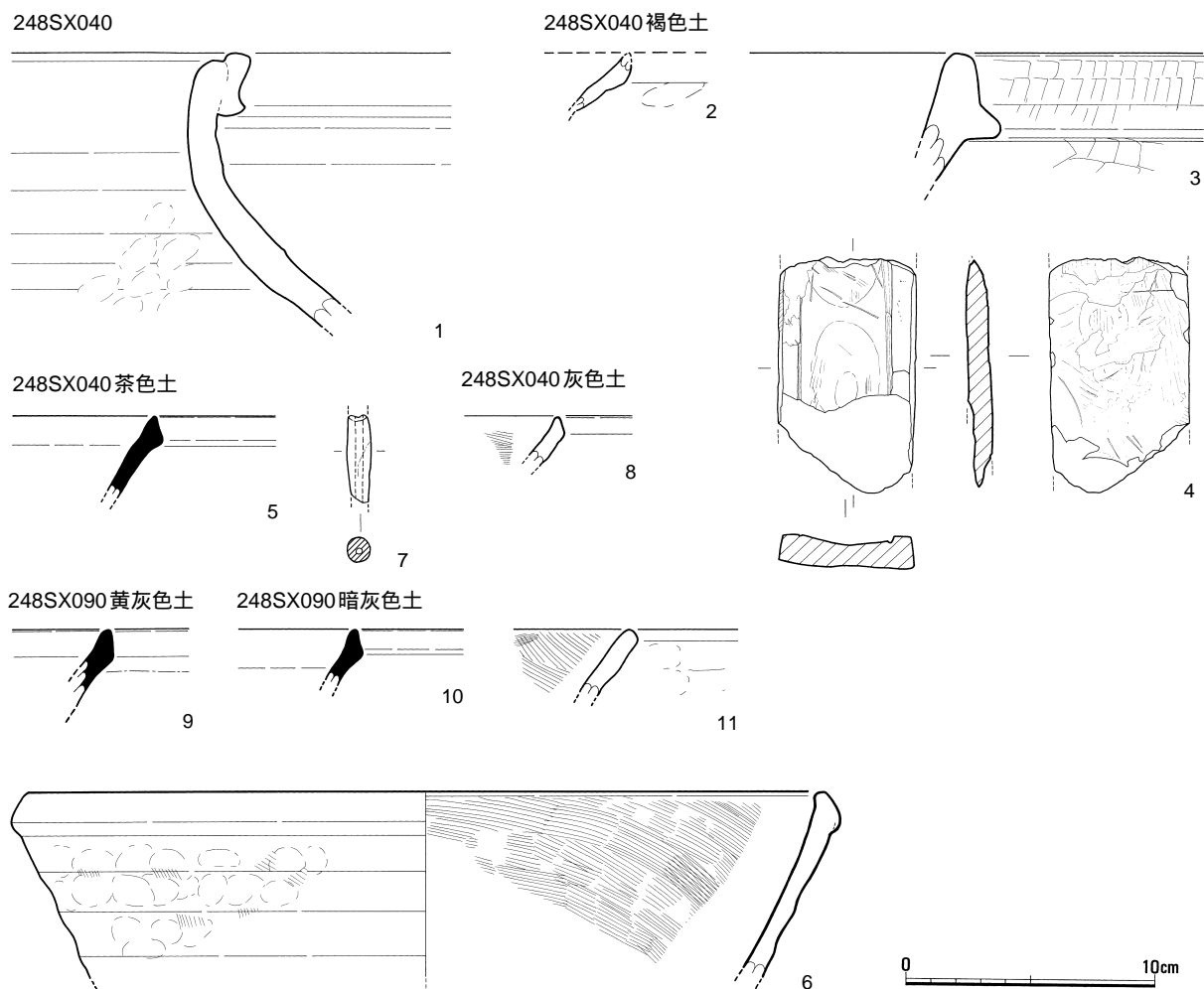
第37図 248SX040・090遺物実測図（1/3）
