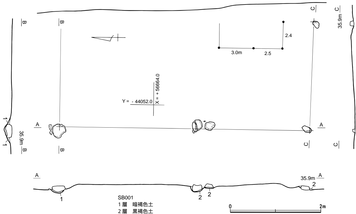
第9図 248SB001実測図(1/50)
