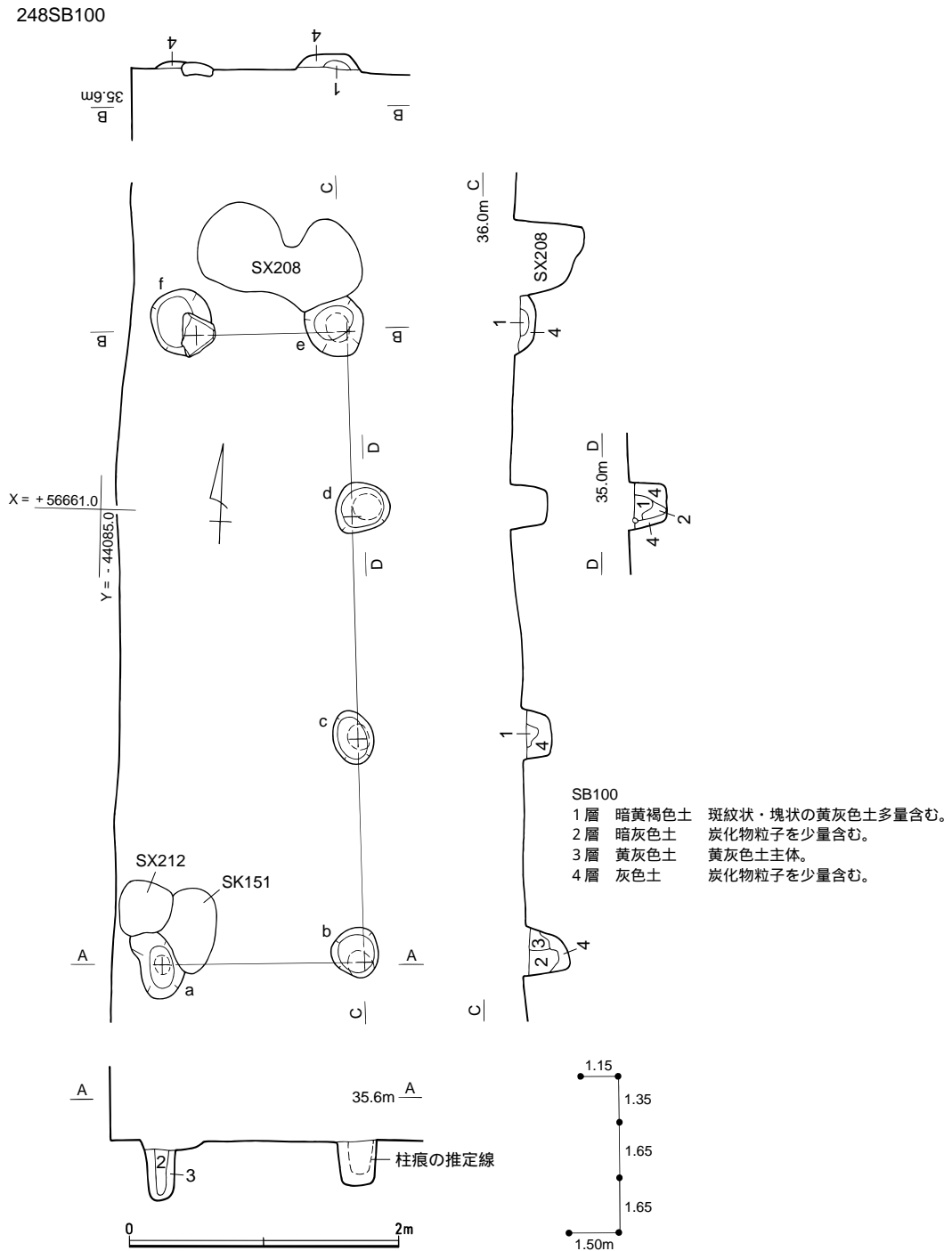
第18図 248SB100実測図(1/50)
