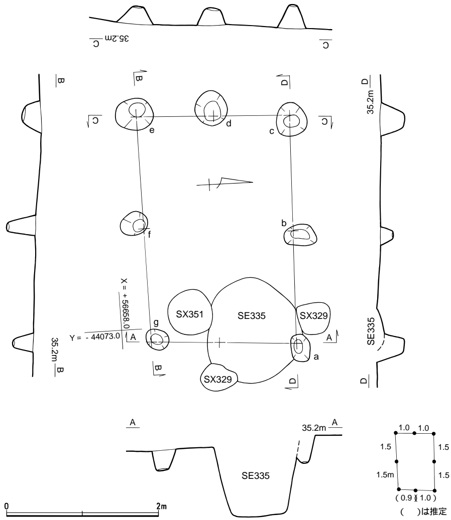
第28図 248SB406実測図(1/50)
