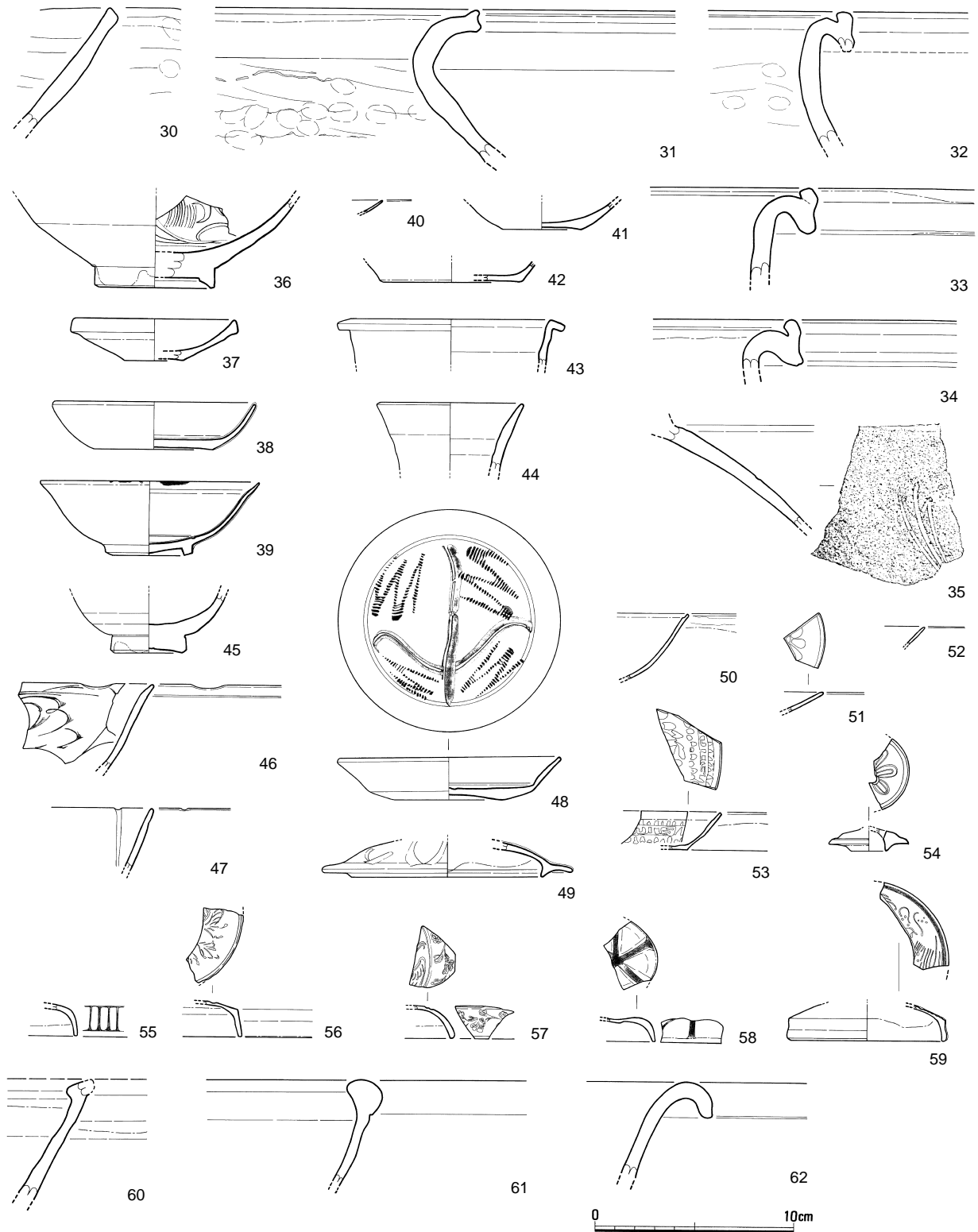
第60図 黄褐色土 2 遺物実測図その2(1/3)
