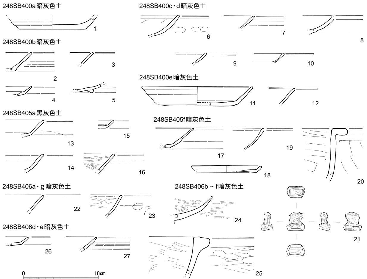
第53図 248SB400・405・406遺物実測図（1/3）
