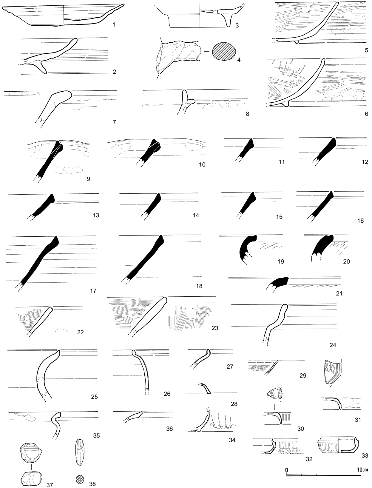
第62図 暗灰色土遺物実測図その1(1/3)
