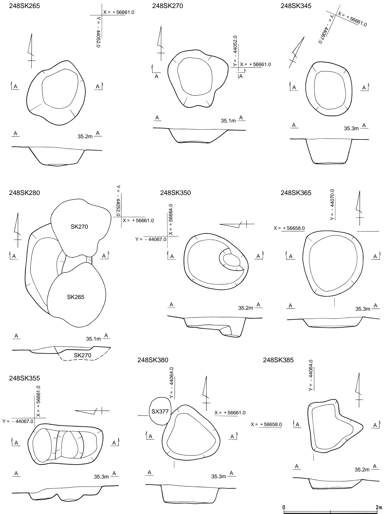
第32图 248SK265 · 270 · 280 · 345 · 350 · 355 · 365 · 380 · 385实测图 (1/50)
