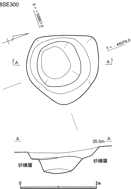
第31図 248SE290・295・300・335実測図(1/50)
