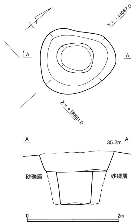
第30図 248SE360実測図(1/50)
