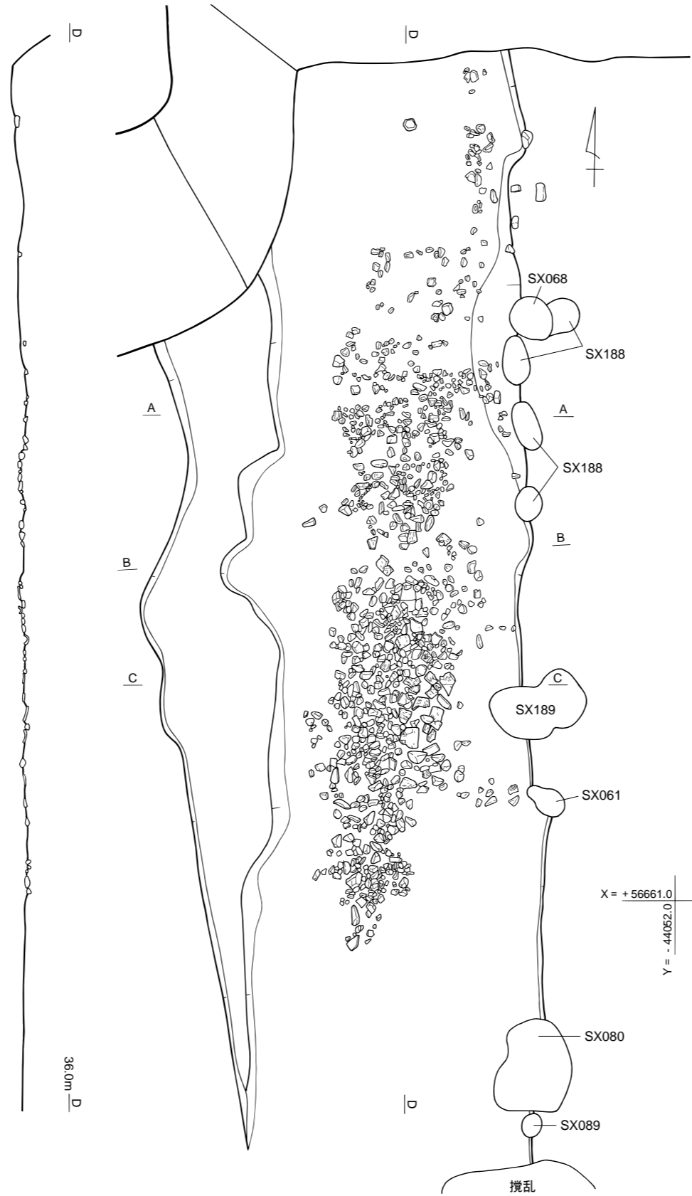
第10図 248SF035実測図(1/50)
