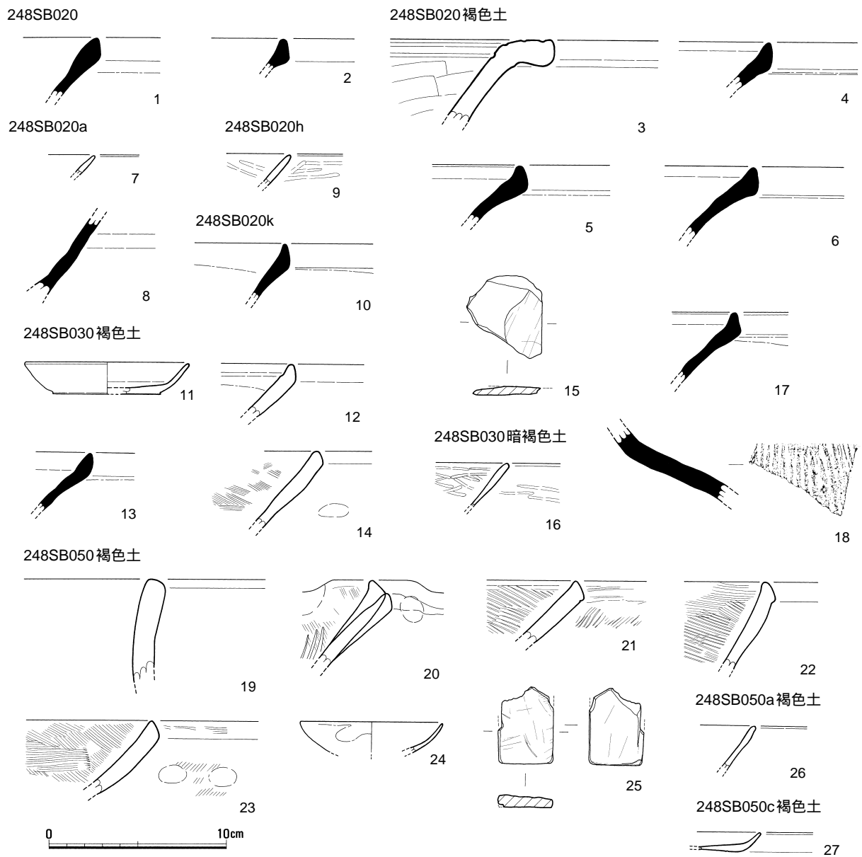
第35図 248SB020・030・050遺物実測図(1/3)
