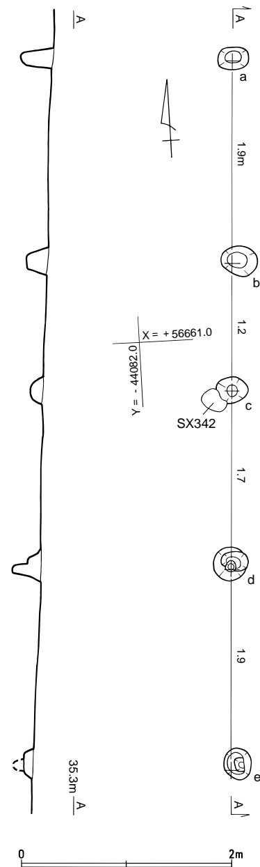
第25図 248SA255実測図(1/50)
