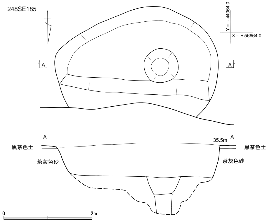
第21図 248SE180・185・195実測図(1/50)
