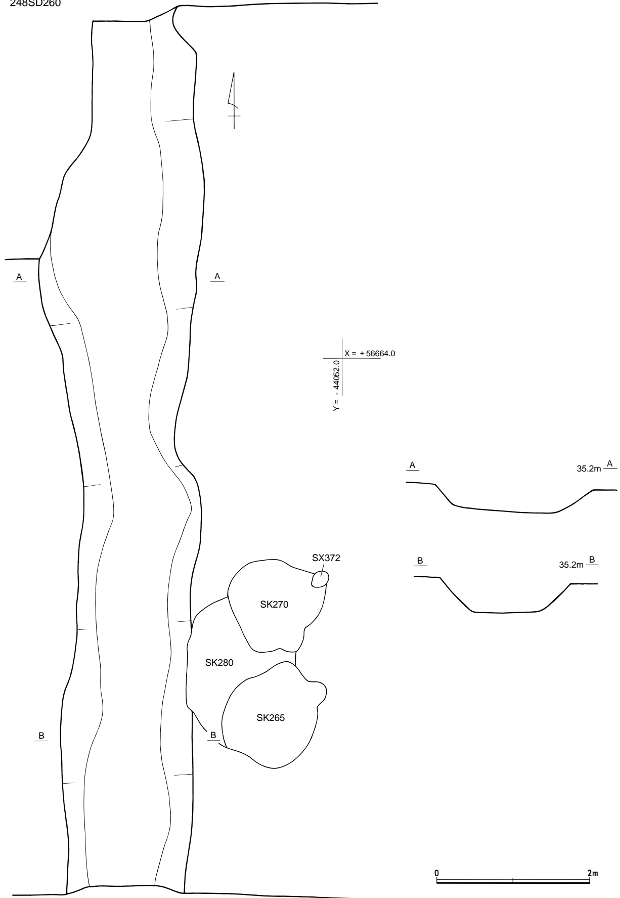
第29図 248SD260実測図(1/50)
