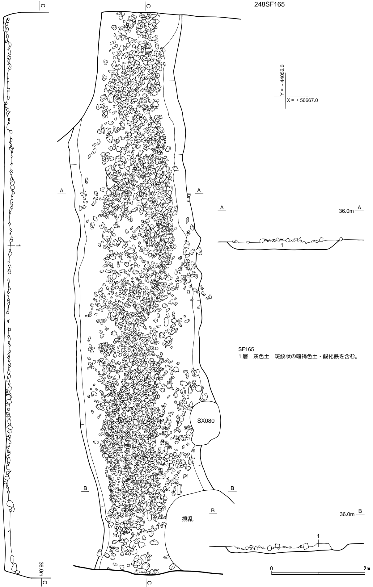
第16図 248SF165実測図(1/50)
