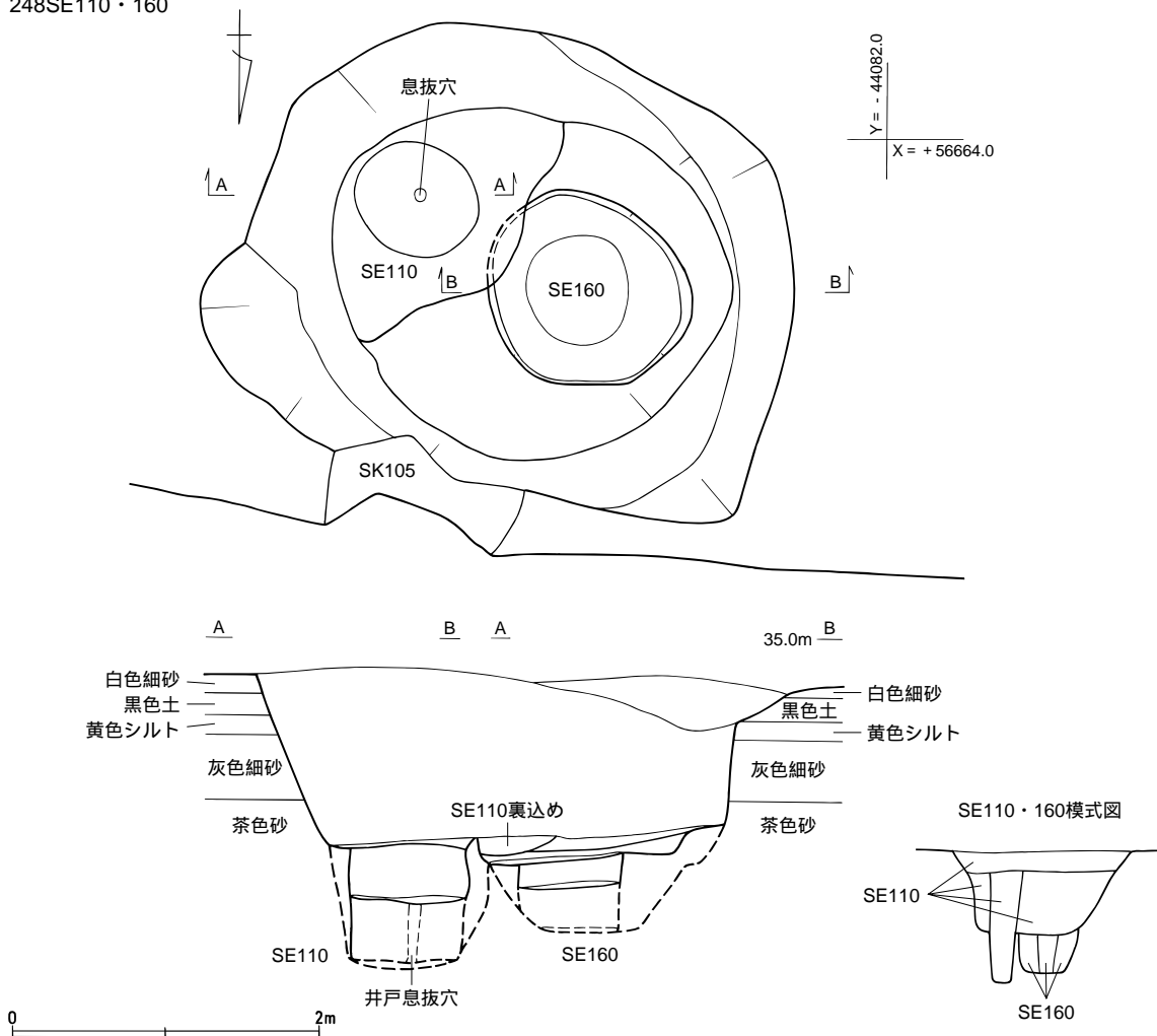
第19図 248SE110・160実測図(1/50)
