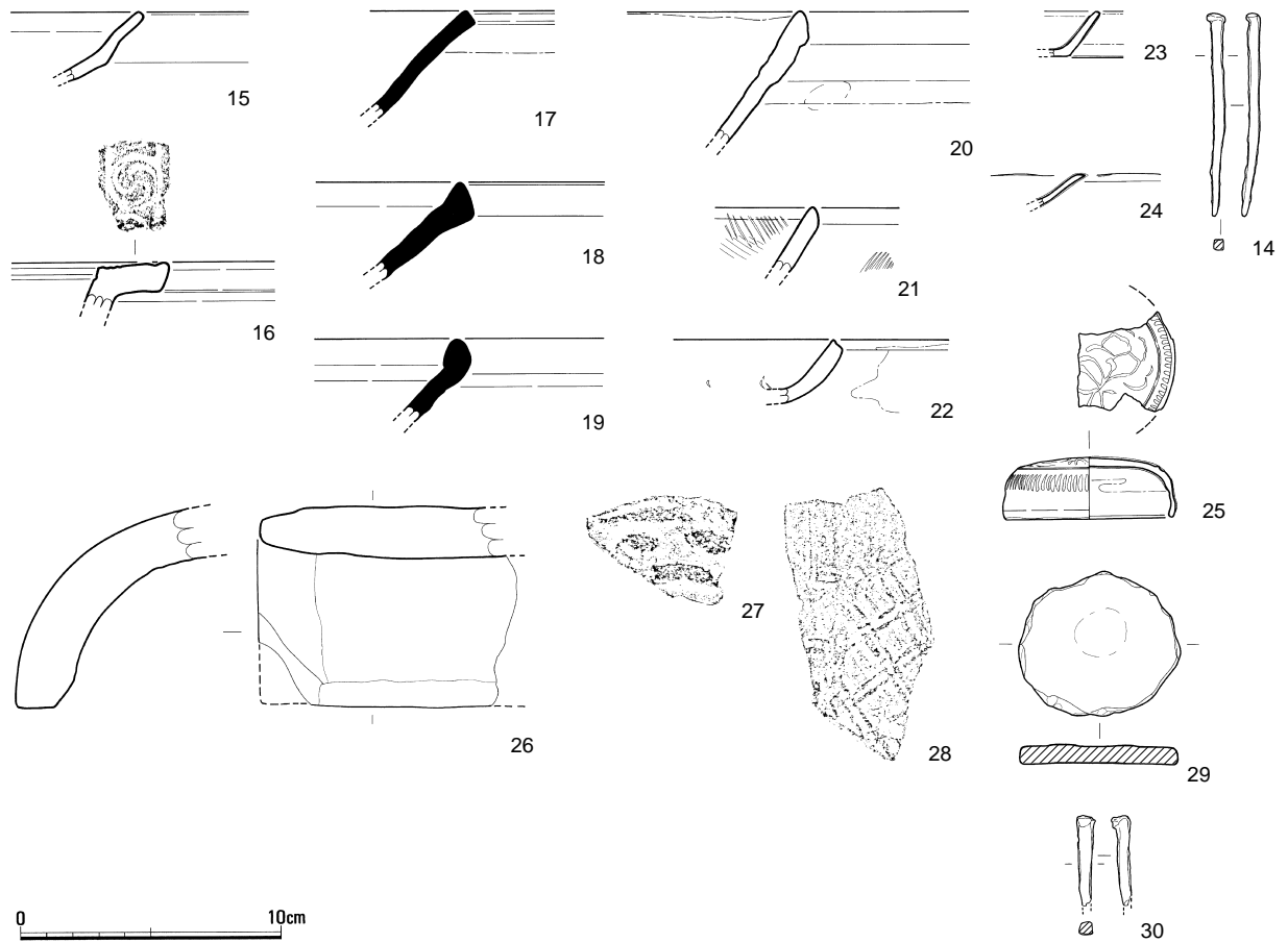
第46图 248SE110遺物実測図(1/3)
