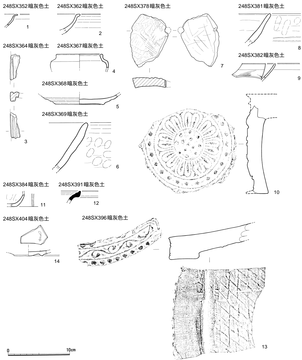
第57图 248SX352 · 362 · 364 · 367 · 368 · 369 · 378 · 381 · 382 · 384 · 391 · 396 · 404 遺物実測図 (1/3)
