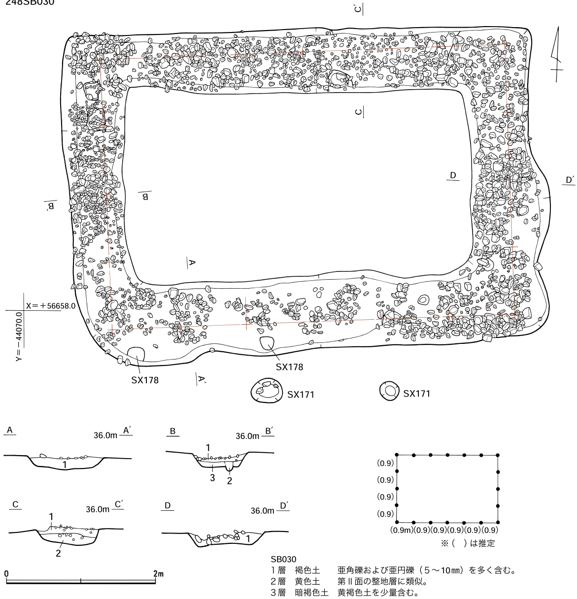
第12図 248SB030実測図（1/50）
