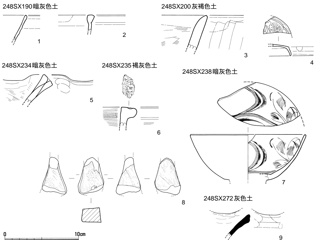
第51図 248SX190・200・234・235・238・272遺物実測図(1/3)
