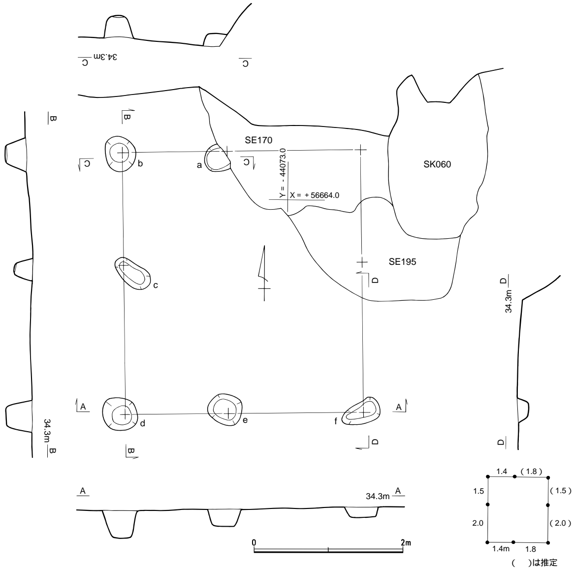
第27図 248SB405実測図(1/50)
