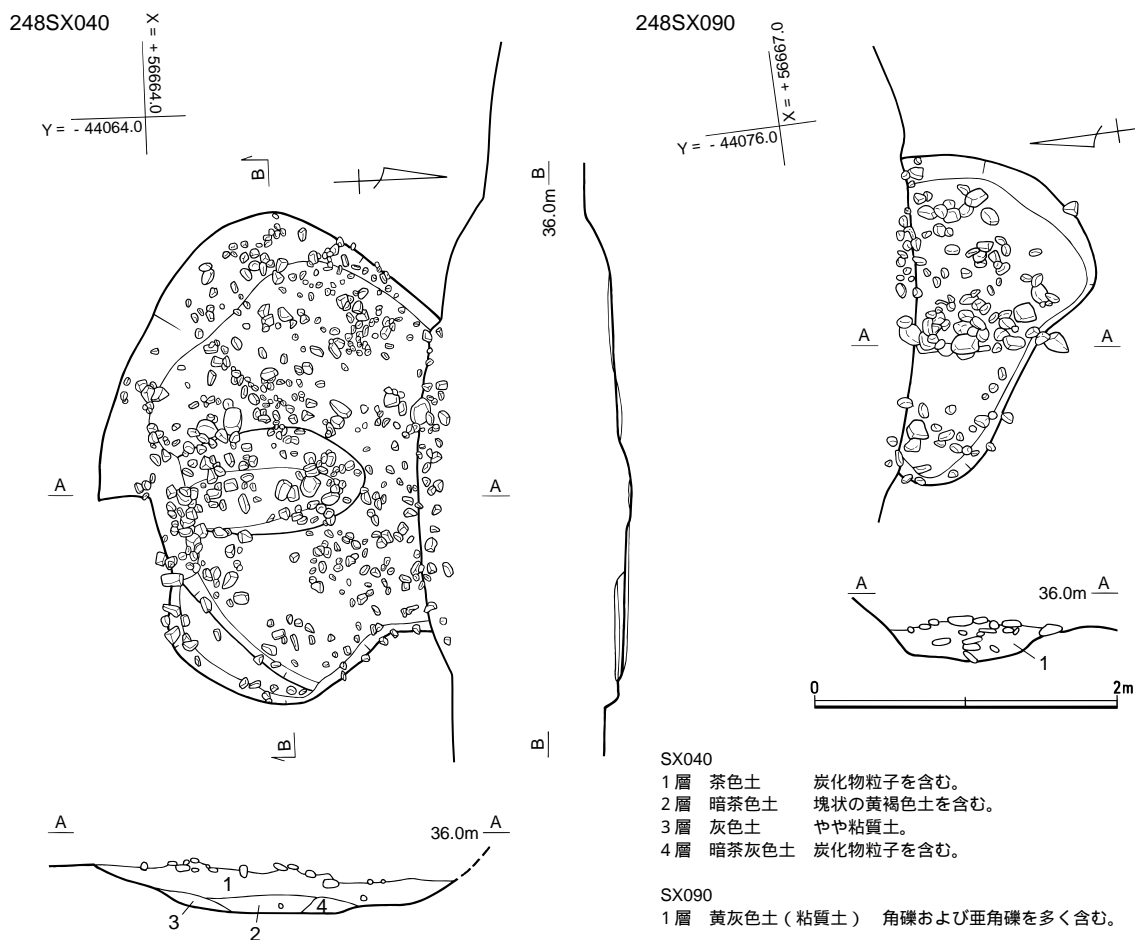
第15図 248SX040・090実測図(1/50)
