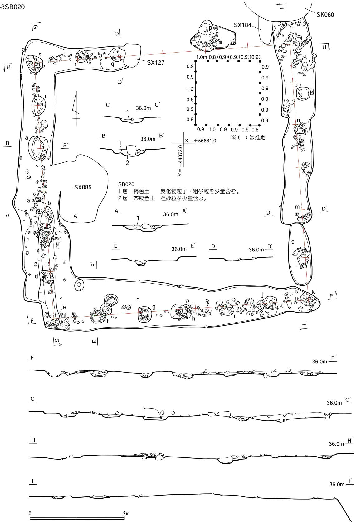
第11図 248SB020実測図 (1/50)
