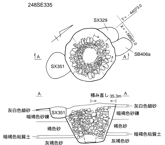
第31図 248SE290・295・300・335実測図(1/50)
