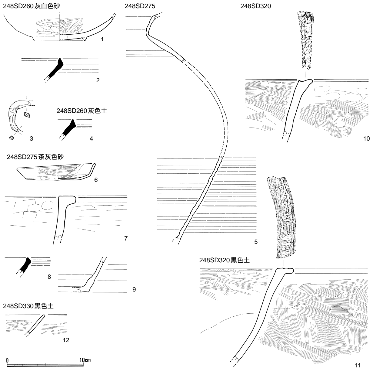
第54図 248SD260・275・320・330遺物実測図（1/3）
