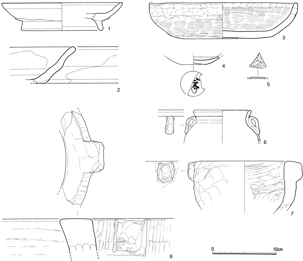
第65図 黄灰色土遺物実測図(1/3)
