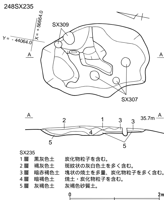
第24図 248SX235実測図(1/50)
