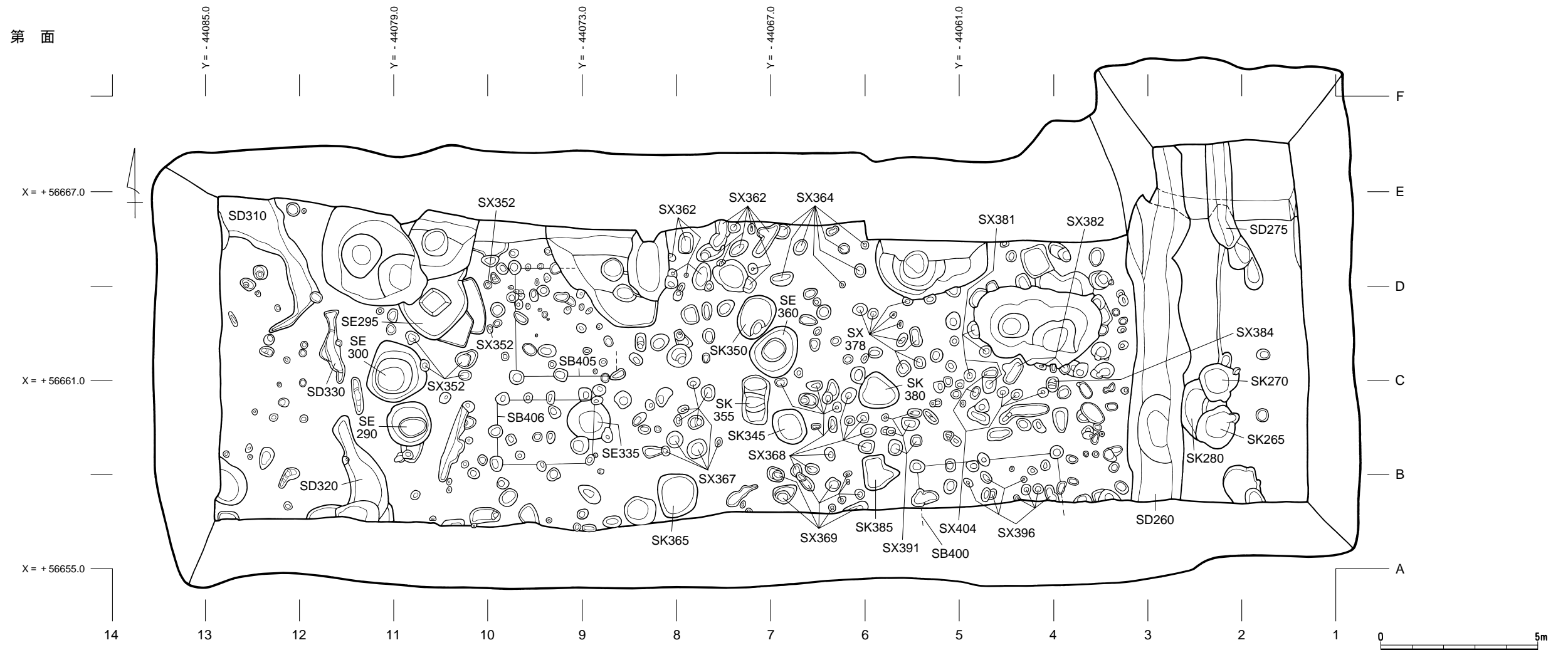
第 6 図 大宰府条坊跡第 248 次調査第 面遺構全体図 ( 1 / 150 )
