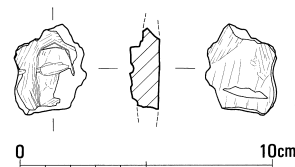
第38図 248SX182 遺物実測図 (1/3)
