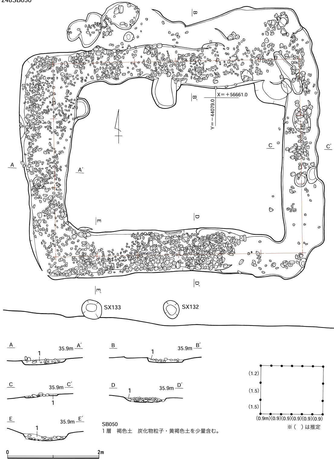
第13図 248SB050実測図 (1/50)
