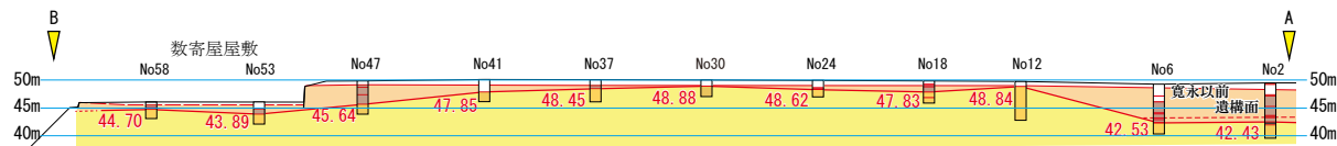
東西断面概略図
