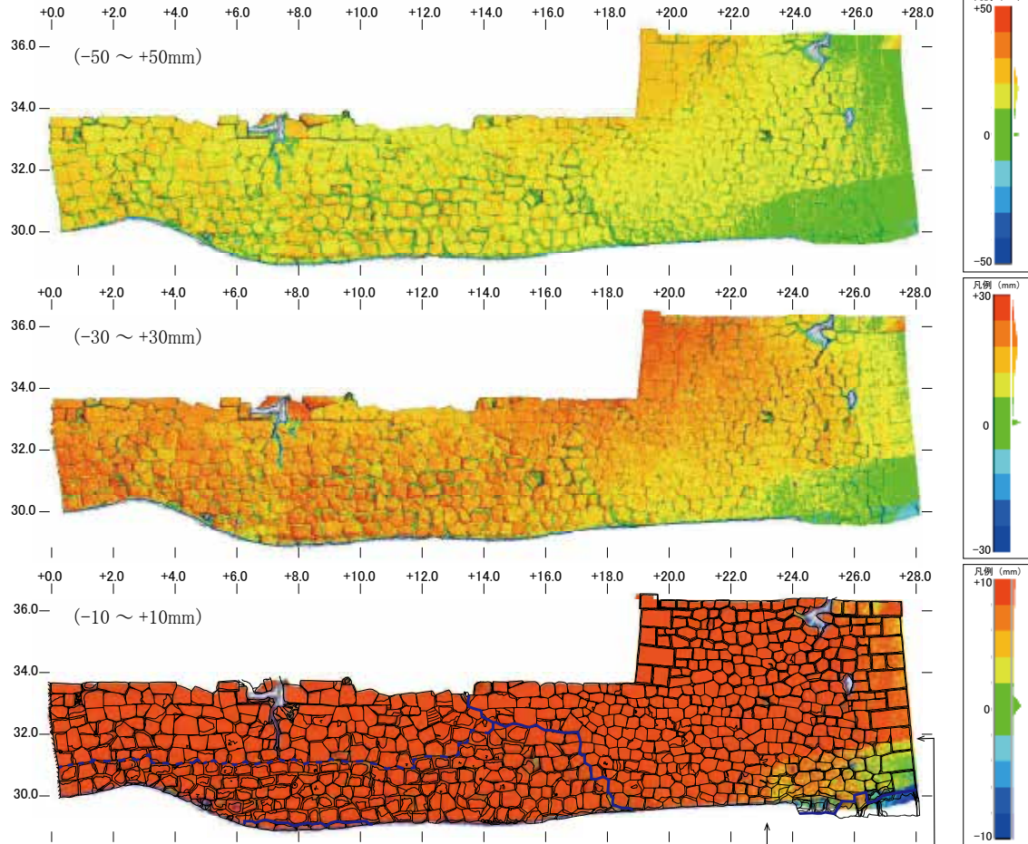
玉泉院丸北泉水縁石垣変形動態 計測誤差による色調変化が顕著となる
