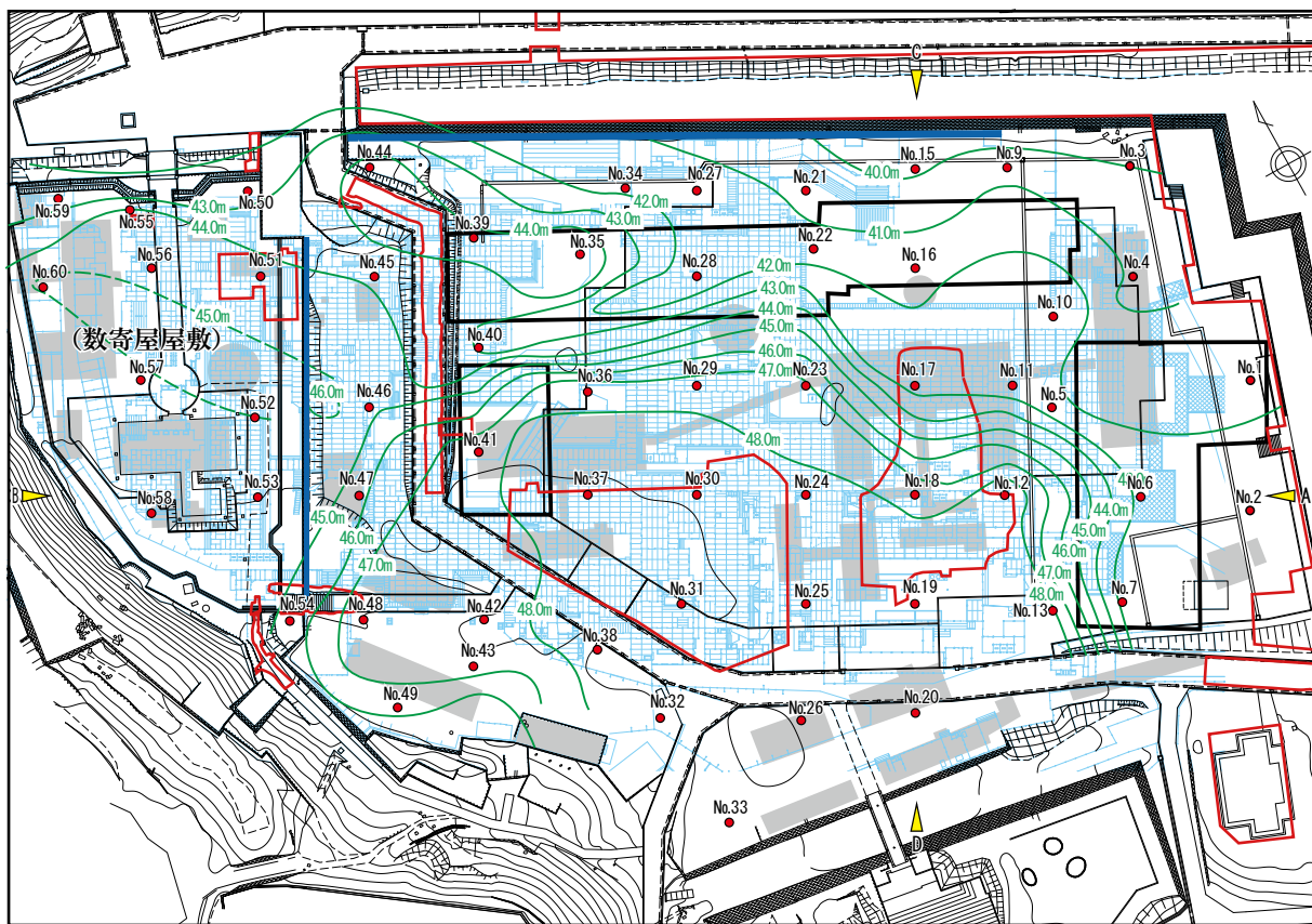
御殿絵図 軍隊建物 大学建物 過年度発掘 — 地山等高線 (推定) ● ボーリング地点 石垣観察調査 0 1:1,500 50m
