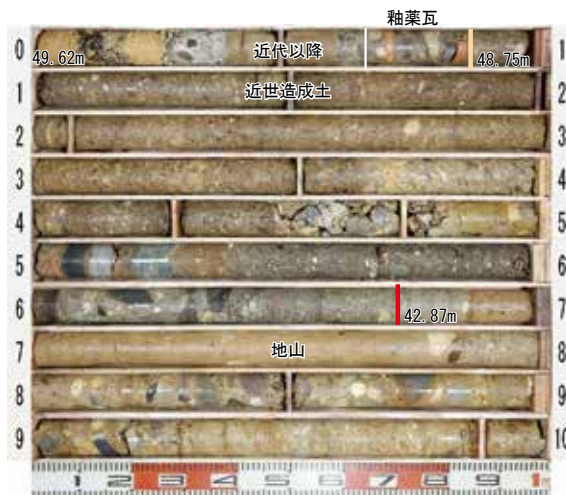
No. 10ボーリングコア写真
