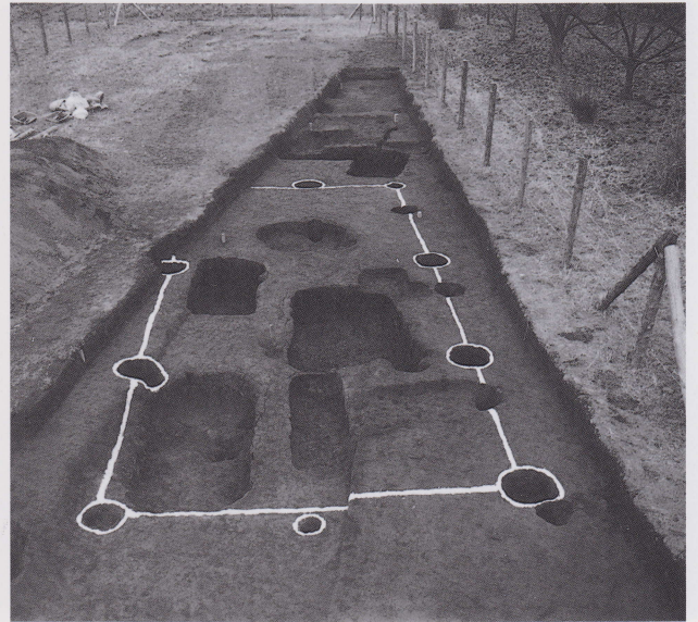
第2号掘立柱建物跡
