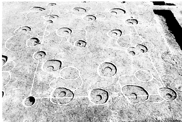
第38号掘立柱建物跡 確認状況
