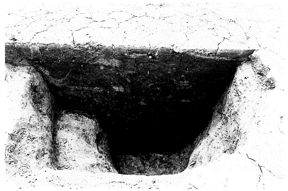
第63号掘立柱建物跡 ピットⅠ断面
