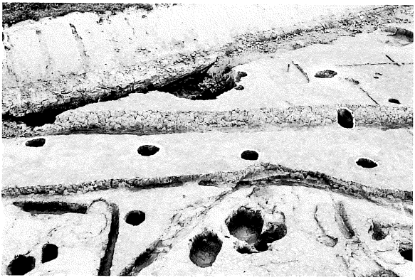
第65号掘立柱建物跡・第167・170号住居跡
