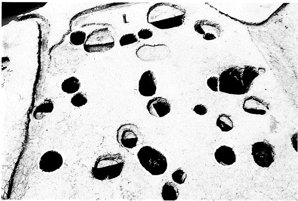
第72号掘立柱建物跡・第84号井戸跡
