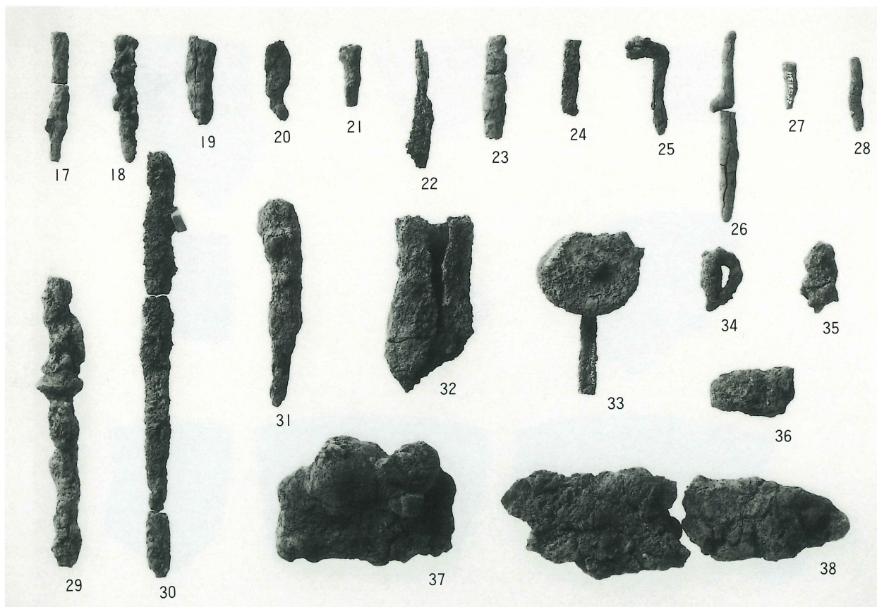
I 区出土鉄製品 第249図
