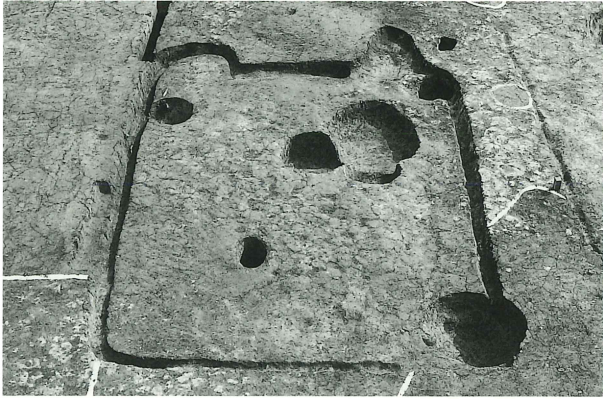
II区第114号住居跡
