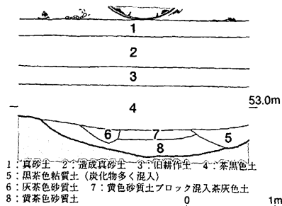
図6 1SD015南壁土層実測図 (S=1/60)
