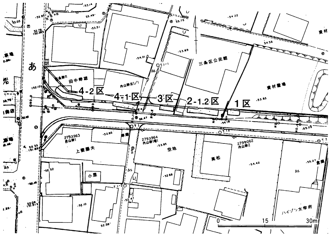
図3.トレンチ設定図 (S=1/750)
