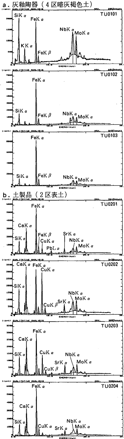
図8 蛍光X線分析による元素のenergy-peak
