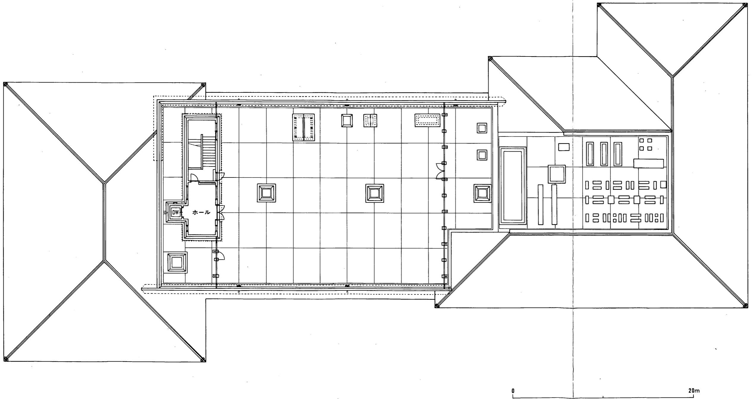
第8図 太宰府市文化ふれあい館 屋上平面図 (1/250)
