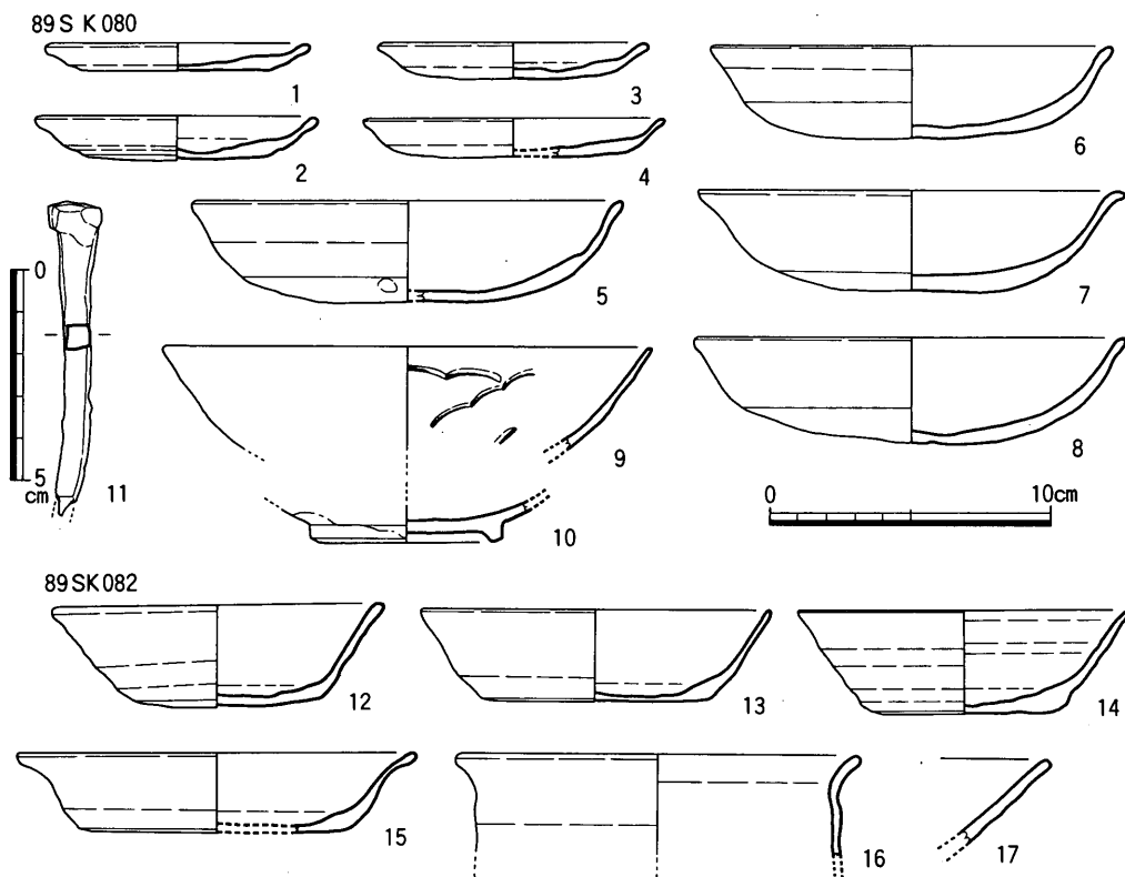
Fig.110 89SK080・082出土遺物実測図(1/3・1/2)
