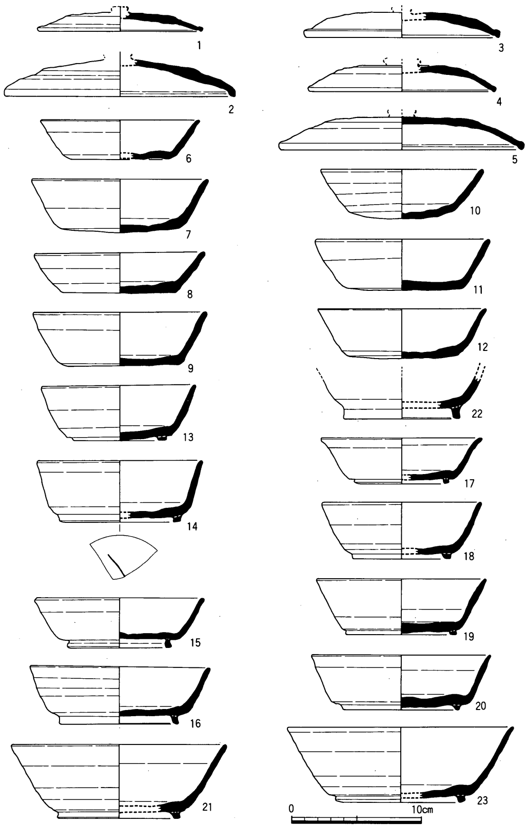
Fig. 52 81SK135出土遺物実測図(1)(1/3)
