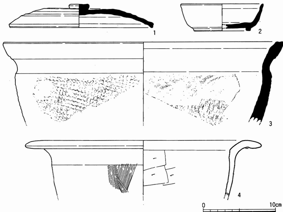
Fig.122 89SX049出土遺物実測図(1/3)
