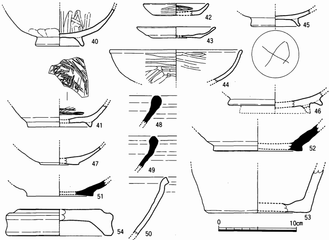
Fig. 80 茶褐色土出土遺物実測図(2)(1/3)
