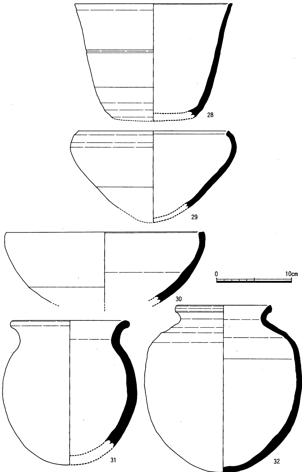
Fig. 49 81SK130出土遺物実測図(2)(1/3)
