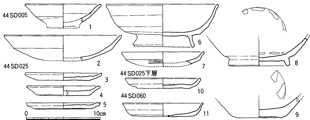
Fig. 5 第44次調査溝出土遺物実測図(1/3)
