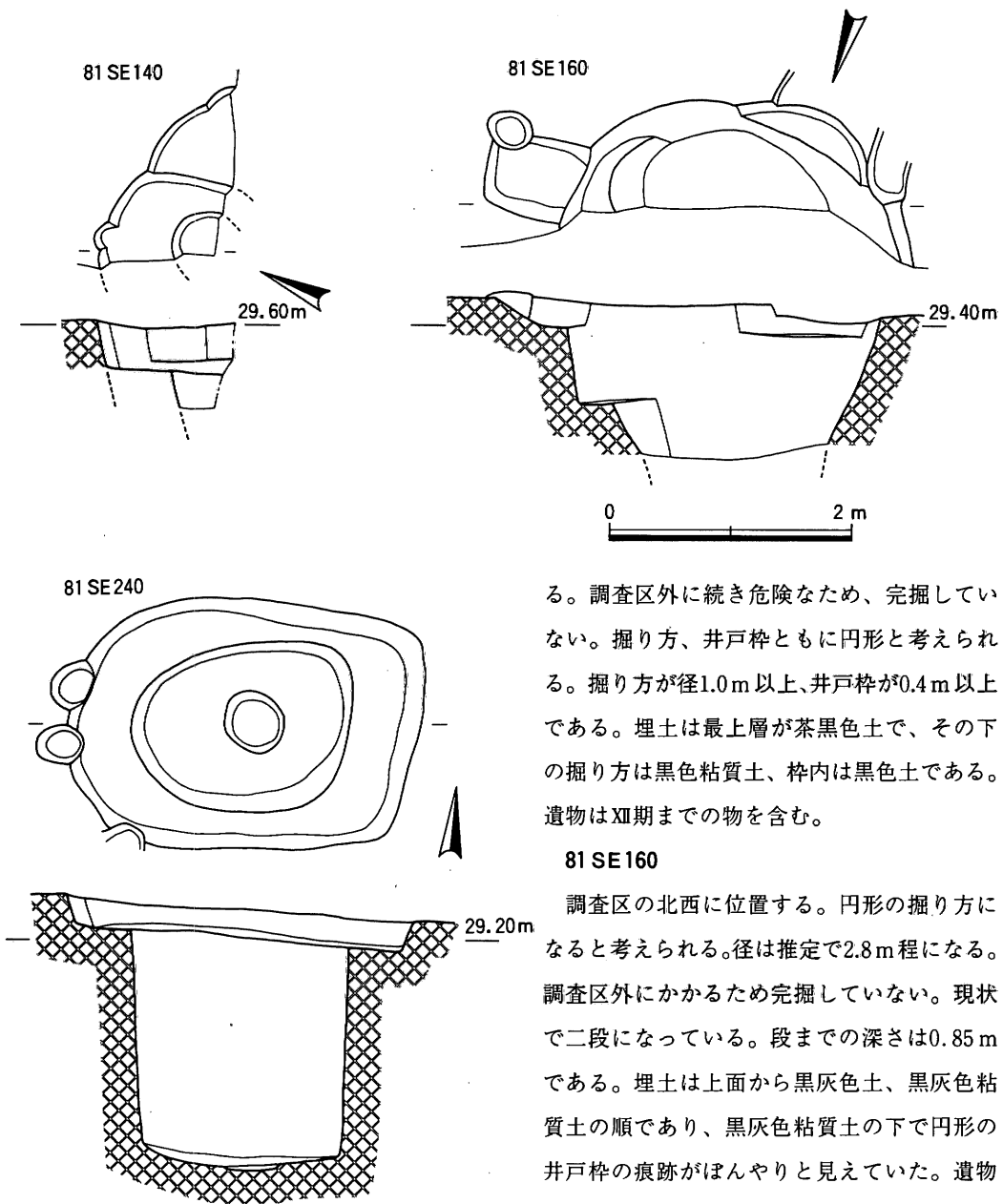
Fig. 37 第81次調査井戸実測図(2)(1/60)
