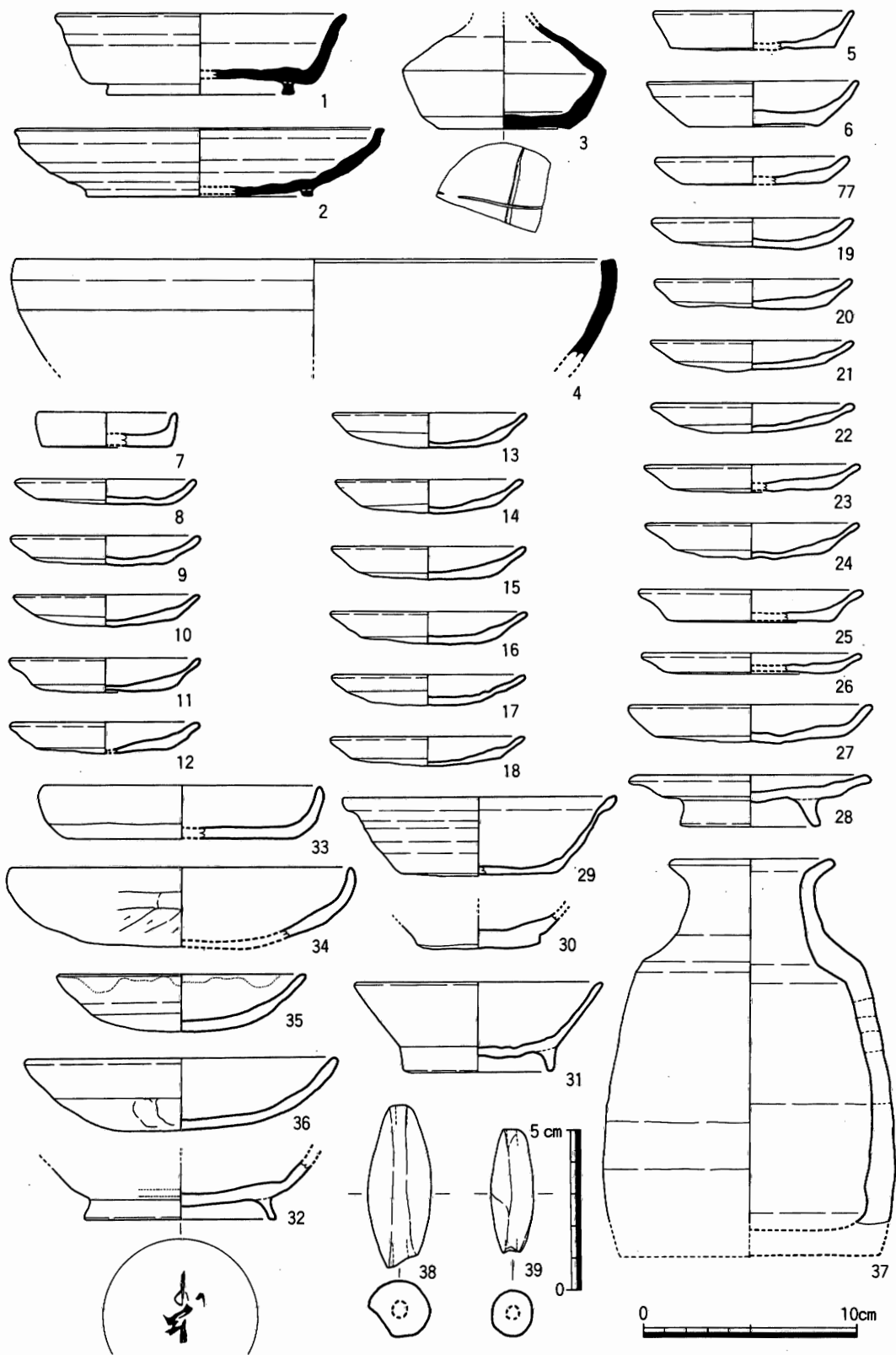
Fig. 79 茶褐色土出土遺物実測図(1)(1/3・1/2)
