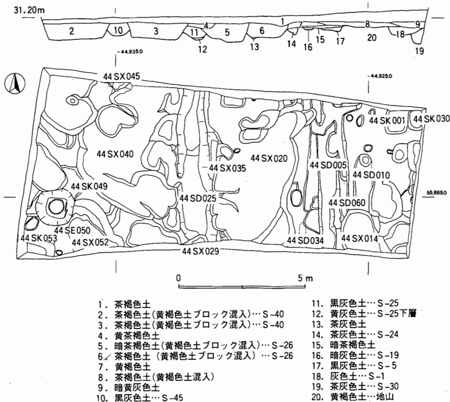
Fig. 3 第44次調査遺構実測図(1/150)
