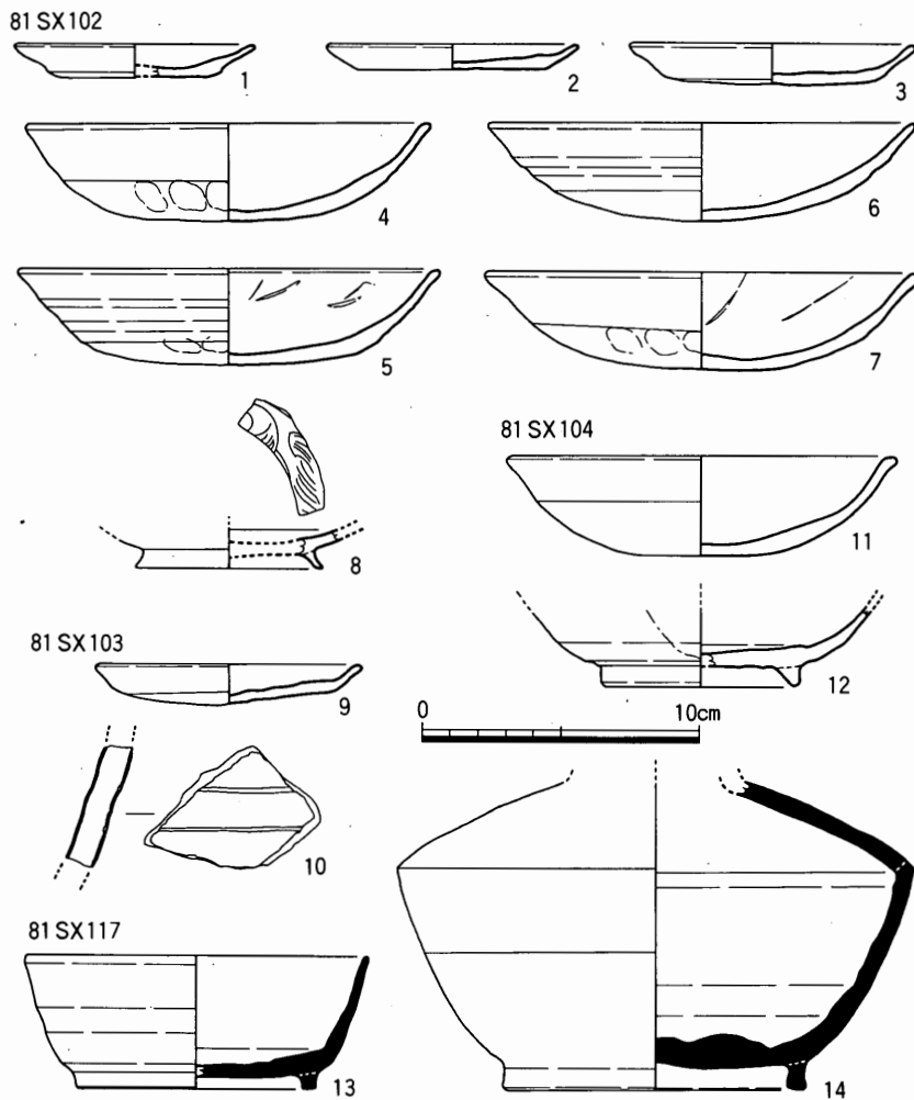
Fig.73 81 SX102・103・104・117出土遺物実測図(1/3)
