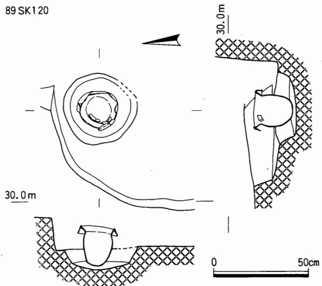
Fig.91 第89次調査土壌実測図(3)(1/20)
