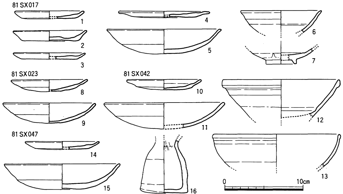
Fig. 69 81 SX017・023・042・047出土遺物実測図(1/3)
