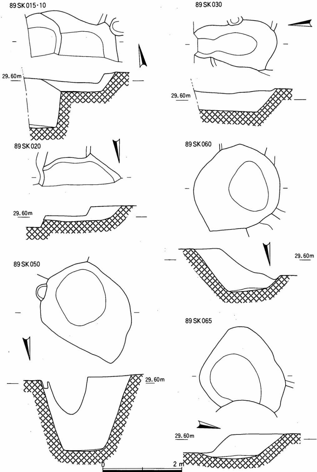
Fig. 89 第89次調査土壌実測図(1) (1/60)
