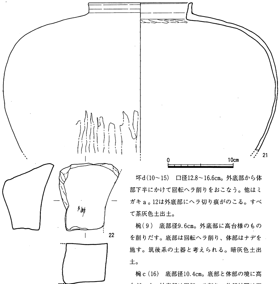
Fig. 61 81 SE060出土 遺物実測図(2)(1/3)
