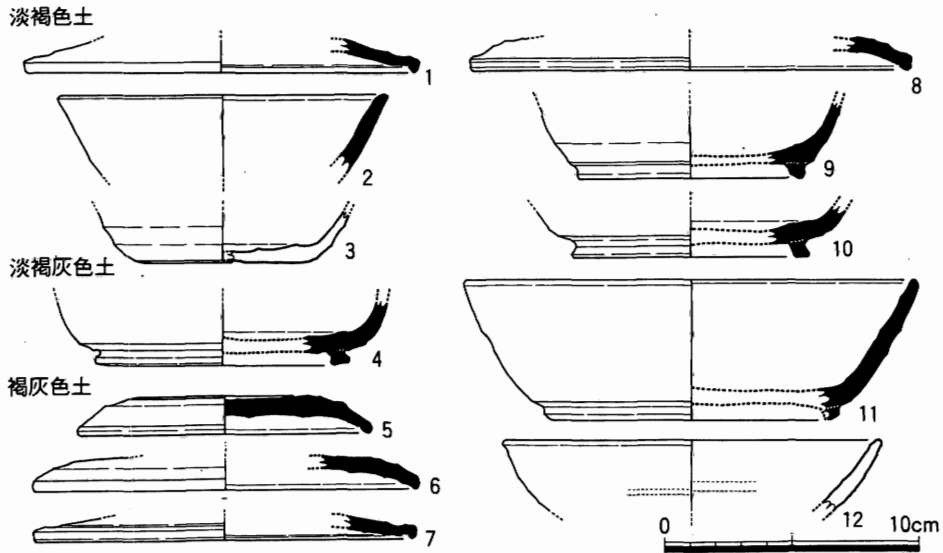
Fig. 32 第65次調査各層出土遺物実測図(1/3)
