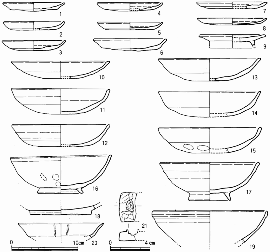
Fig.67 81SD110出土遺物実測図(1/3・1/2)
