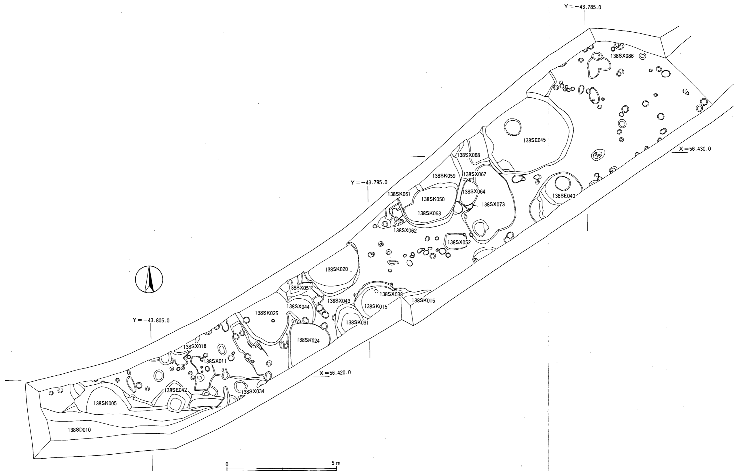
Fig. 6 大宰府条坊跡第138次調査遺構配置図
