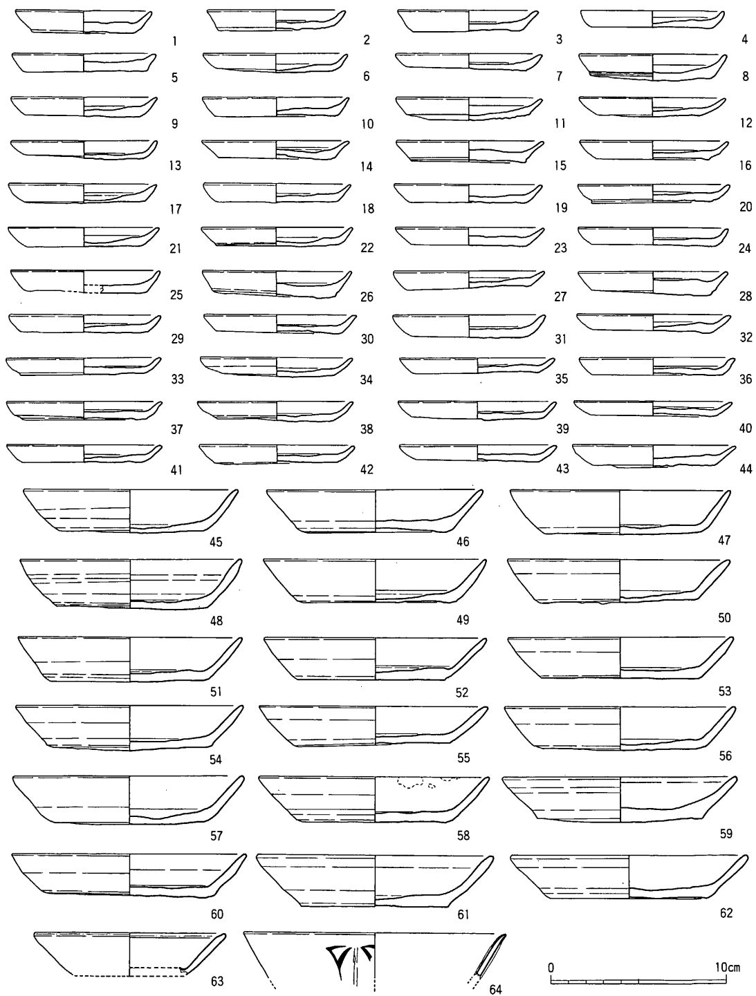
Fig. 19 138SK050炭層下層出土土器実測図
