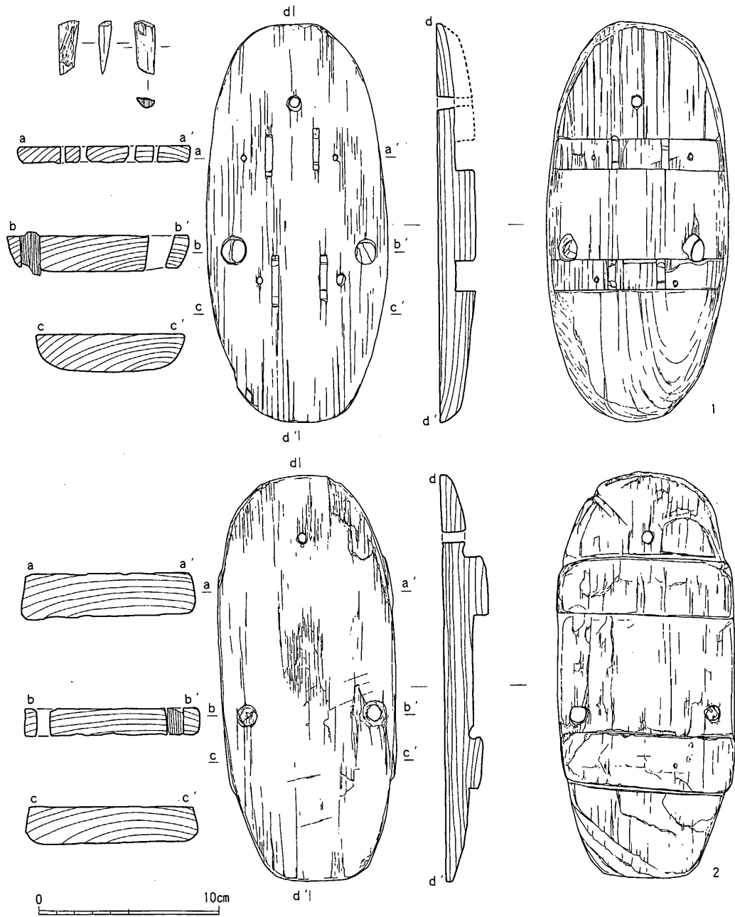
Fig. 24 138SK059出土木製品実測図 I
