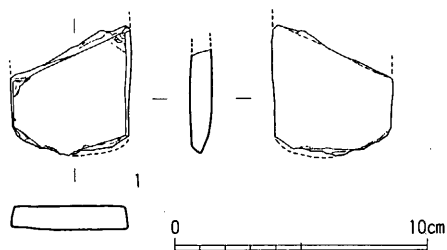
Fig. 27 石製品実測図
