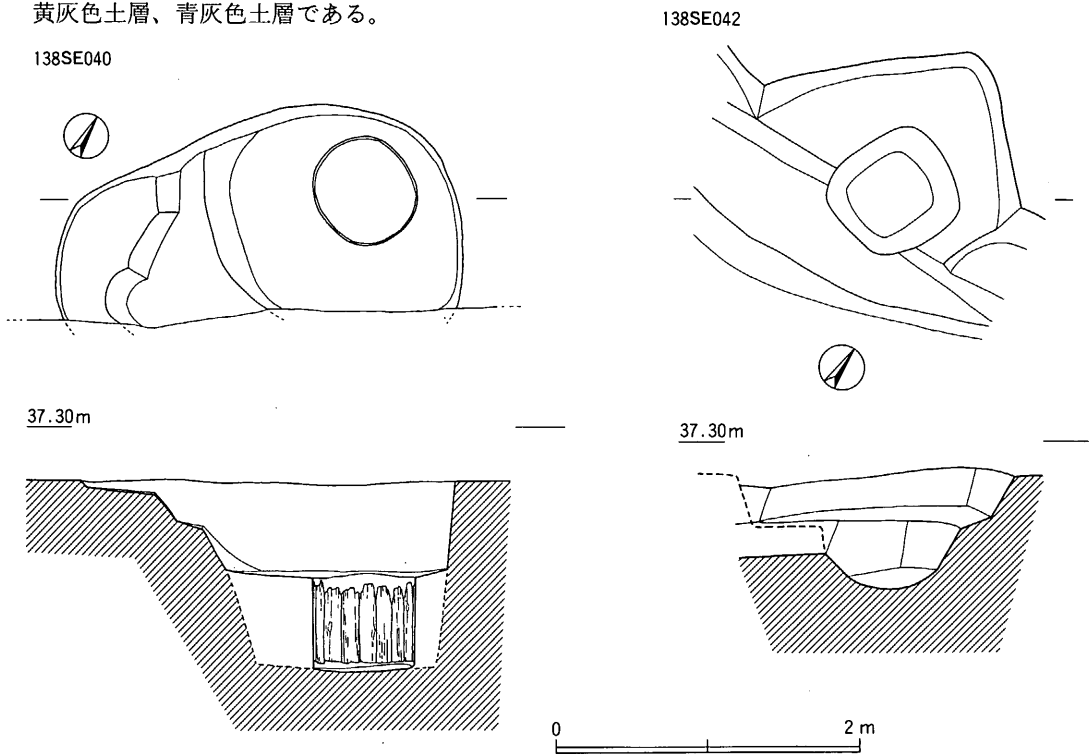
Fig. 9 138SE040・042実測図
