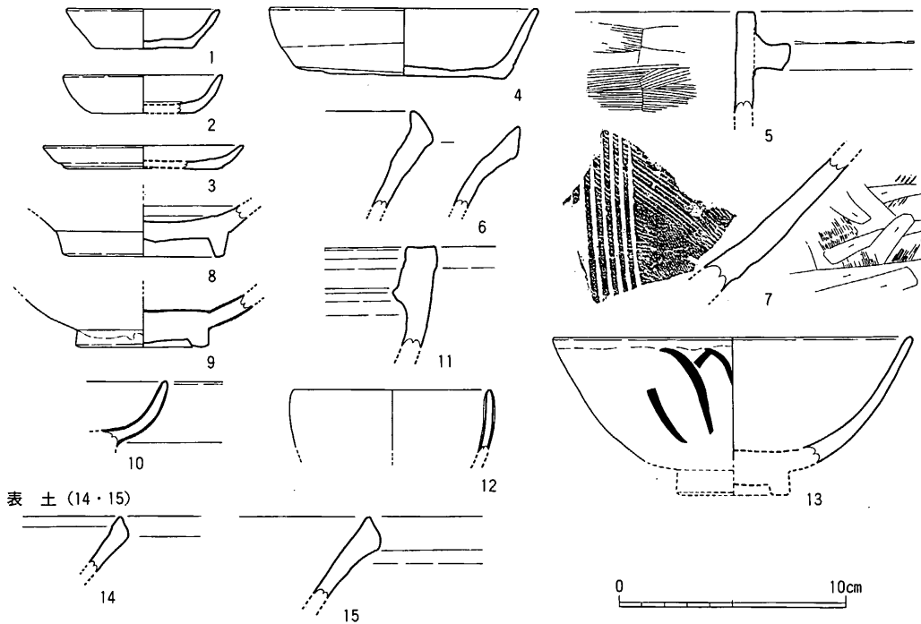
Fig. 23 茶色土層・表土出土土器実測図
