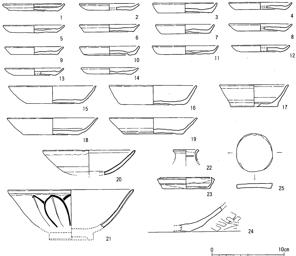
Fig.15 138SK015黒灰色土層出土土器実測図
