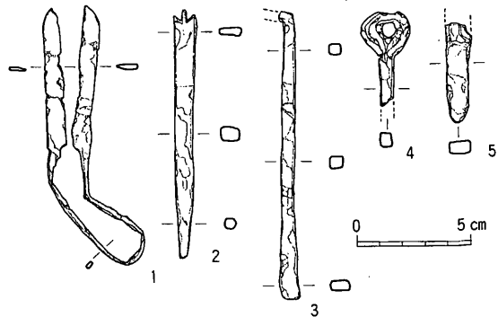
Fig.26 鉄製品実測図
