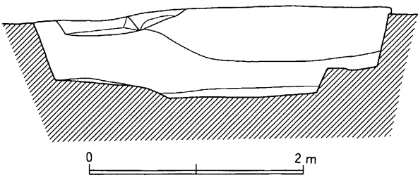
Fig. 8 138SK020・050実測図・土層観察図
