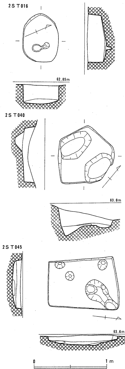
Fig.34 火葬施設実測図
