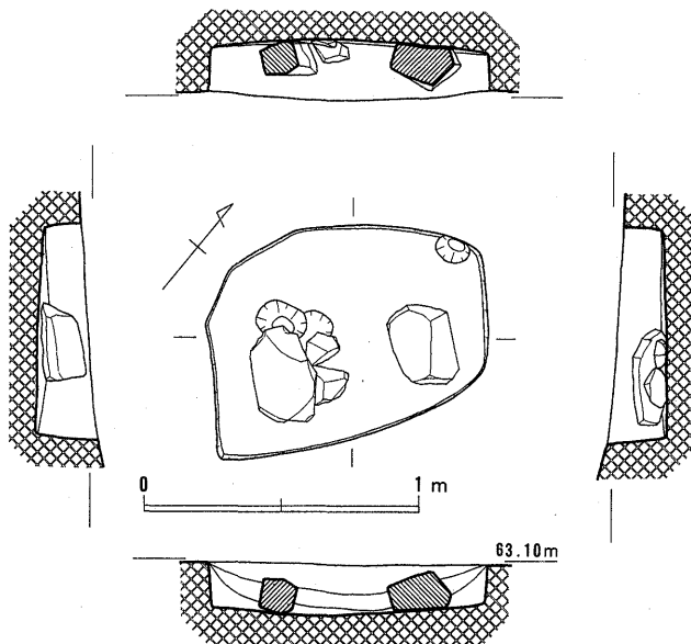
Fig.19 5号墓実測図
