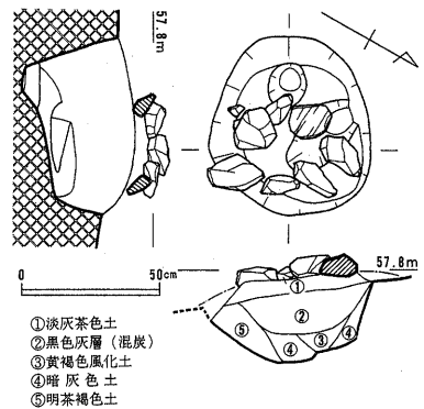
Fig.32 10号墓実測図
