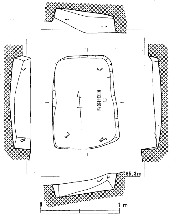
Fig.22 6号墓実測図
