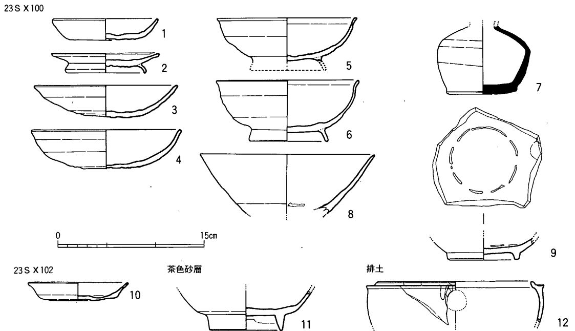
fig. 50 第23次調査出土土器実測図
