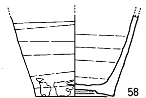
fig. 16 19SK004出土土器実測図 (Ⅶ)
