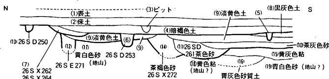
fig. 58 第26次調査土層模式図
