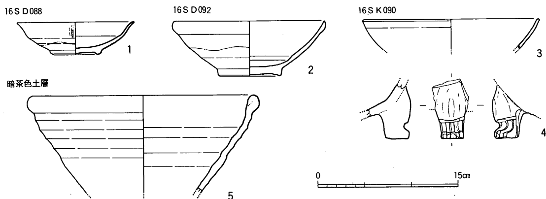
fig. 84 第16次調査 (6 A Y N - B 地区) 出土遺物実測図
