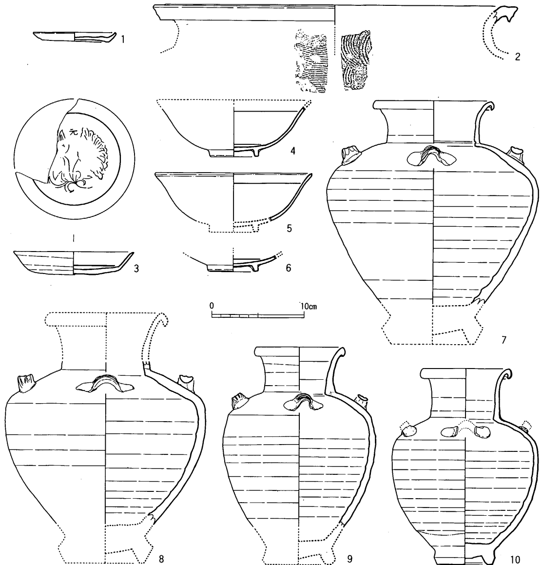
fig. 10 19SK004出土土器実測図 (Ⅰ)
