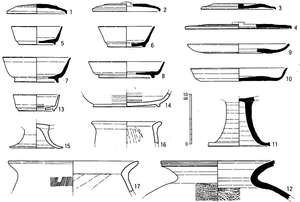
fig. 37 19SX075出土土器実測図
