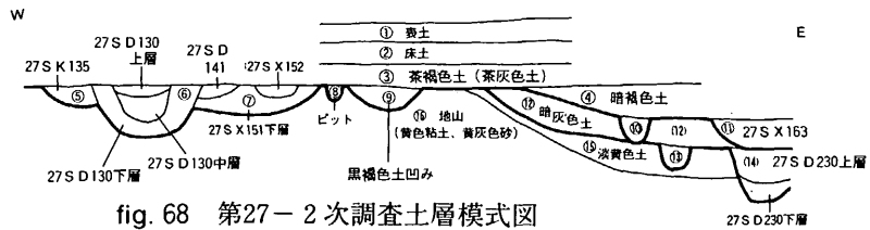
fig. 68 第27-2次調査土層模式図
