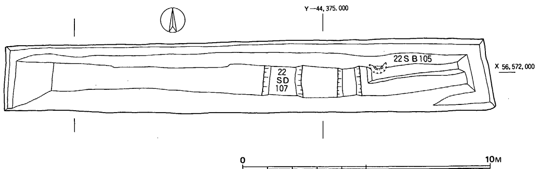
fig. 45 第22次調査遺構配置図
