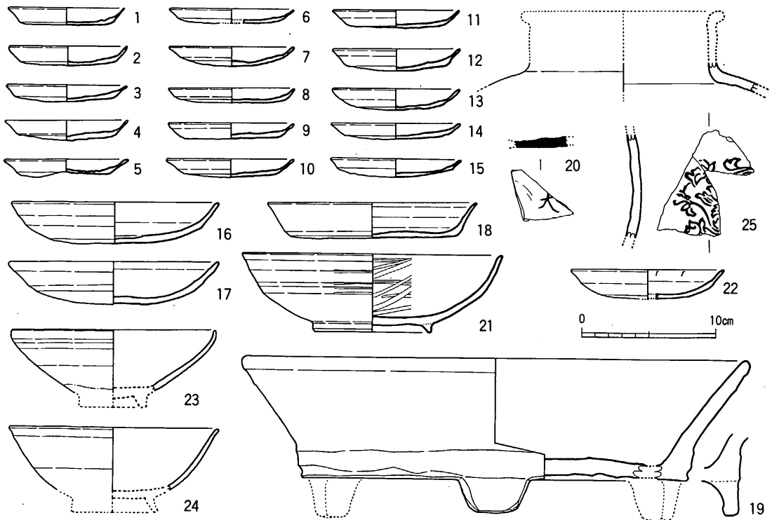
fig. 41 19SX055出土土器実測図
