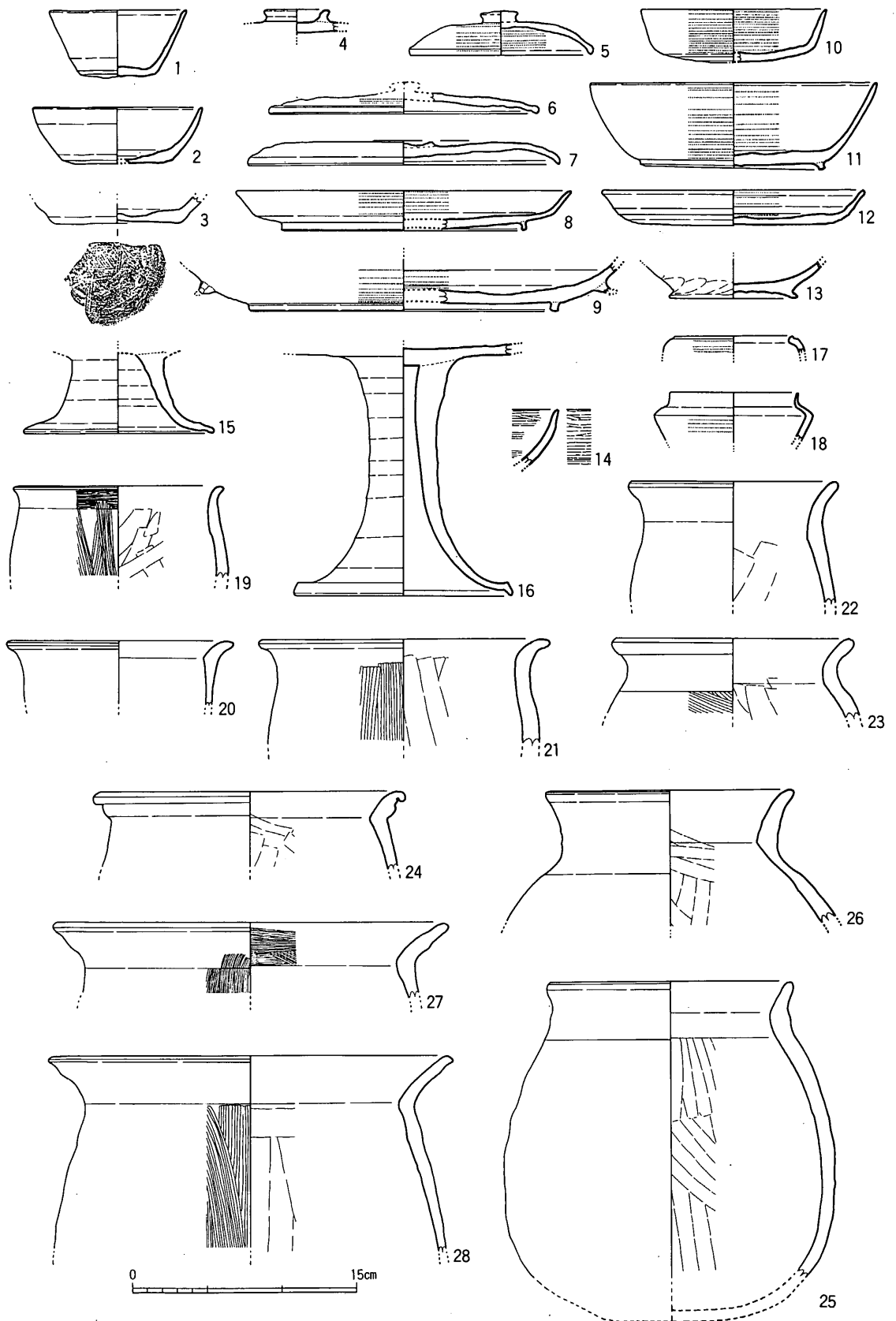
fig. 30 19SD080上層出土土器実測図 (I)
