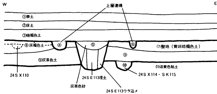
fig. 52 第24次調査土層模式図
