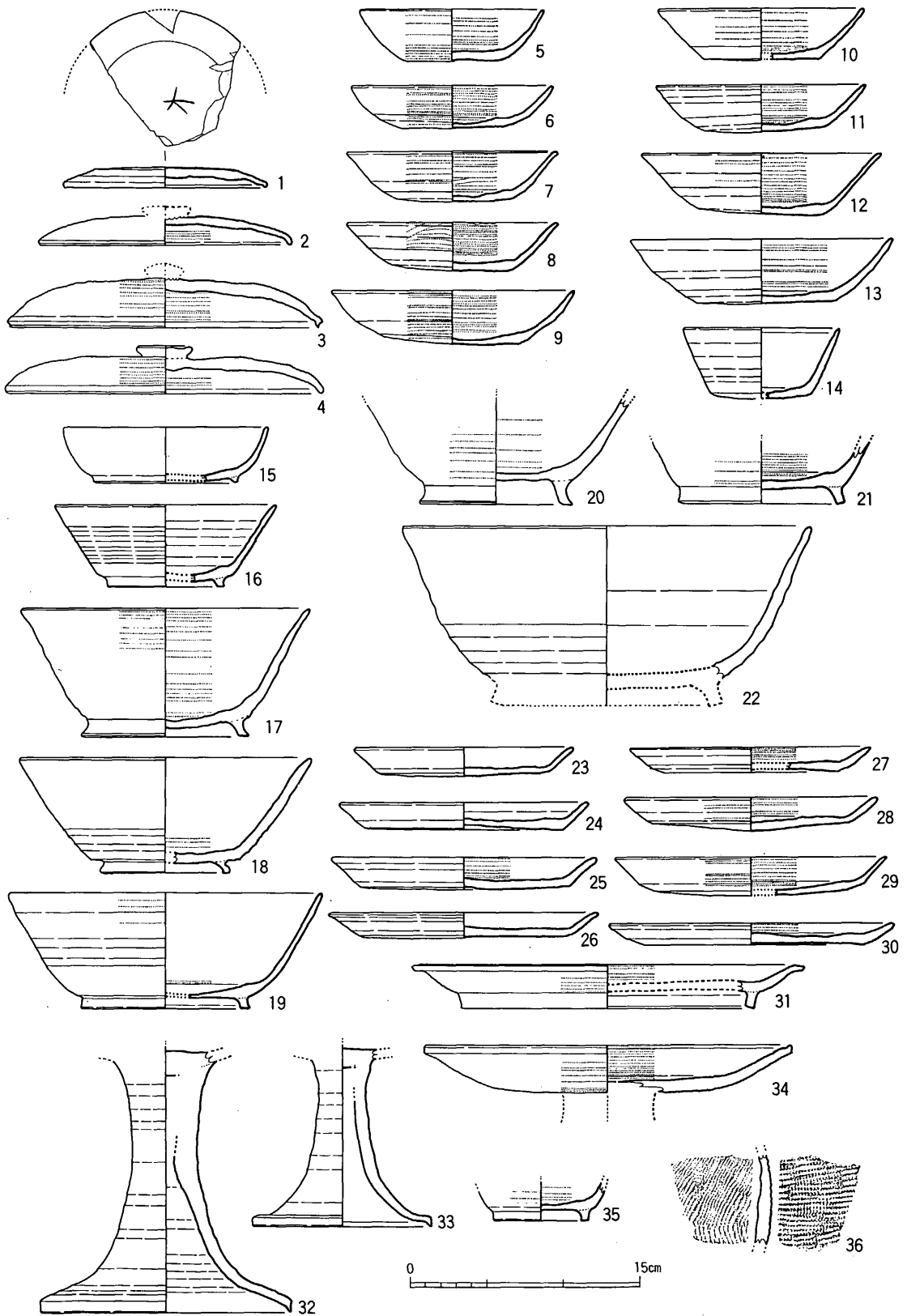
fig. 34 19SD080下層出土土器実測図 (I)
