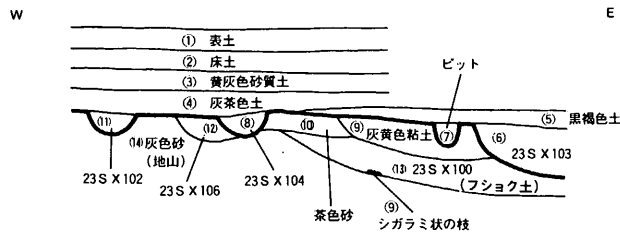
fig. 49 第23次調査土層模式図
