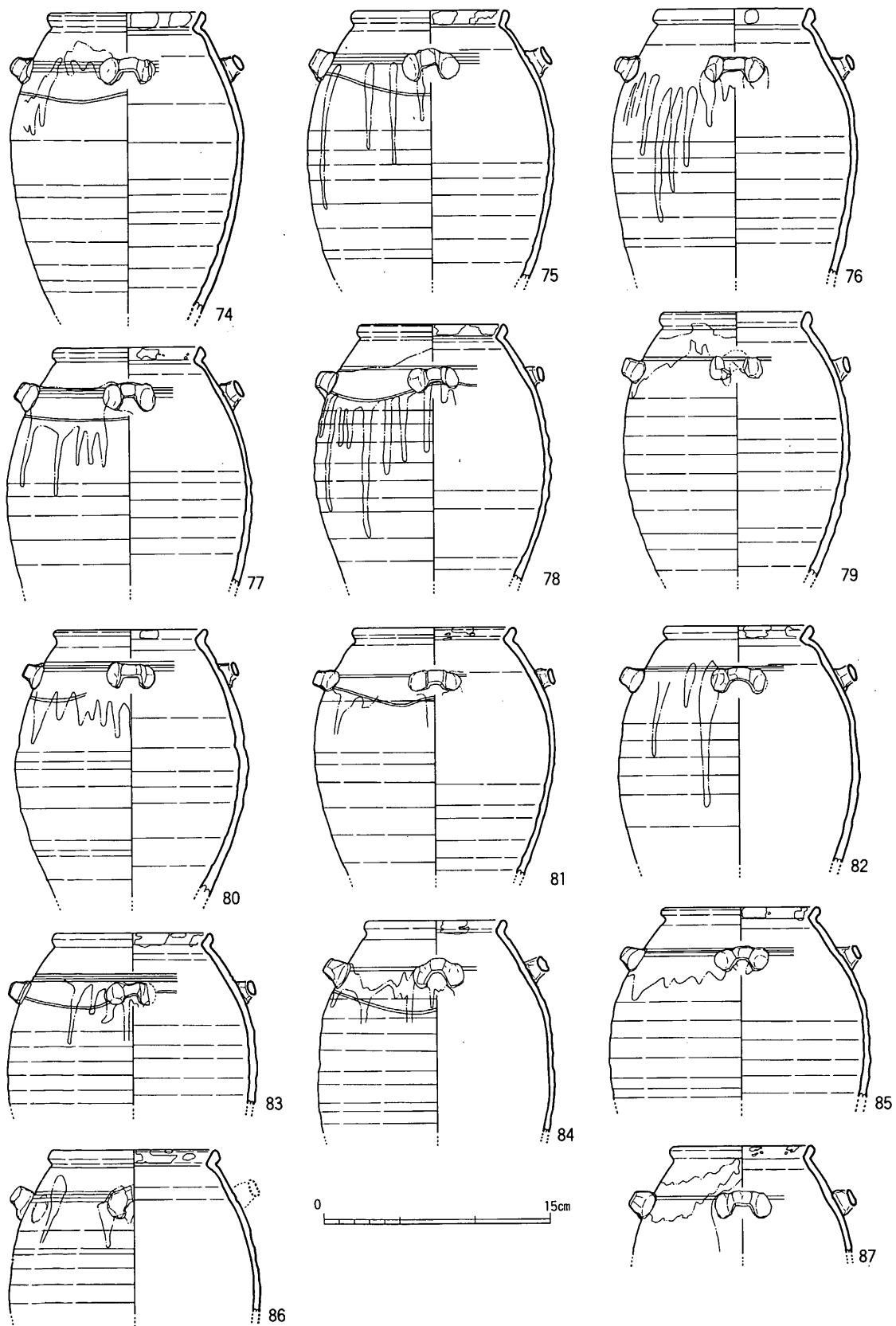
fig. 18 19SK004出土土器実測図 (IX)
