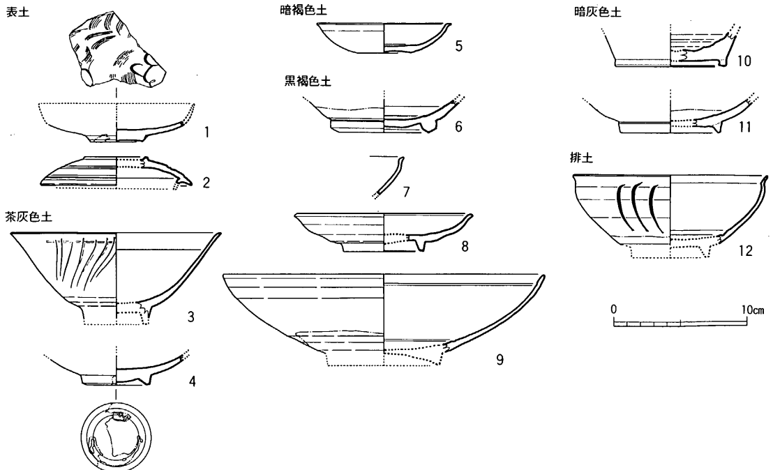
fig. 71 第27-2次調査各土層出土土器実測図
