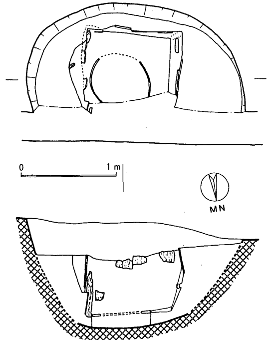
fig. 53 24 S E 113井戸実測図
