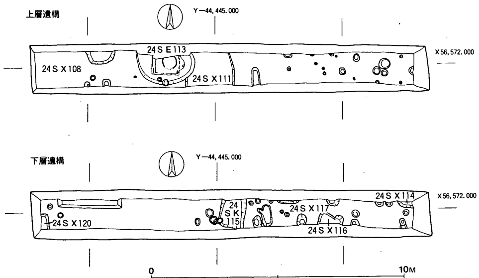
fig. 51 第24次調査遺構配置図
