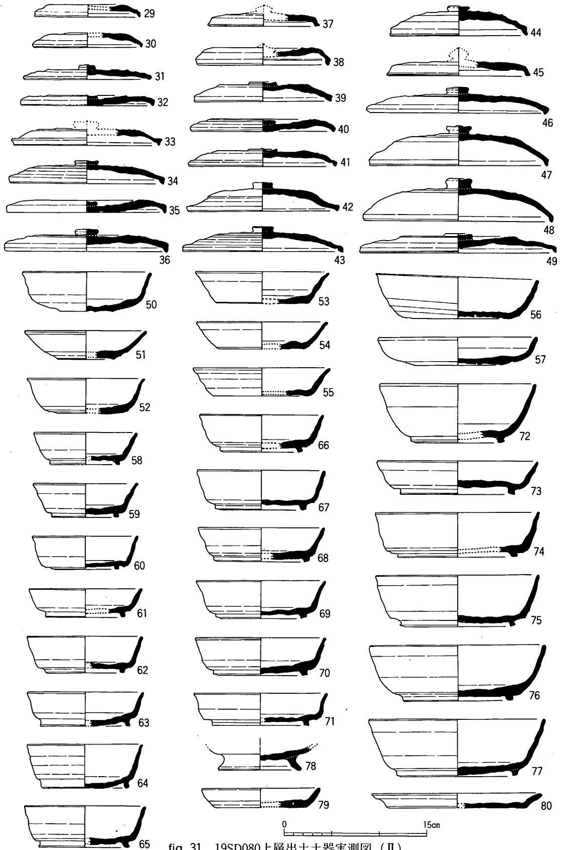
fig. 31 19SD080上層出土土器実測図 (II)
