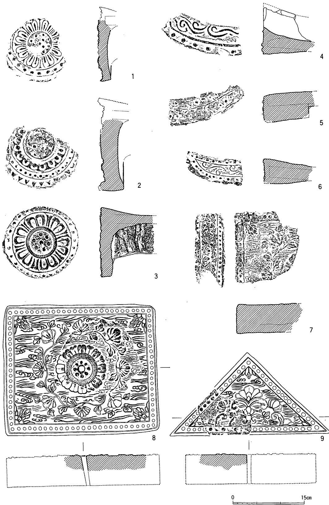
fig. 79 第21-1、22、25、26、27次調查出土瓦・磚實測圖
