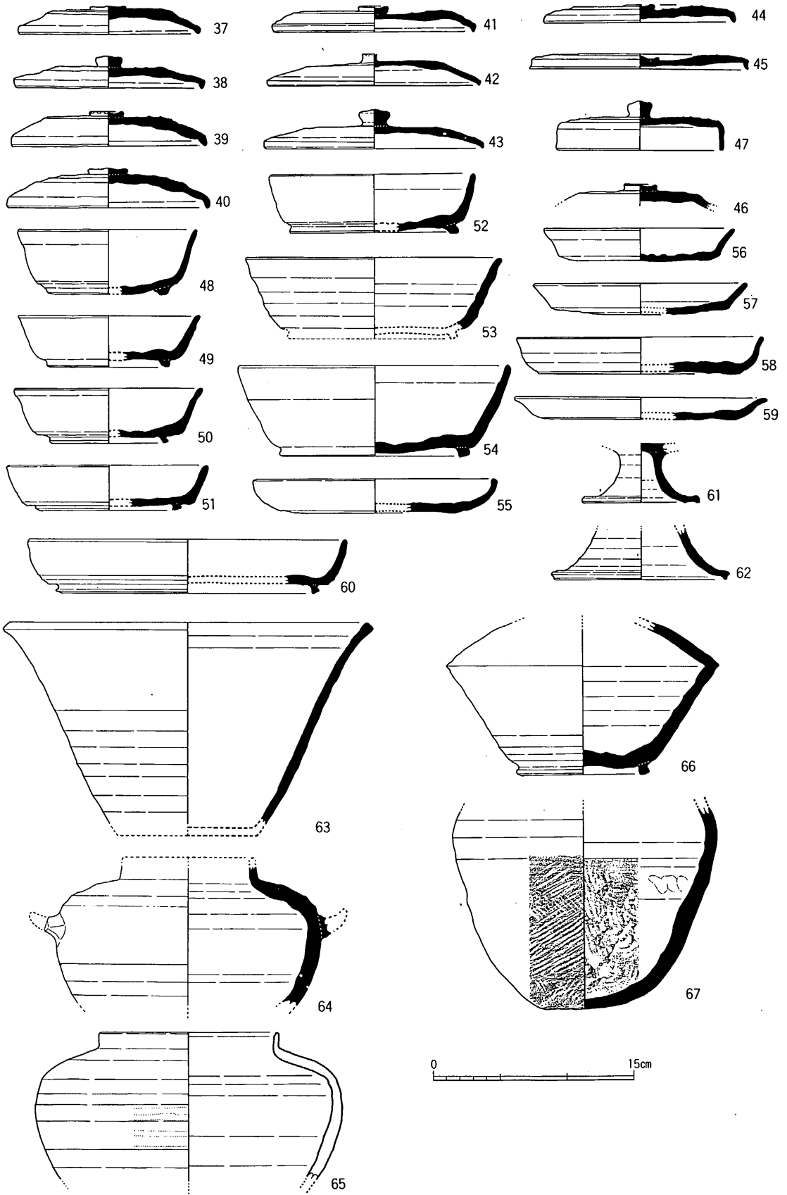
fig. 35 19SD080下層出土土器実測図(Ⅱ)
