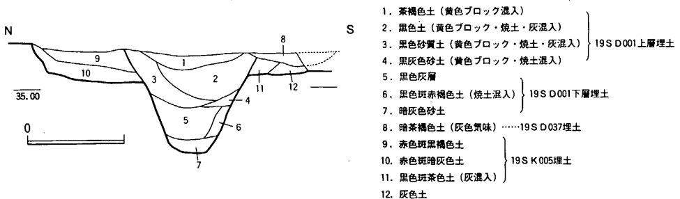
fig. 5 19S D 001土層図
