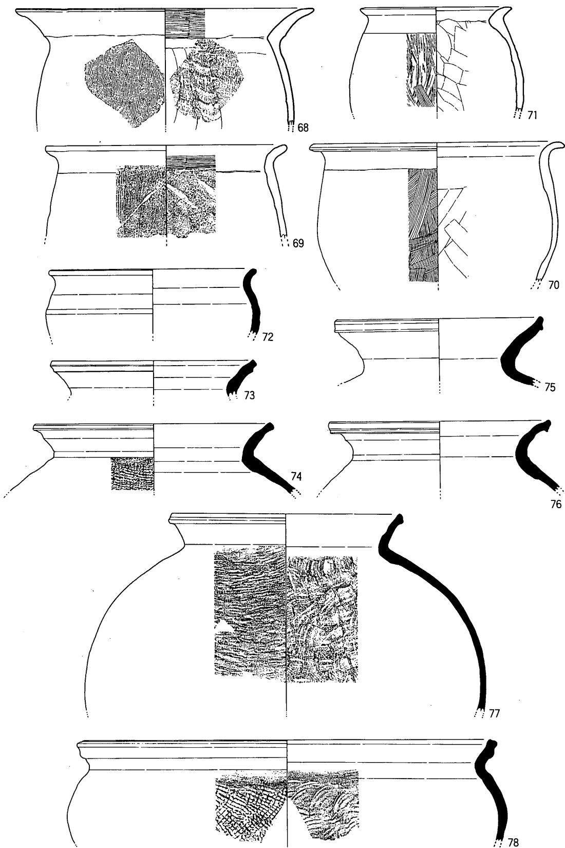
fig. 36 19SD080下層出土土器実測図 (Ⅲ)
