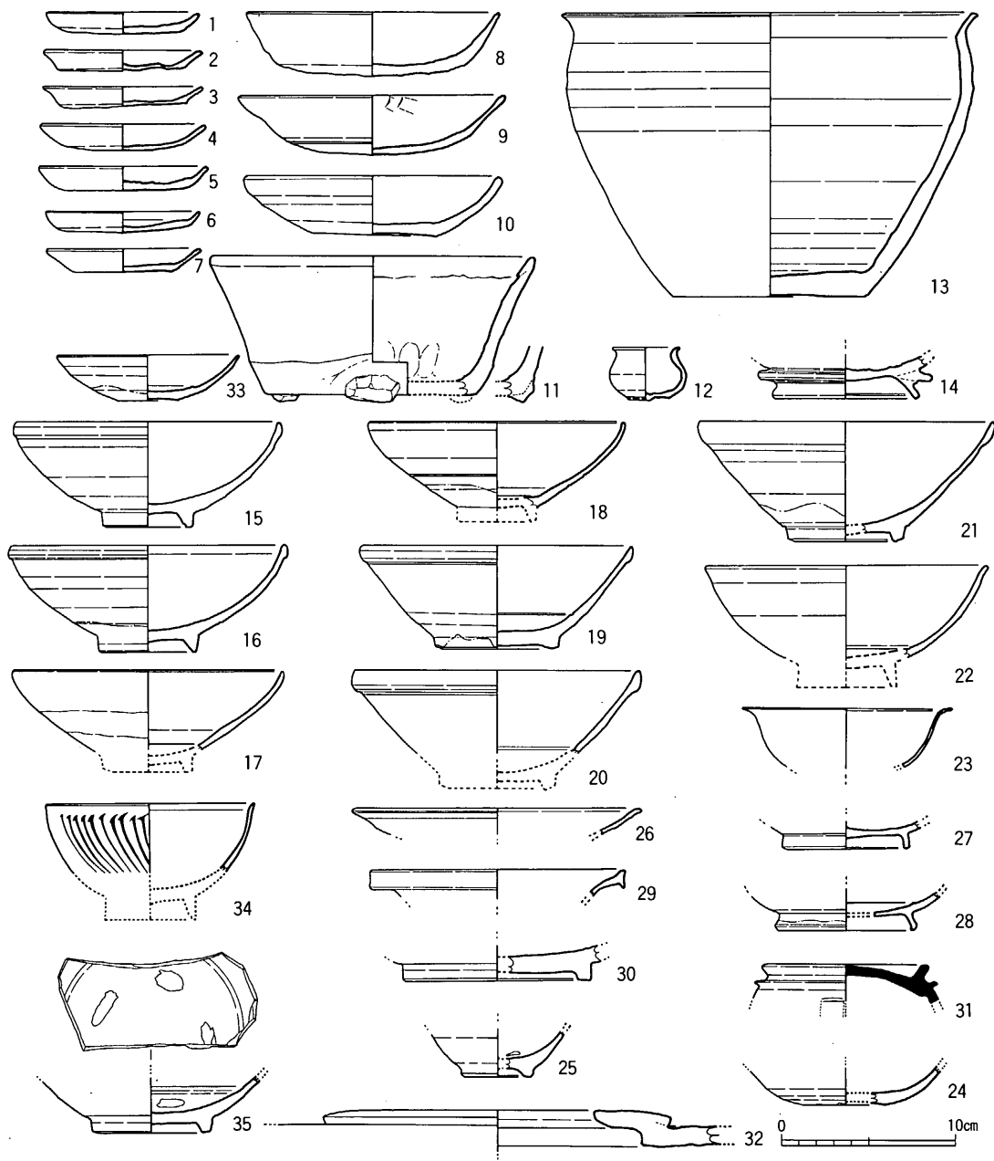
fig. 40 第19次調査灰色土層出土土器実測図
