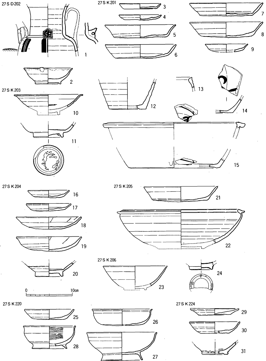
fig. 62 第27-1次調査各遺構出土土器実測図
