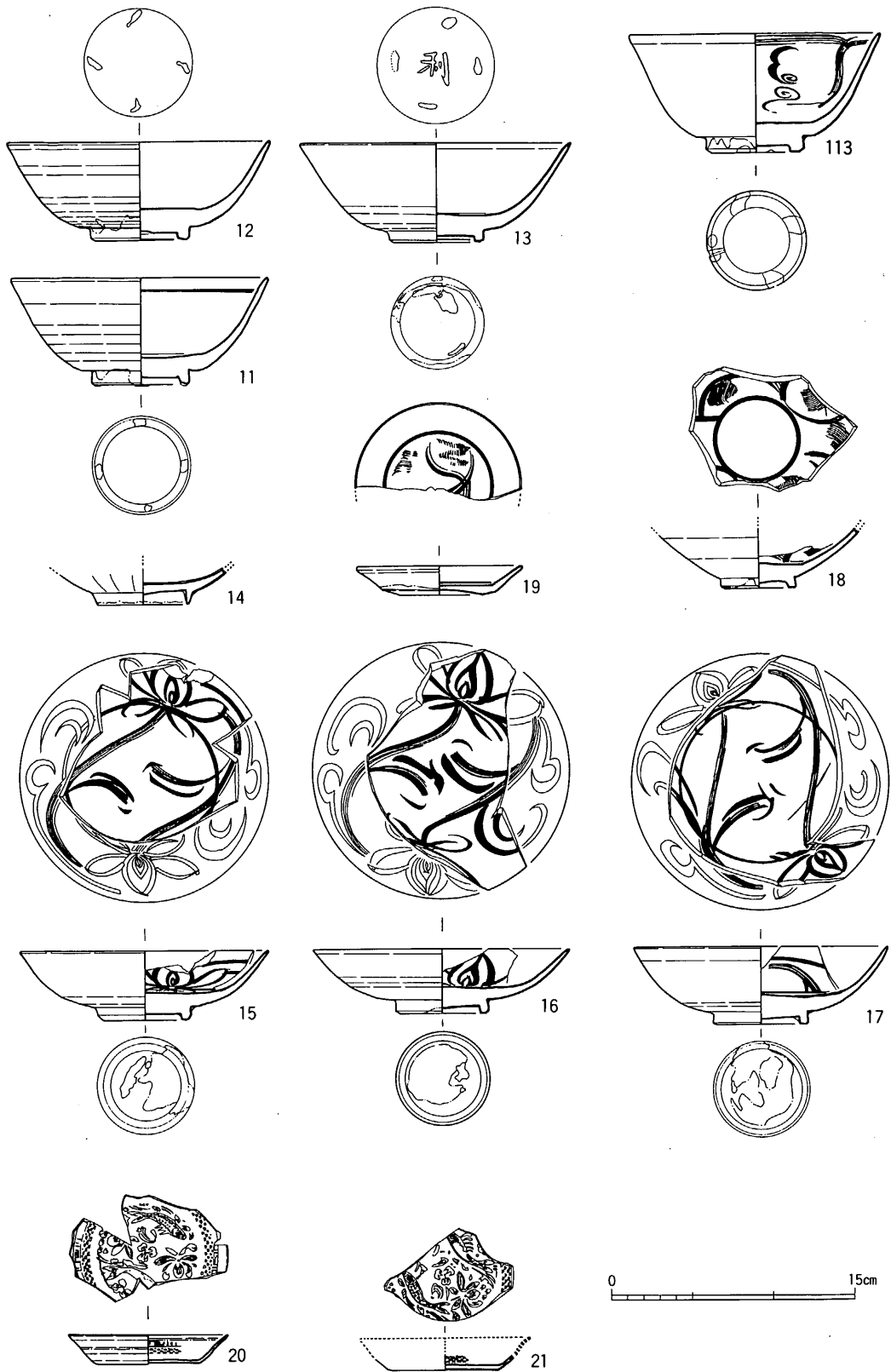
fig. 11 19SK004出土土器実測図 (Ⅱ)
