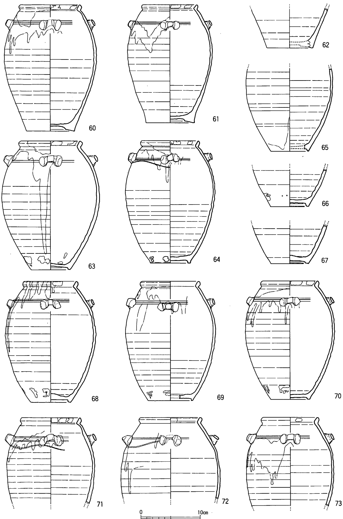
fig. 17 19SK004出土土器実測図 (Ⅷ)
