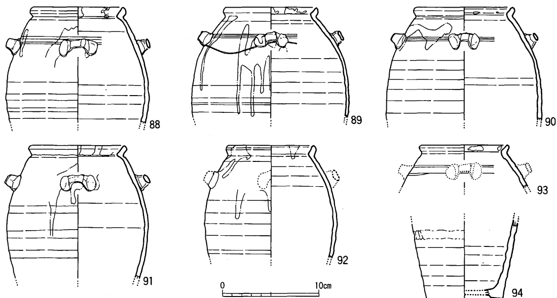
fig. 19 19SK004出土土器実測図(X)
