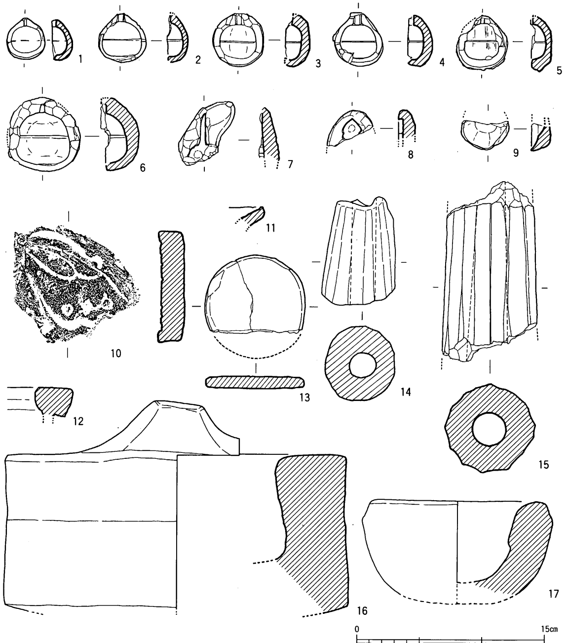
fig. 78 第19, 24, 26, 27-1・2次調査出土生産関係遺物
