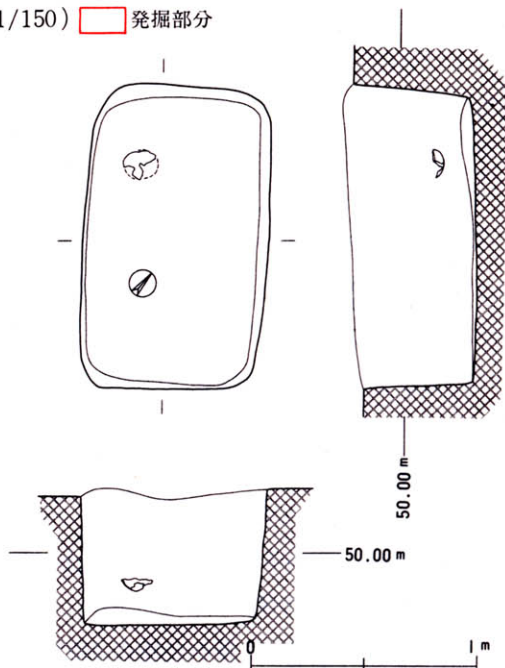
Fig 40. ST086 実測図
