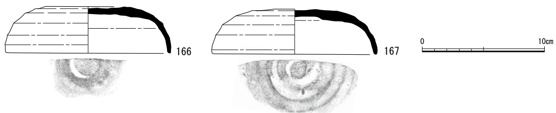
第28図 野添12号窯跡出土遺物実測図（1/3）
