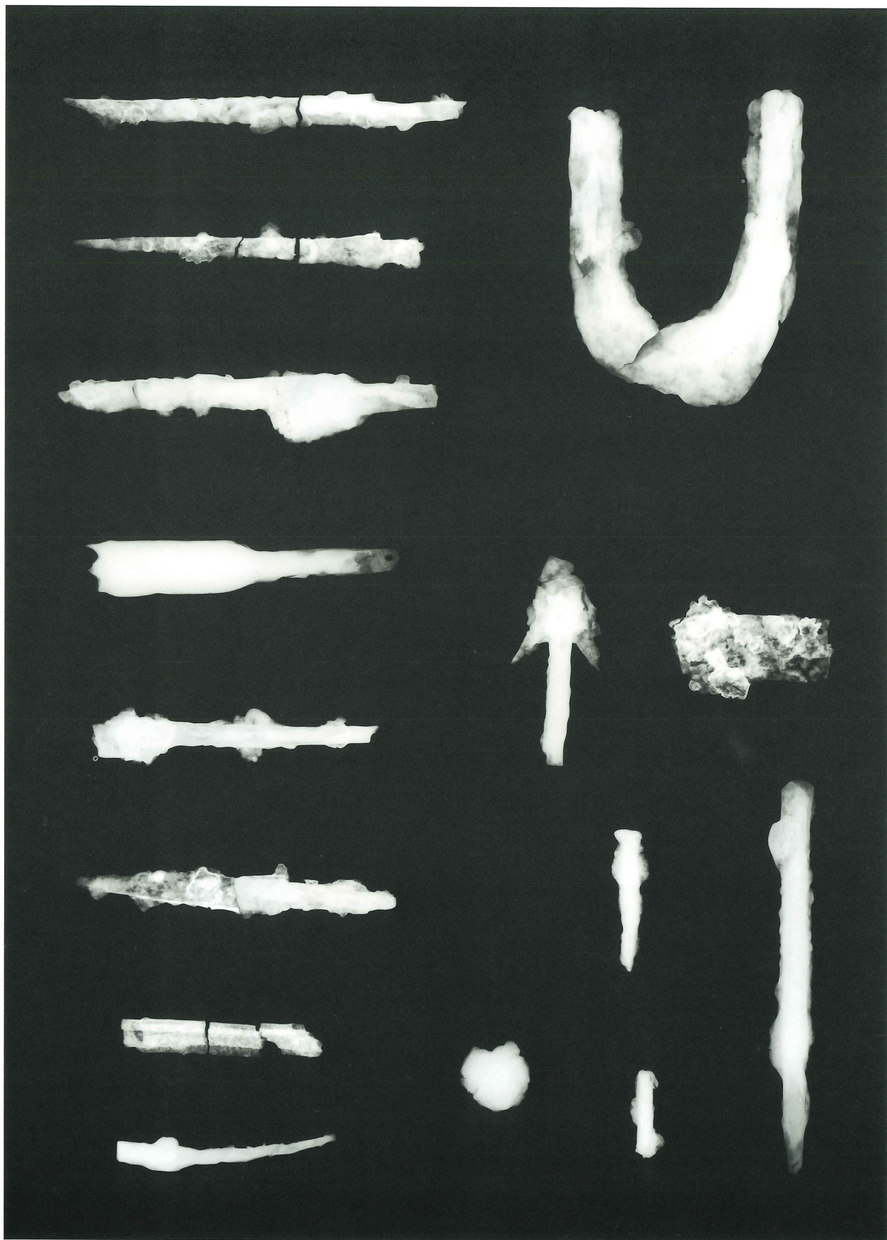
鉄製品 X線写真 第9図7 第17図50 第19図33 第20図8 第24図58 第29図8 第43図49 第66図17 第76図12 第78図29 第82図5 第113図12 第140図41・42・43 第146図69
