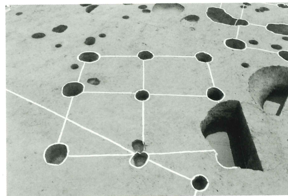
F区第40号掘立柱建物跡
