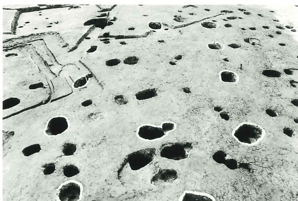
F区第5号掘立柱建物跡
