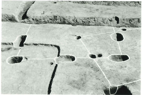
F区第78号掘立柱建物跡
