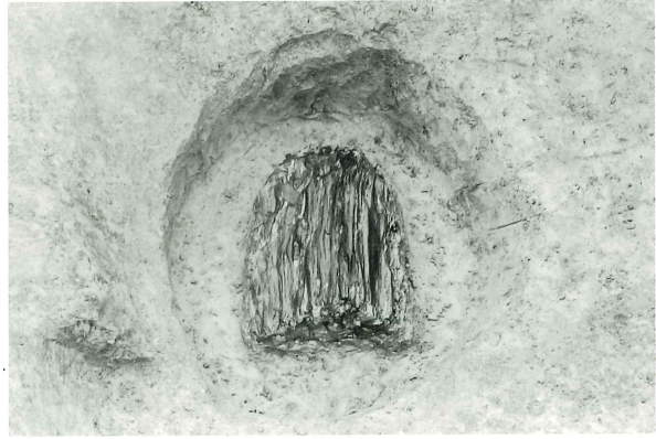
F 区第13号掘立柱建物跡 P 5 敷板検出状況
