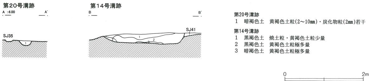
第493图 F区沟迹 (20) (第67图)
