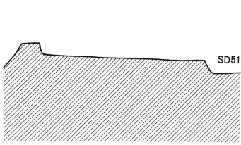
第73号溝跡 A 16.00
