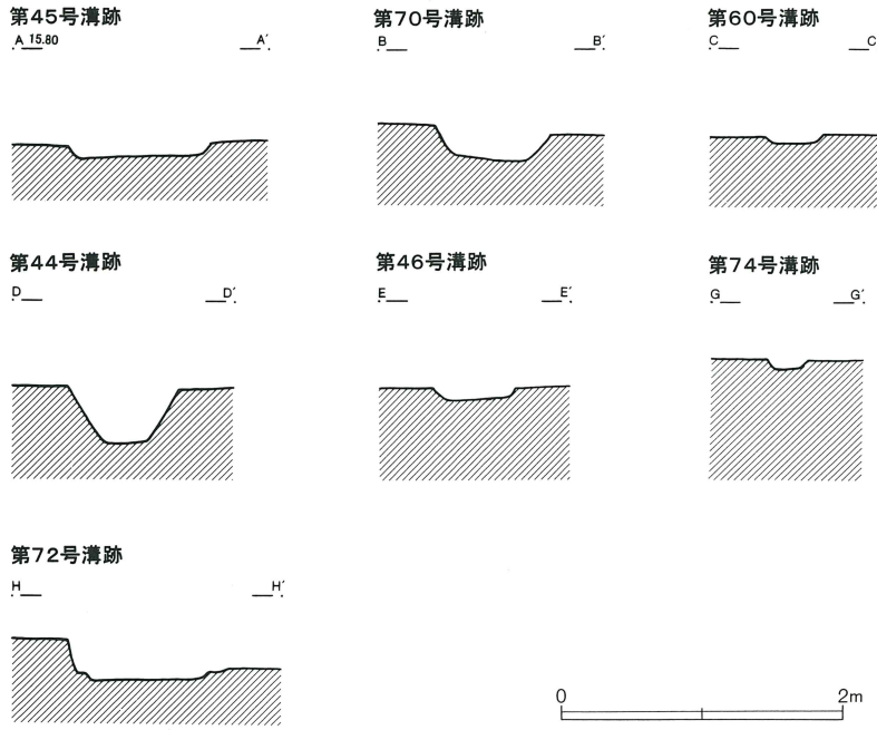
第481図 F区溝跡(8)(第54図)
