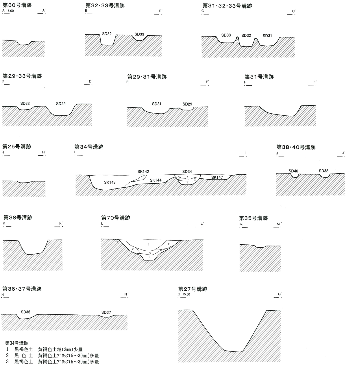
第485図 F区溝跡(12)(第58図)
