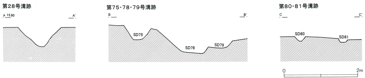
第490图 F区沟迹(17)(第63图)
