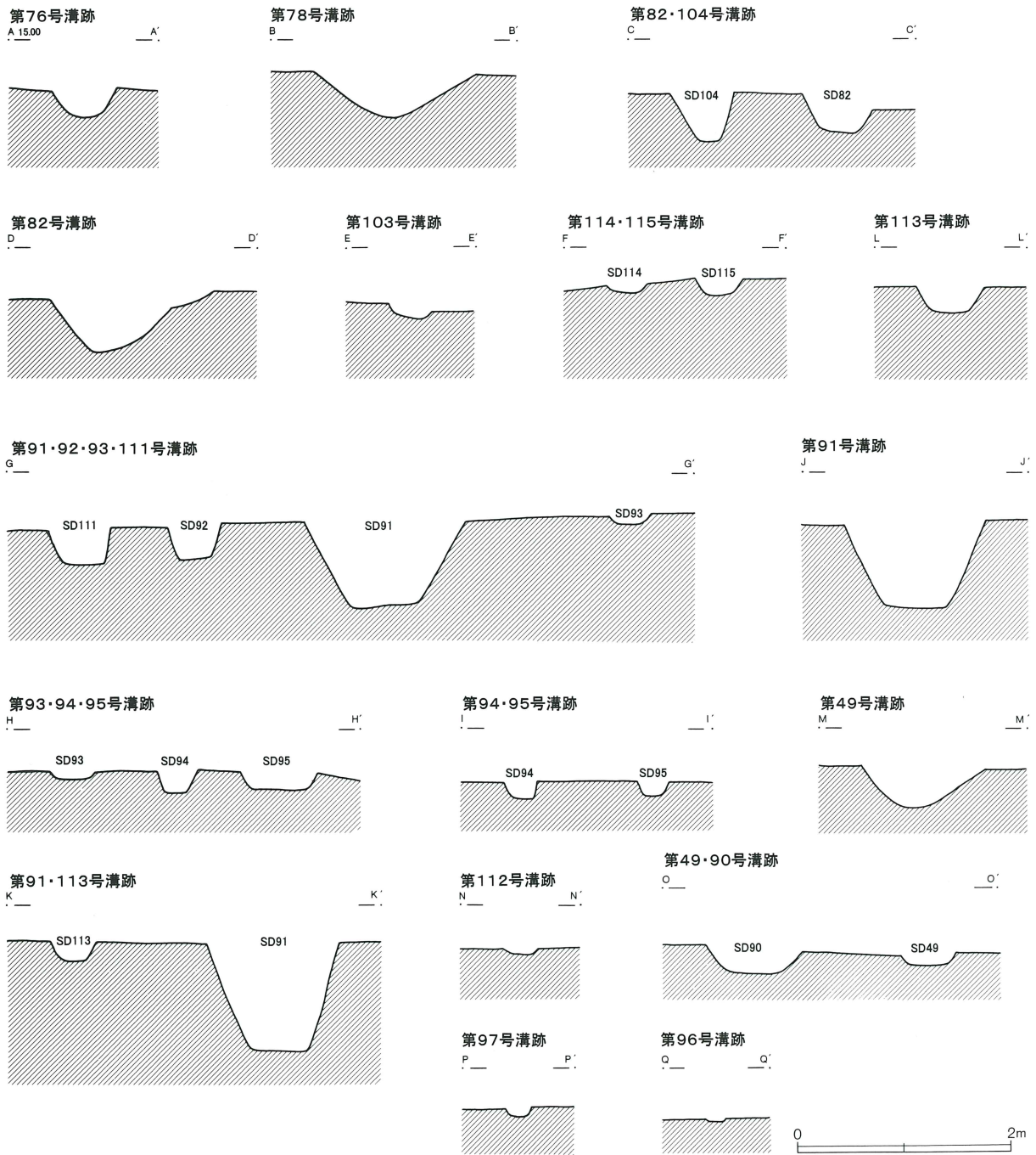
第487图 F区沟迹(14)(第60图)
