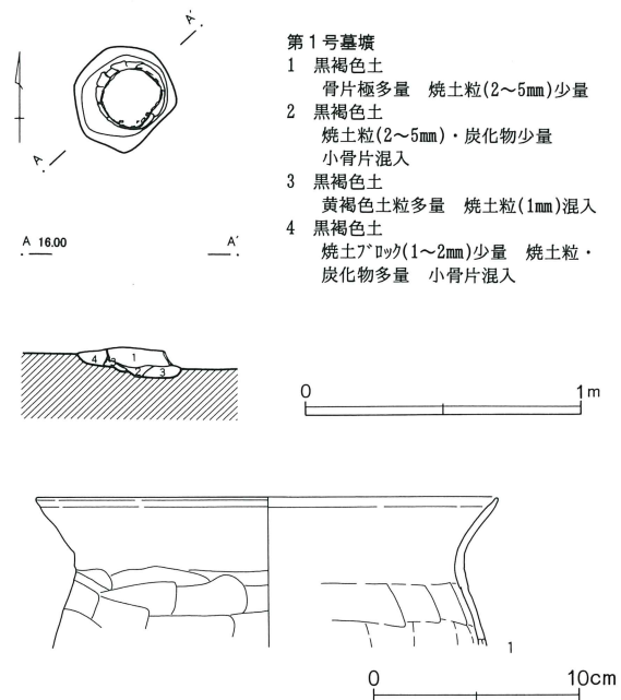
第503図 F区第1号墓墳・出土遺物
