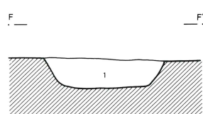
第85号溝跡 F
