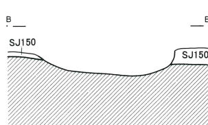
第127号溝跡 B
