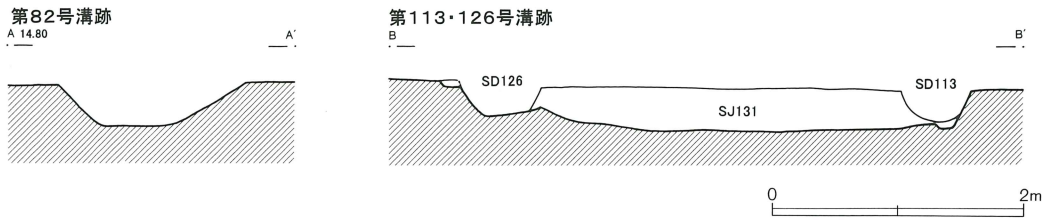
第484図 F区溝跡(11)(第57図)
