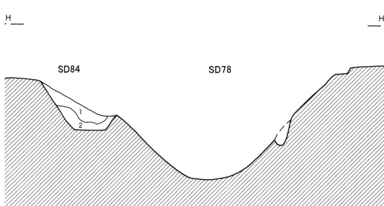
第78・84号溝跡 H
