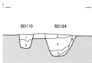
第110・124号溝跡 I
