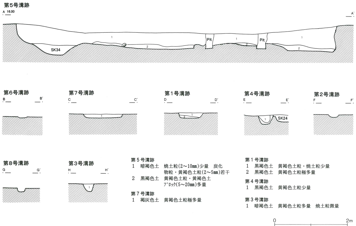
第493图 F区沟迹 (20) (第67图)
