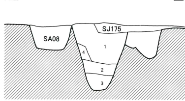
第53号溝跡 B
