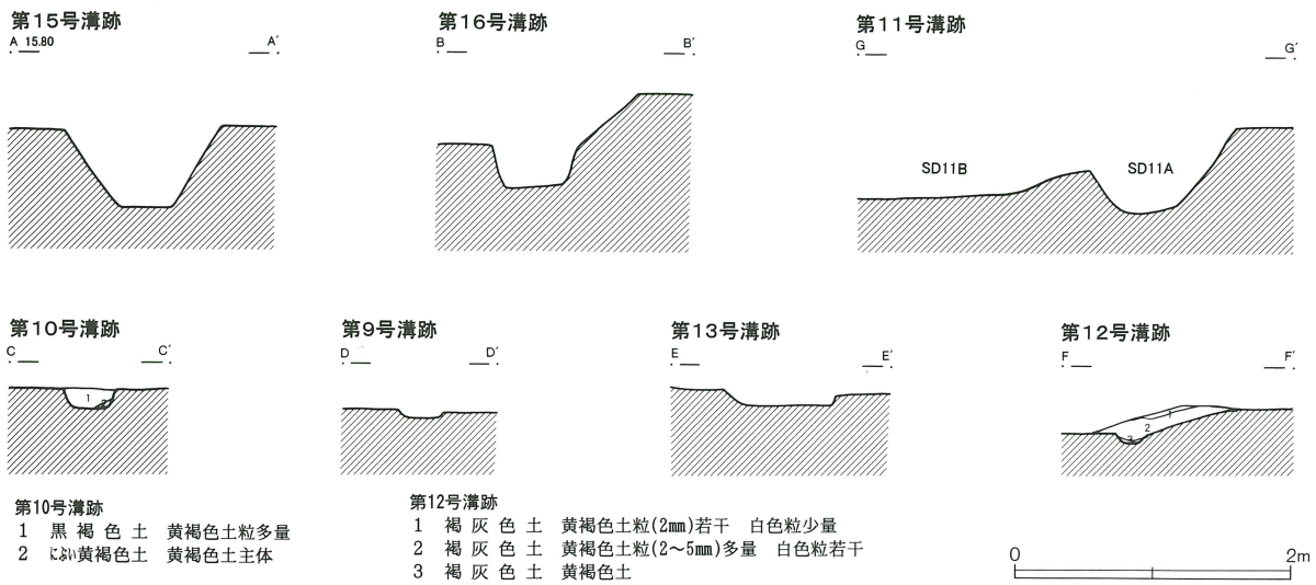
第492图 F区沟迹 (19) (第66图)
