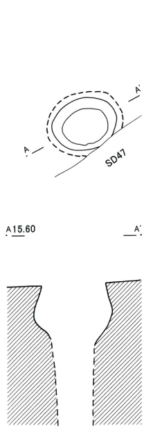
第77号井戸跡
