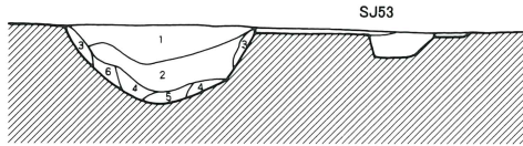
第50・53号溝跡
