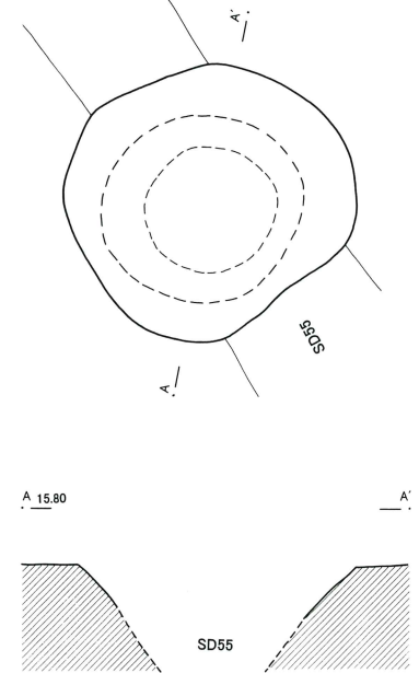
第86号井戸跡
