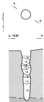
第211号井戸跡
