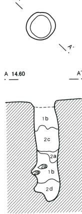
第215号井戸跡
