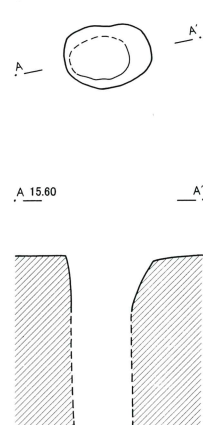
第101号井戸跡
