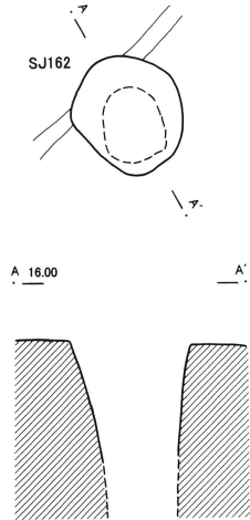
第242号井戸跡
