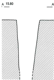
第148号井戸跡
