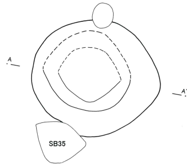
第88号井戸跡
