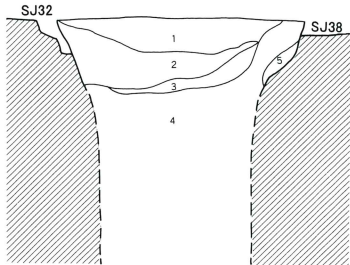
第171号井戸跡
