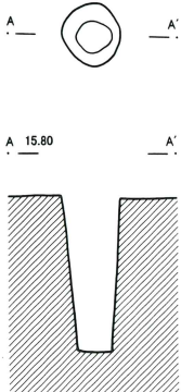
第191号井戸跡
