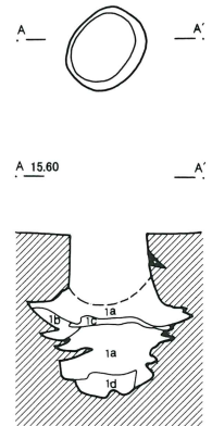
第125号井戸跡
