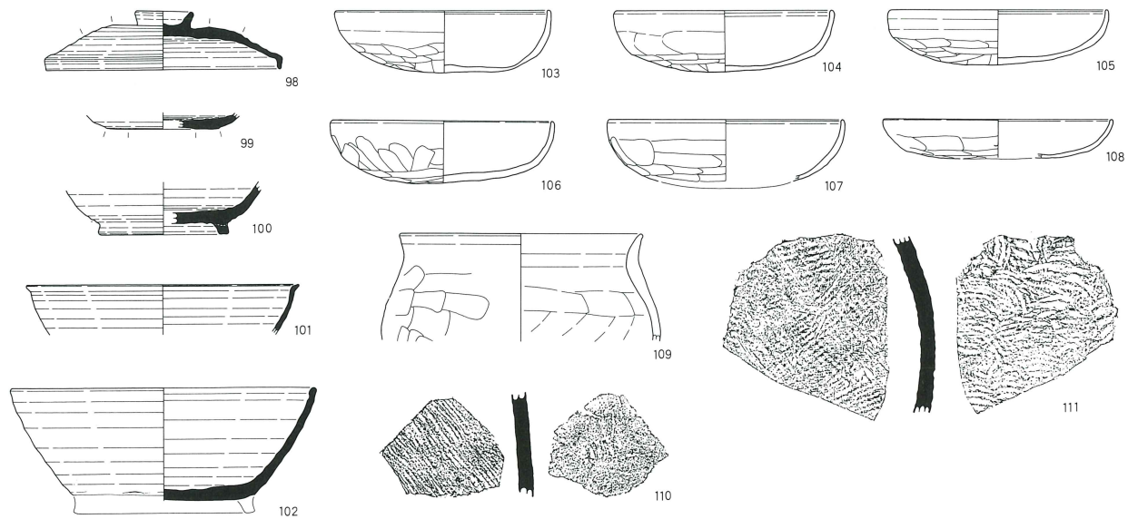
第88号井戸跡
