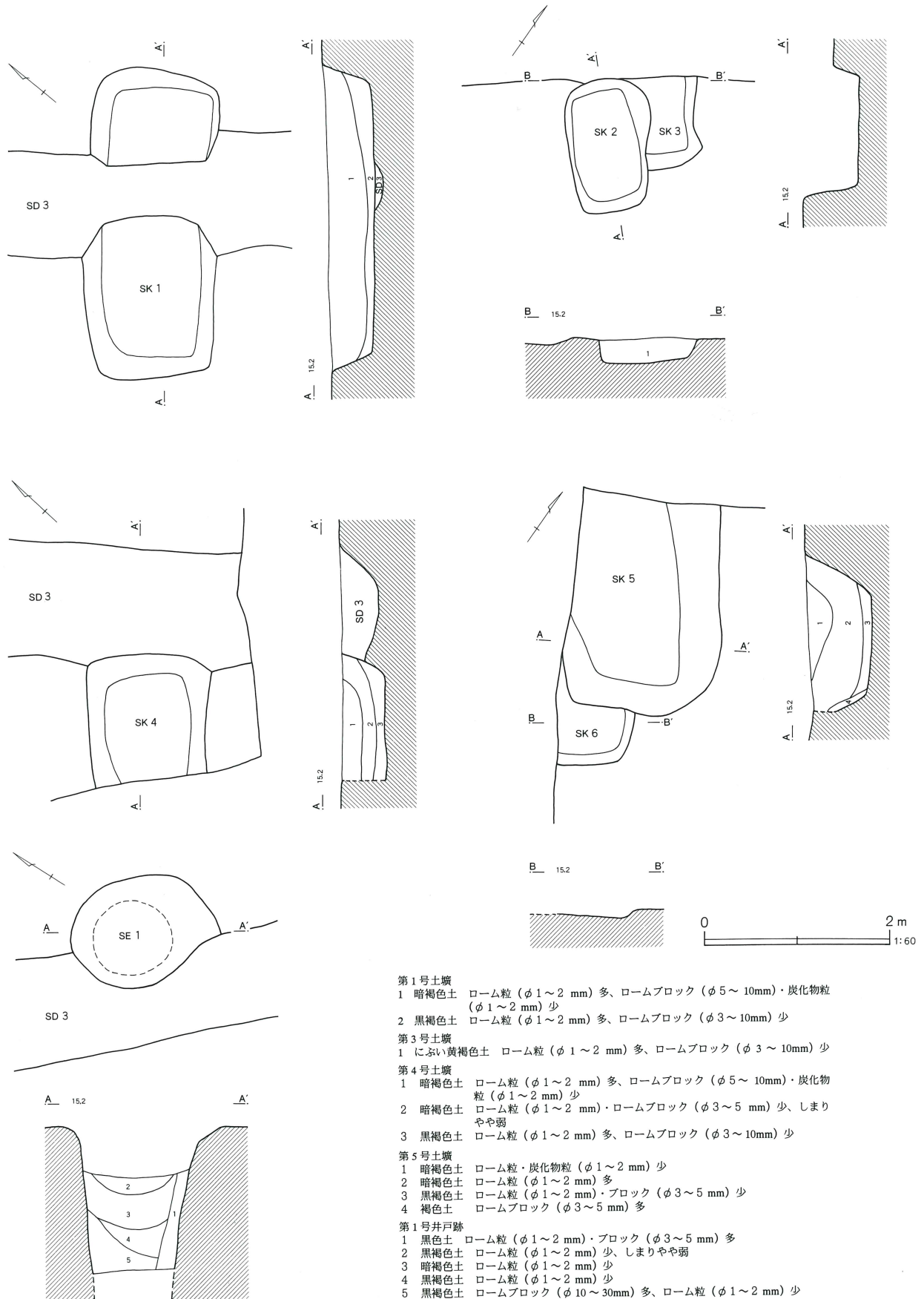
第5図 第1～6号土壇、第1号井戸跡
