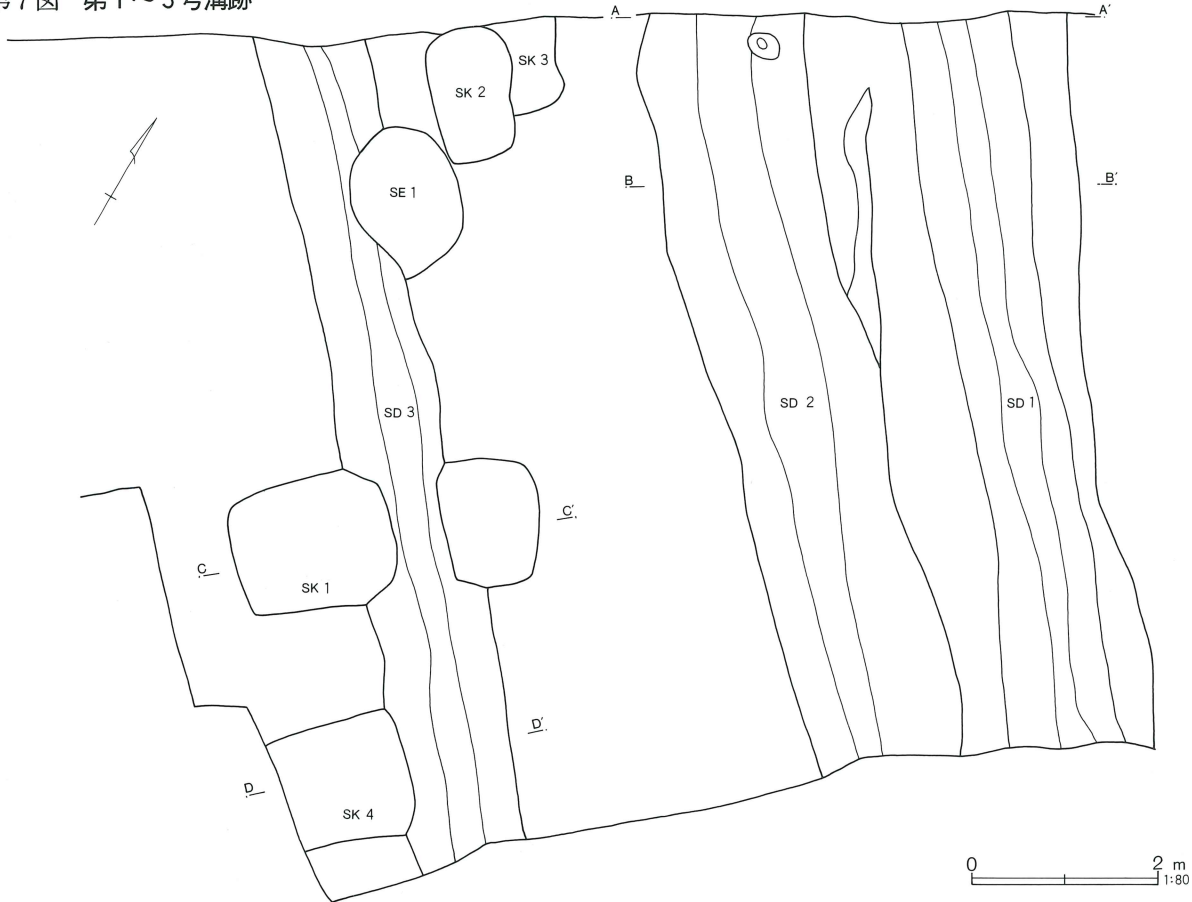
第7図 第1～3号溝跡
