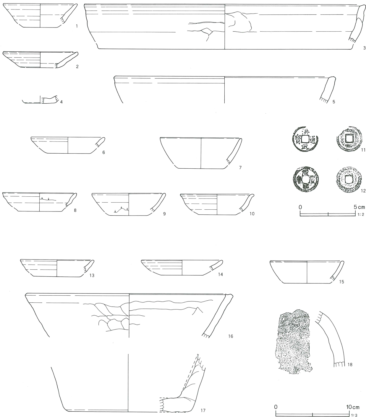
第6図 第1～5号土壙、第1号井戸跡出土遺物
