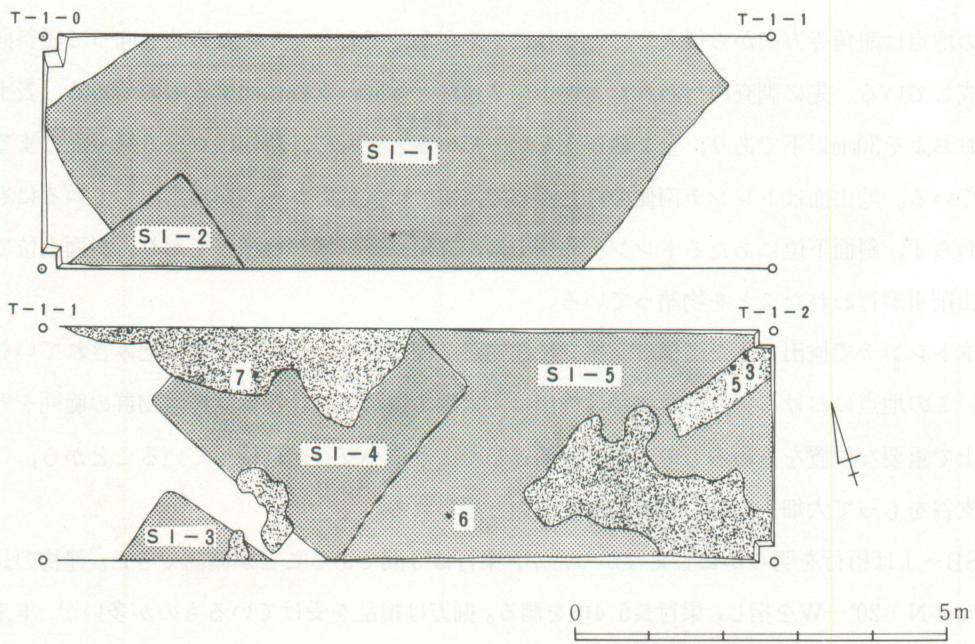
第2図 トレンチ1平面図
