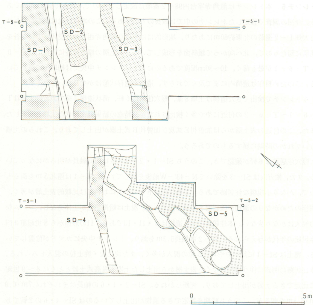
第9図 トレンチ5平面図
