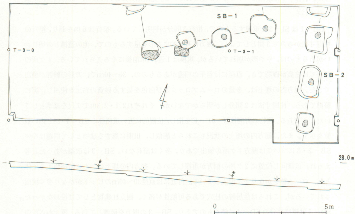
第6図 トレンチ3平面図
