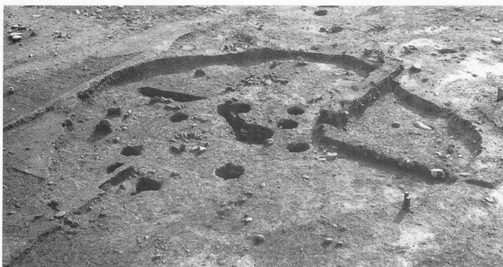
平面 G 20㊦住居跡
