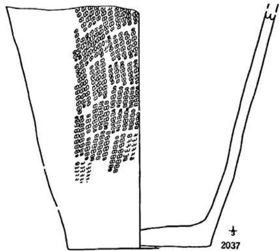
F 21 土器埋設遺構
