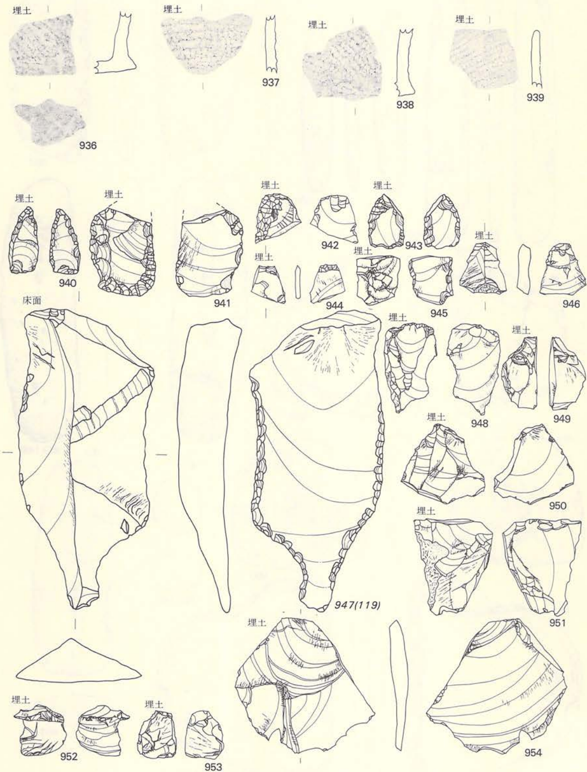
第55图 F IV - 4 住居址
