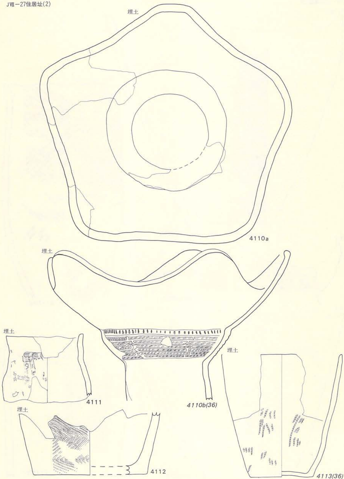
第213図 JVII-27住居址
