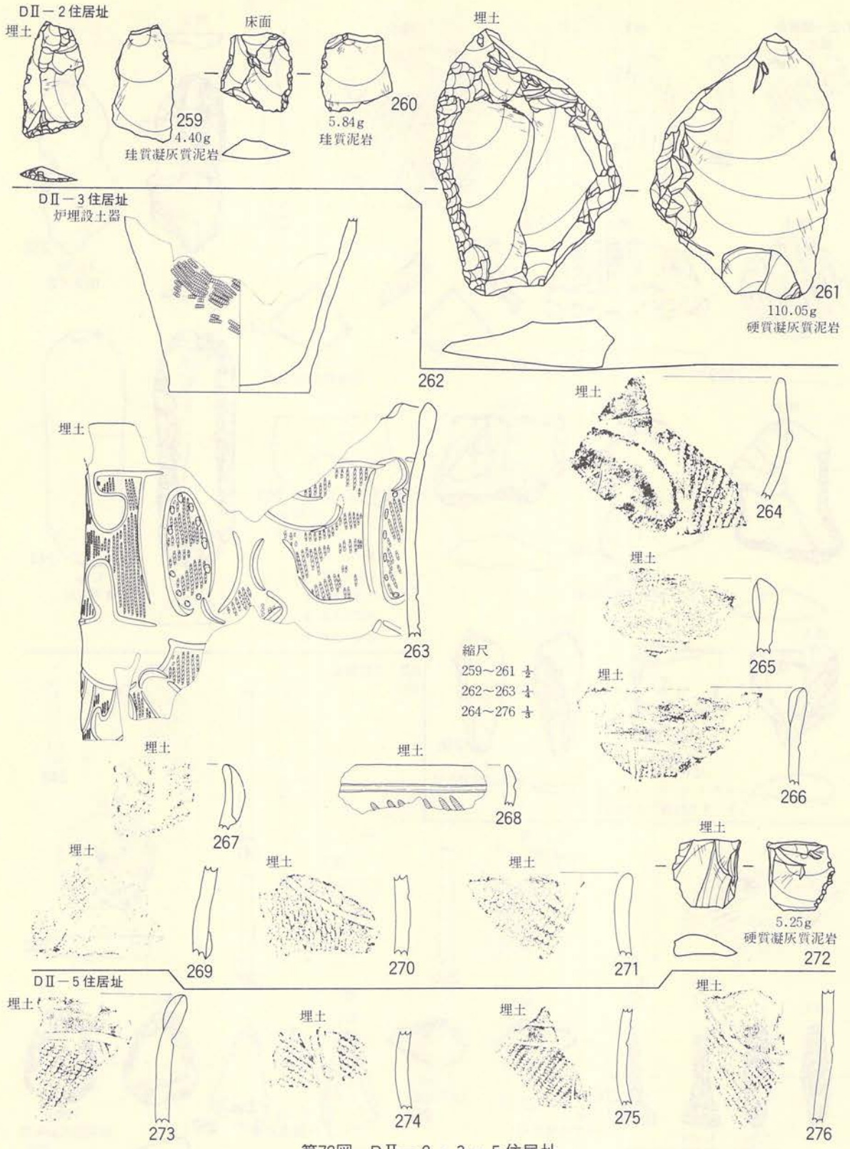
第72図 DII-2・3・5住居址
