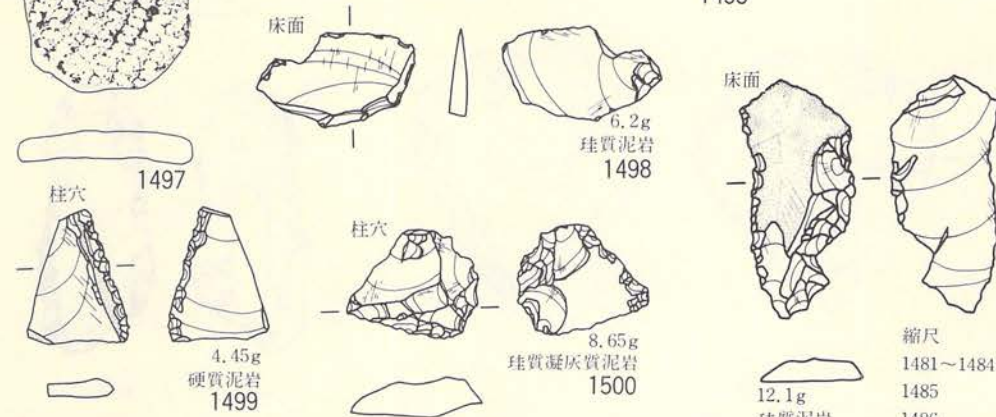
第159图 F II-16·17住居址
