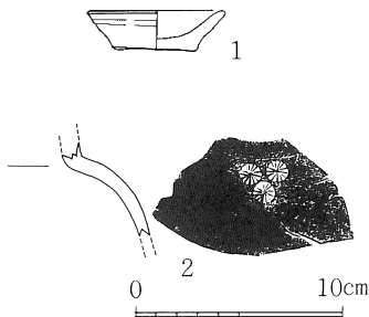
Fig. 14 P005・015出土遺物 実測図 (S=1/4)
