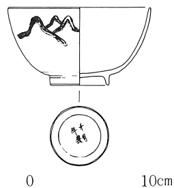
Fig. 4 SK002出土遺物実測図 (S=1/4)
