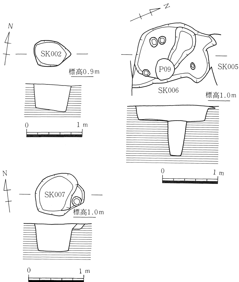
Fig. 3 SK002・007実測図 (S=1/40)
