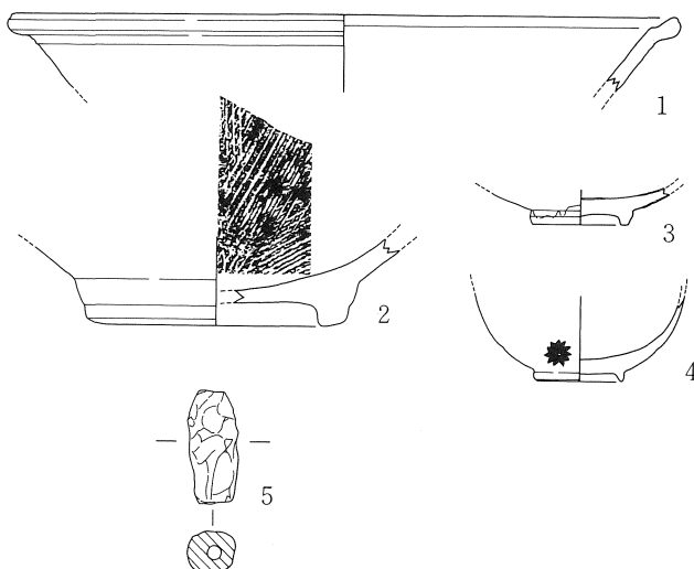
Fig. 15 その他の出土遺物実測図 (S = 1/4)
