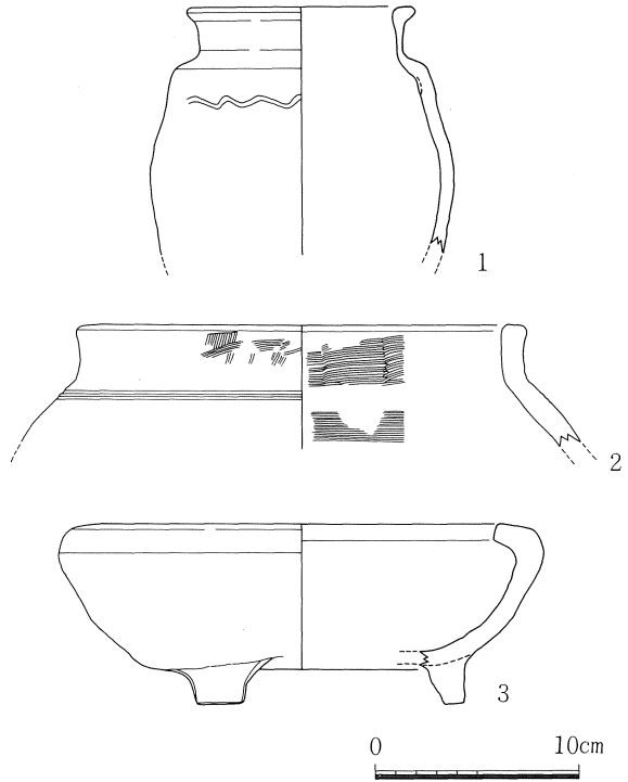
Fig. 7 SK031・032出土遺物実測図 (S=1/4)
