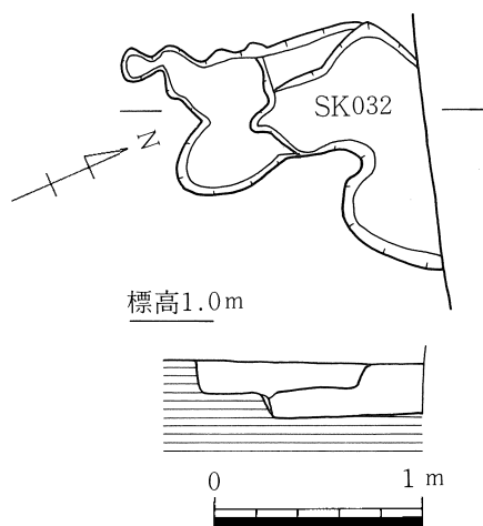
Fig. 6 SK031・032実測図 (S=1/40)
