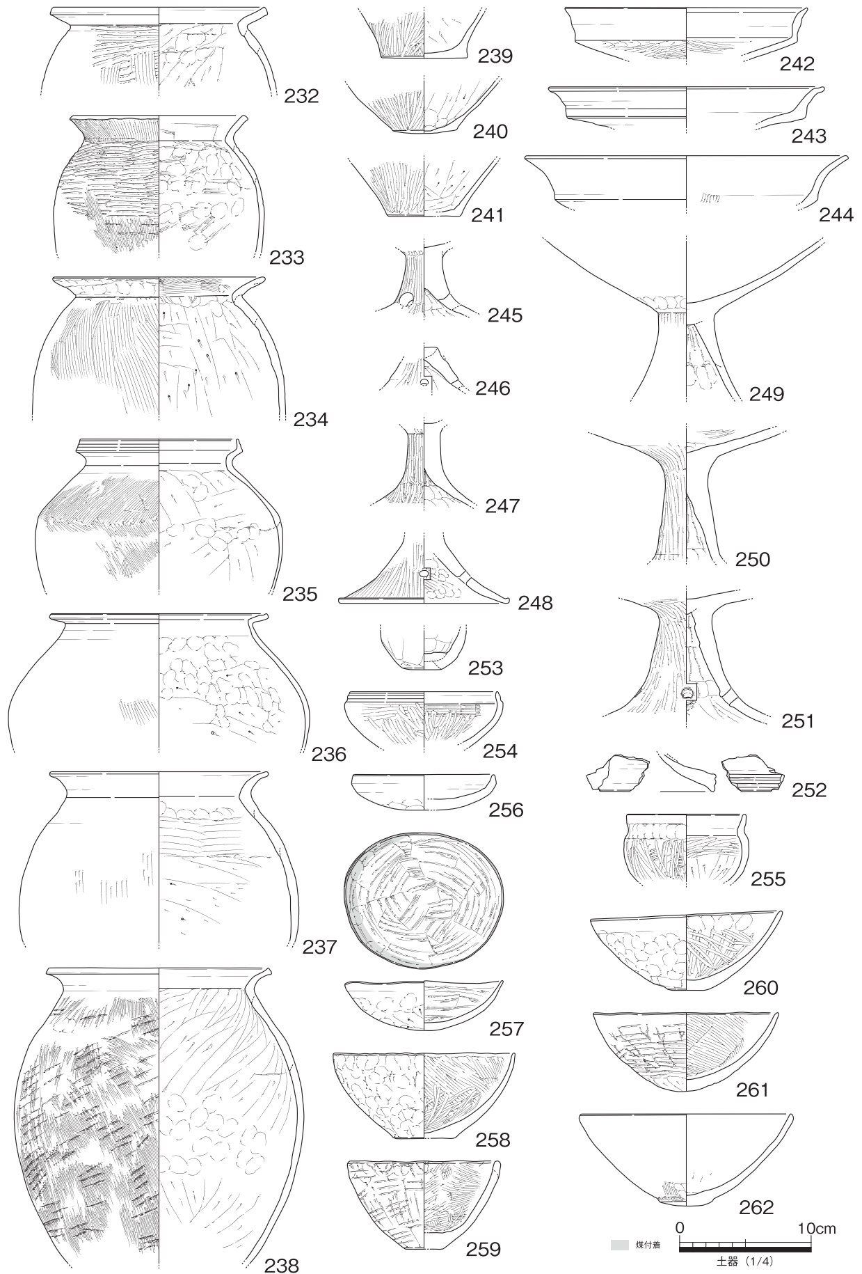
第 89 図 SD093 出土遺物実測図 2
