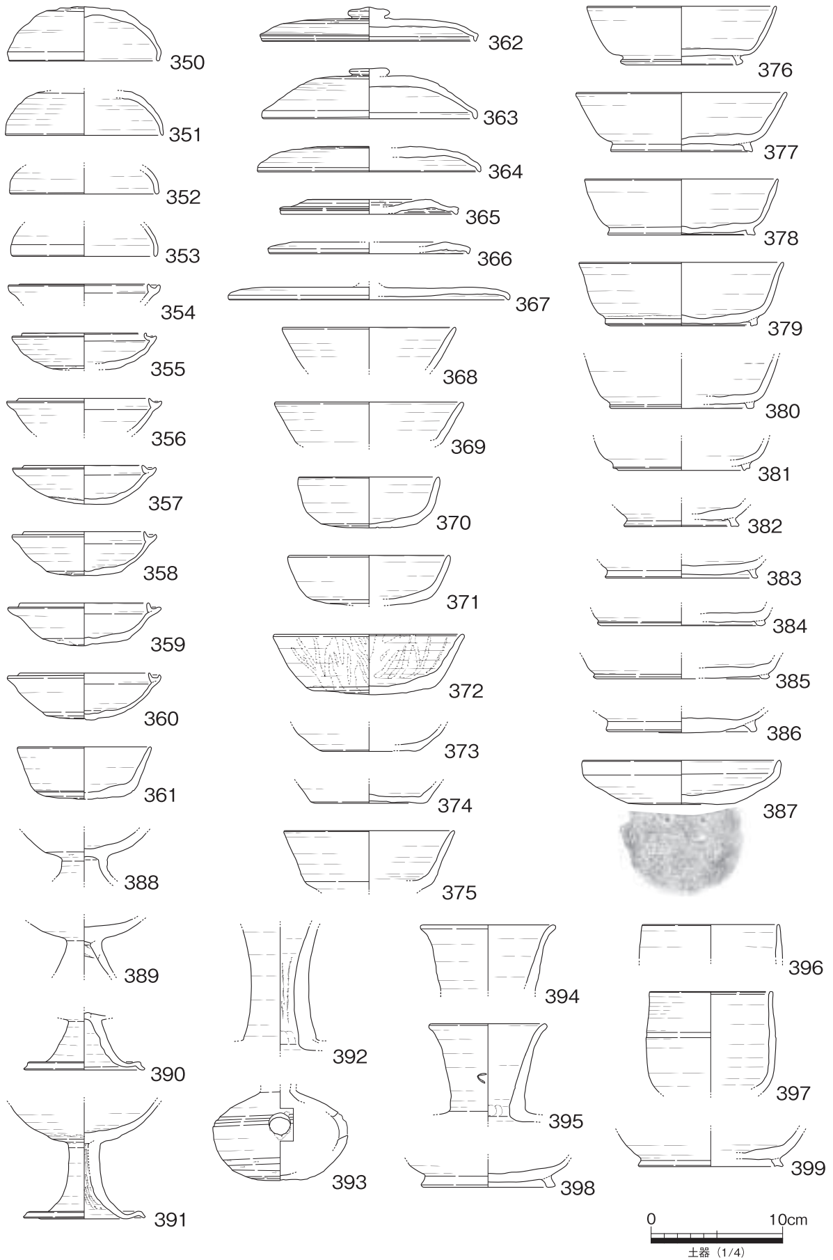
第 94 図 SD093 出土遺物実測図 7
