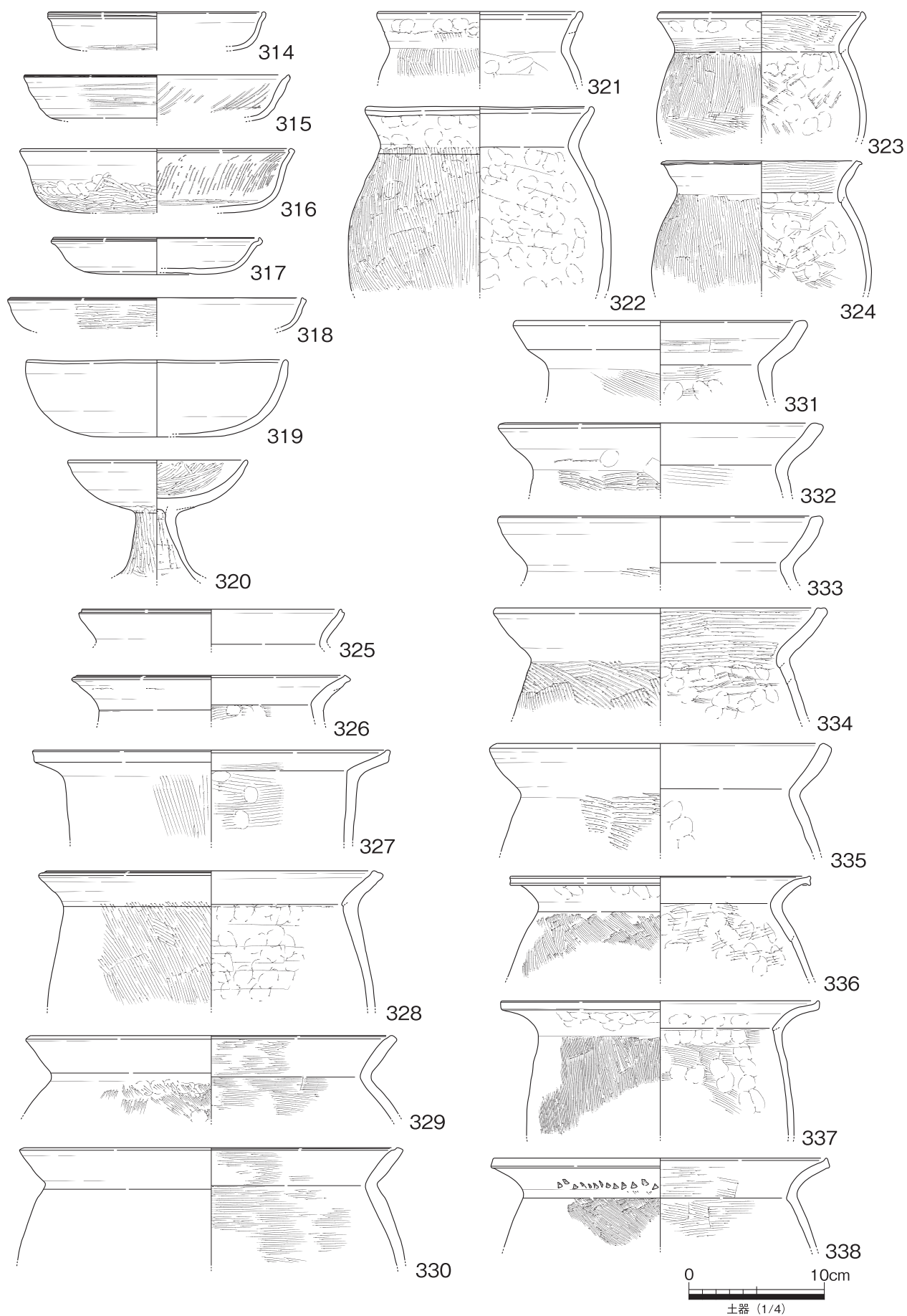
第92図 SD093 出土遺物実測図5
