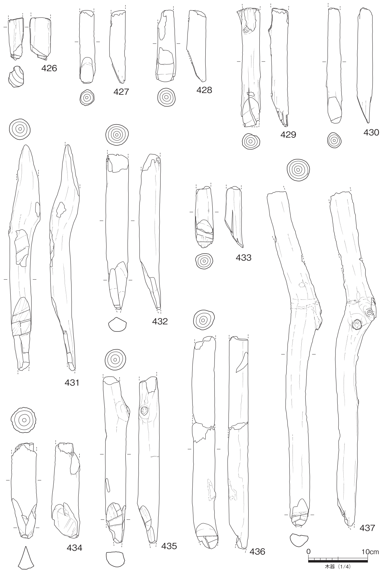
第99図 SD093 出土遺物実測図 12
