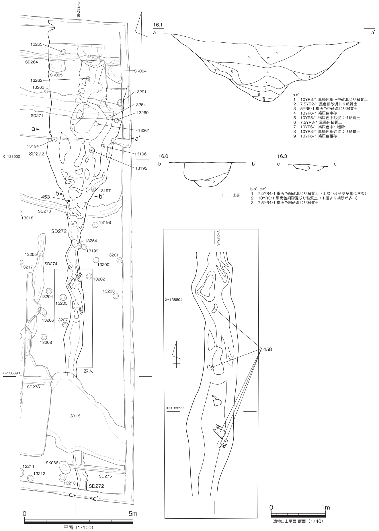
第102図 SD272平・断面図
